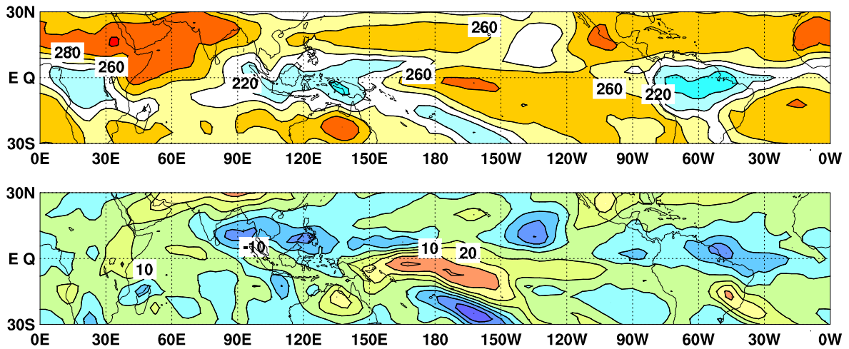
図9 外向き長波放射量 (OLR) (上) 及び平年偏差 (下) の分布図 (2022年3月)
