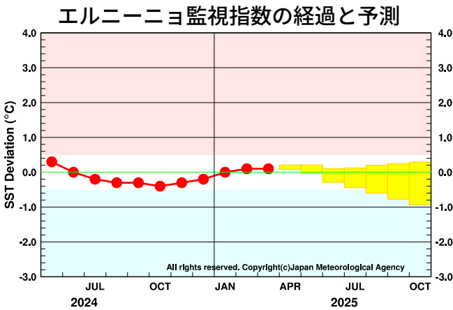
図 1 エルニーニョ監視海域の監視指数（海面水温の基準値との差）の 5 か月移動平均値の経過と予測 エルニーニョ監視海域の監視指数（海面水温の基準値との差）の 5 か月移動平均値について、3 月までの経過（観測値）を折れ線グラフで、大気海洋結合モデルによる予測結果（70%の確率で入ると予想される範囲）をボックスで示している。監視指数の 5 か月移動平均値が赤（+0.5℃以上）／青（-0.5℃以下）の範囲に入っている状態で 6 か月以上持続した場合に、エルニーニョ／ラニーニャ現象の発生としている。エルニーニョ監視海域の海面水温の基準値はその年の前年までの 30 年間の各月の平均値。
