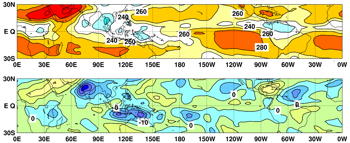
図 9 外向き長波放射量 (OLR) (上) 及び年間偏差 (下) の分布図 (2025 年 5 月)
