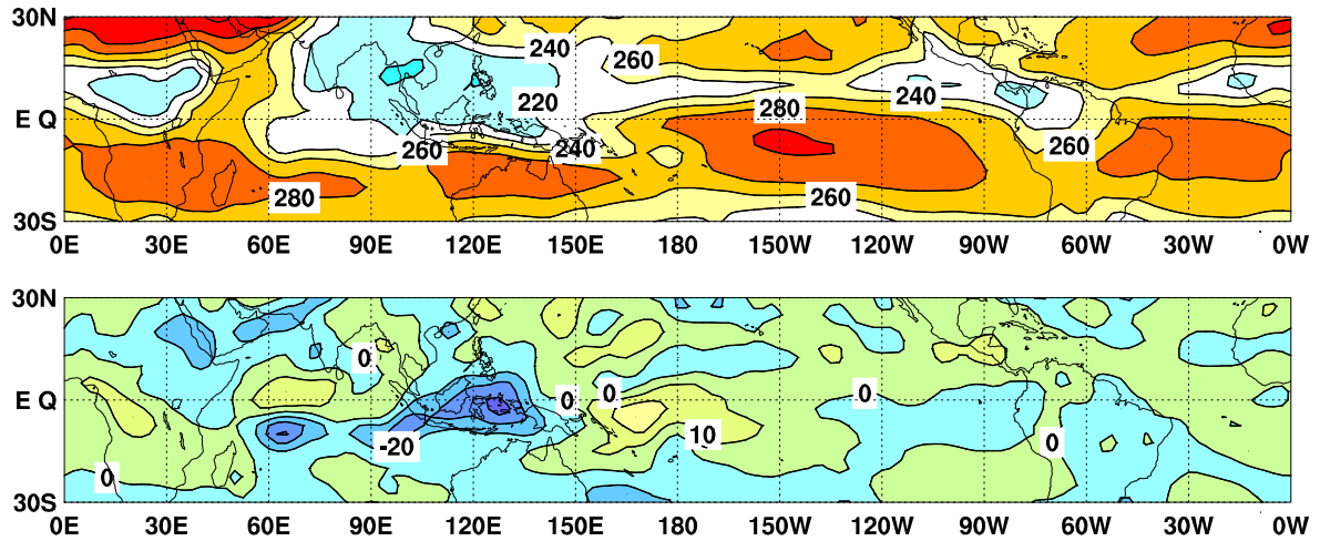
図 9 外向き長波放射量 (OLR) (上) 及び年偏差 (下) の分布図 (2025 年 8 月)
