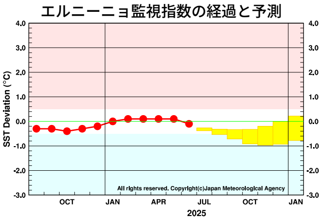
図 1 エルニーニョ監視海域の監視指数（海面水温の基準値との差）の 5 か月移動平均値の経過と予測 エルニーニョ監視海域の監視指数（海面水温の基準値との差）の 5 か月移動平均値について、6 月までの経過（観測値）を折れ線グラフで、大気海洋結合モデルによる予測結果（70%の確率で入ると予想される範囲）をボックスで示している。監視指数の 5 か月移動平均値が赤（+0.5°C 以上）／青（-0.5°C 以下）の範囲に入っている状態で 6 か月以上持続した場合に、エルニーニョ／ラニーニャ現象の発生としている。エルニーニョ監視海域の海面水温の基準値はその年の前年までの 30 年間の各月の平均値。
