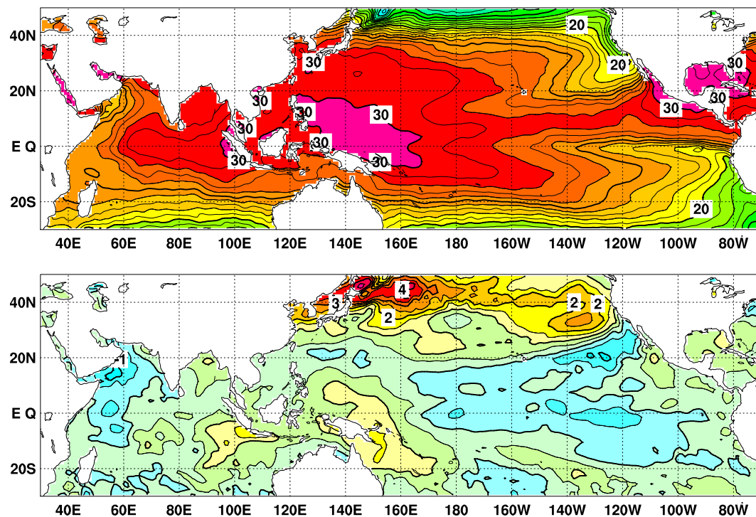
図4 2025年8月の海面水温図（上）及び平年偏差図（下）
