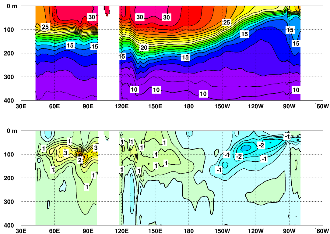
図5 2025年8月のインド洋から太平洋の赤道に沿った水温（上）及び平年偏差（下）の断面図
