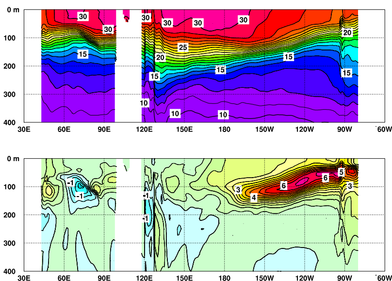
図 5 2026 年 6 月のインド洋から太平洋の赤道に沿った水温 (上) 及び平年偏差 (下) の断面図
