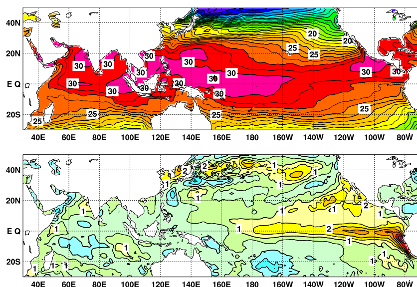
図 4 2026 年 6 月の海面水温図 (上) 及び平年偏差図 (下)
