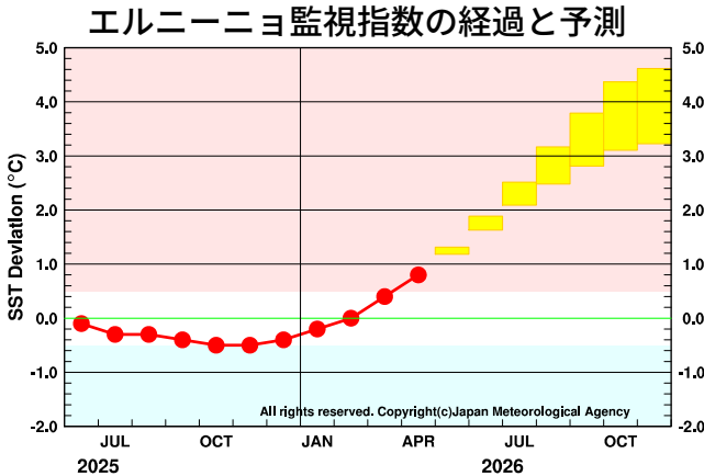
図 1 エルニーニョ監視海域の監視指数（海面水温の基準値との差）の 5 か月移動平均値の経過と予測 赤色（折れ線グラフ）はエルニーニョ監視海域の監視指数（海面水温の基準値との差）の 5 か月移動平均値の 4 月までの経過（観測値）、黄色のボックスは大気海洋結合モデルによる予測結果（70%の確率で入ると予想される範囲）を示す。ピンクの陰影は監視指数の 5 か月移動平均値が +0.5^{\circ}\text{C} 以上、水色の陰影は -0.5^{\circ}\text{C} 以下の範囲を示す。 監視指数は、エルニーニョ監視海域（北緯 5 度-南緯 5 度、西経 150 度-90 度）で平均した海面水温について、各月の値と基準値（その年の前年までの 30 年間の各月の平均値）の差を取ったもの。 気象庁では、監視指数の 5 か月移動平均値が赤（ +0.5^{\circ}\text{C} 以上）／青（ -0.5^{\circ}\text{C} 以下）の範囲に入っている状態で 6 か月以上持続した場合に、エルニーニョ／ラニーニャ現象の発生としている。
