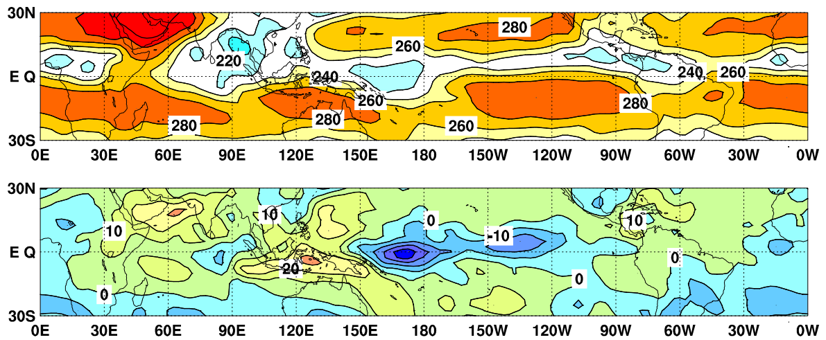
図 9 外向き長波放射量 (OLR) (上) 及び年間偏差 (下) の分布図 (2026 年 6 月)
