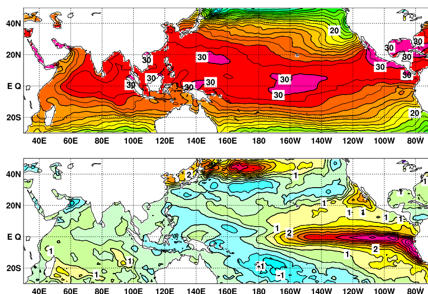
図 4 2026 年 8 月の海面水温図 (上) 及び平年偏差図 (下)
