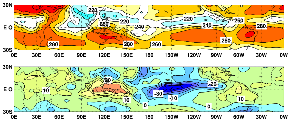
図 9 外向き長波放射量 (OLR) (上) 及び年間偏差 (下) の分布図 (2026 年 8 月)
