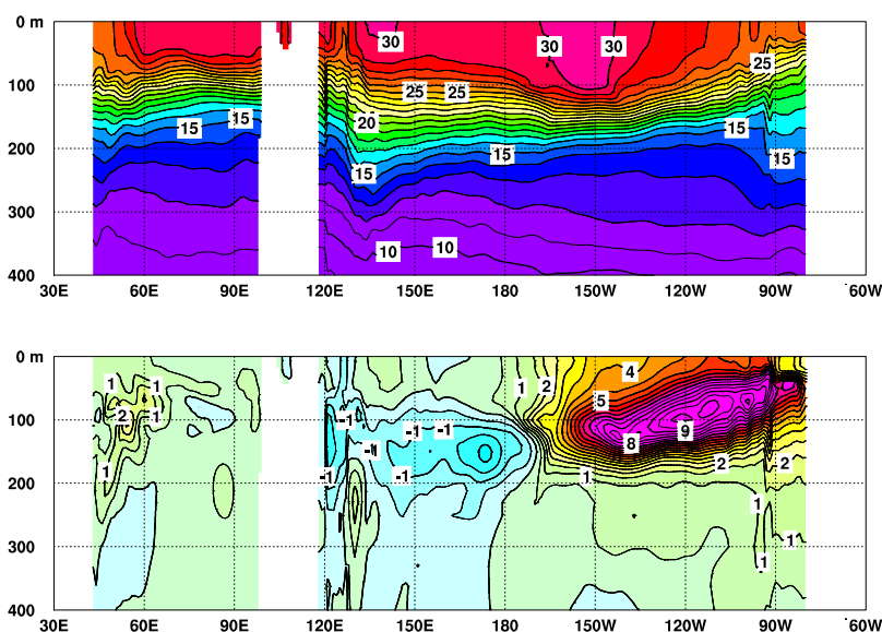
図 5 2026 年 8 月のインド洋から太平洋の赤道に沿った水温 (上) 及び平年偏差 (下) の断面図
