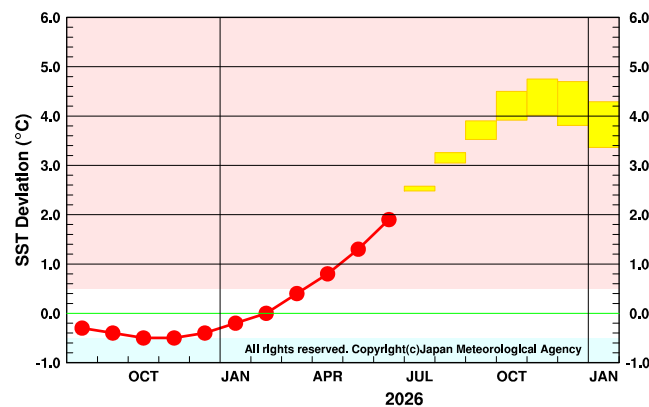
図 1 エルニーニョ監視海域の監視指数（海面水温の基準値との差）の 5 か月移動平均値の経過と予測 赤い折れ線グラフはエルニーニョ監視海域の監視指数（観測値）の 5 か月移動平均値の経過、黄色のボックスは大気海洋結合モデルによる監視指数の予測結果（70%の確率で入ると予想される範囲）を示す。ピンクの部分は監視指数の 5 か月移動平均値が +0.5℃ 以上、水色の部分は -0.5℃ 以下の範囲を示す。
