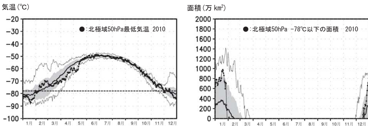
図II 4-1：北半球高緯度下部成層圏の最低気温(左)および気温が -78^{\circ}\text{C} 以下の領域の面積(右)の年変化(2010年)
