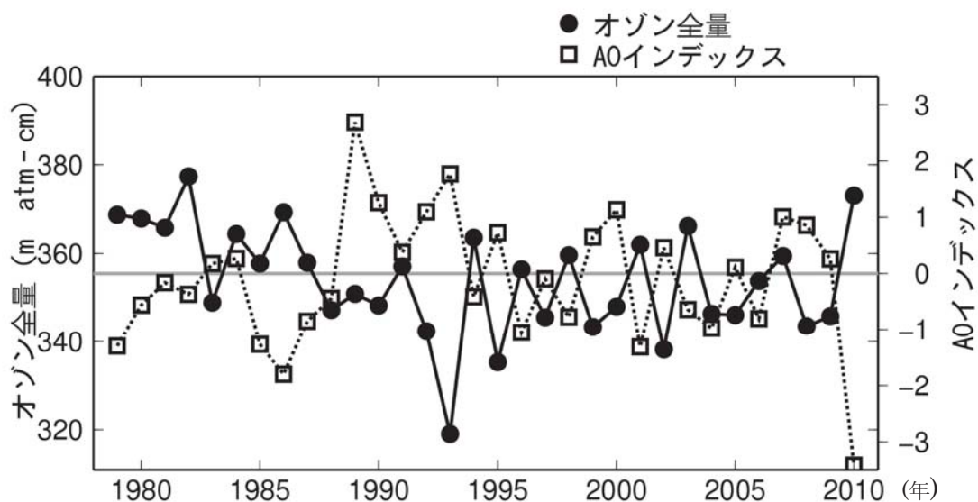
図E9-2：AOインデックスと中緯度のオゾン全量の推移(1979～2010年)
