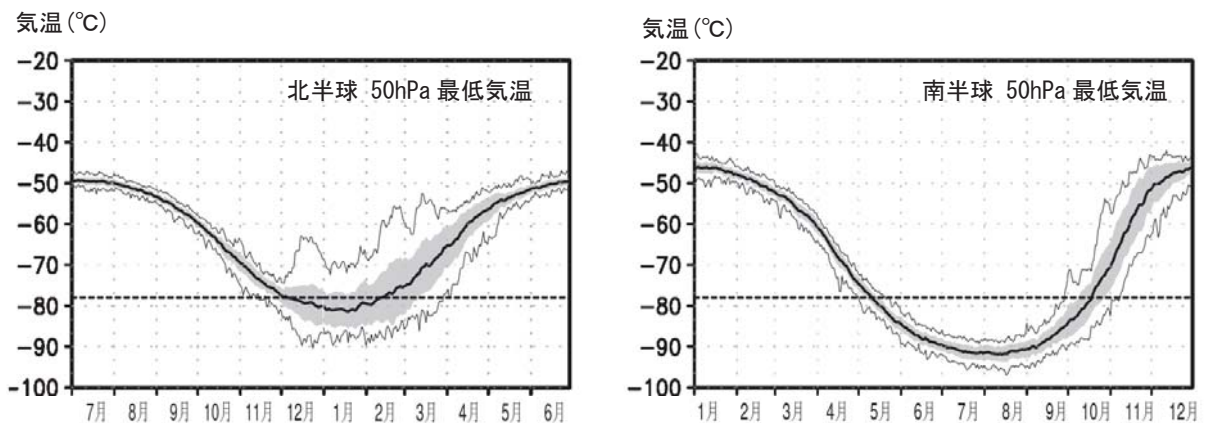
図E8-1：北半球と南半球50hPa面における高緯度域の最低気温の年変化
