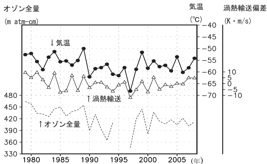
図E9-1：3月の北半球高緯度下部成層圏気温とオゾン全量の経年変化(2008年まで)
