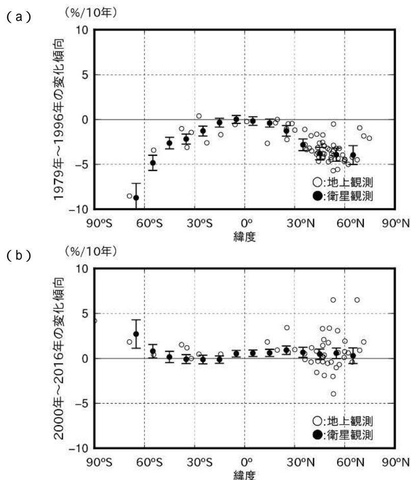
図2-2：オゾン全量の長期変化傾向の緯度帯別分布
