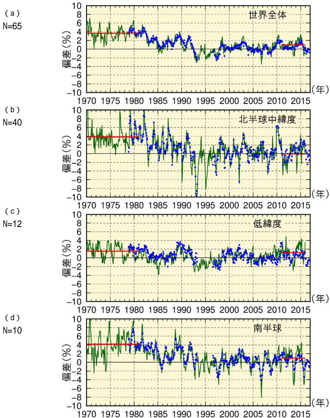
図2-1：世界のオゾン全量偏差 (%) の長期変化
