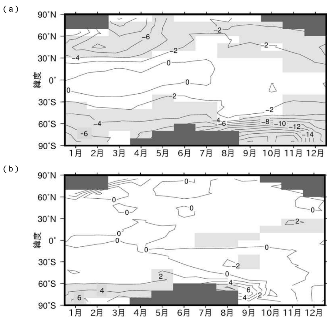
図2-3：オゾン全量の季節変化の緯度別長期変化傾向
