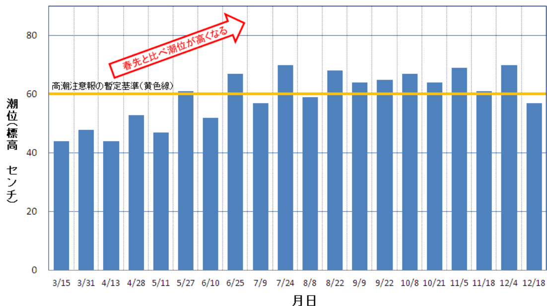
図 1-1 大潮の時期の最高潮位 (大船渡 (岩手県))
