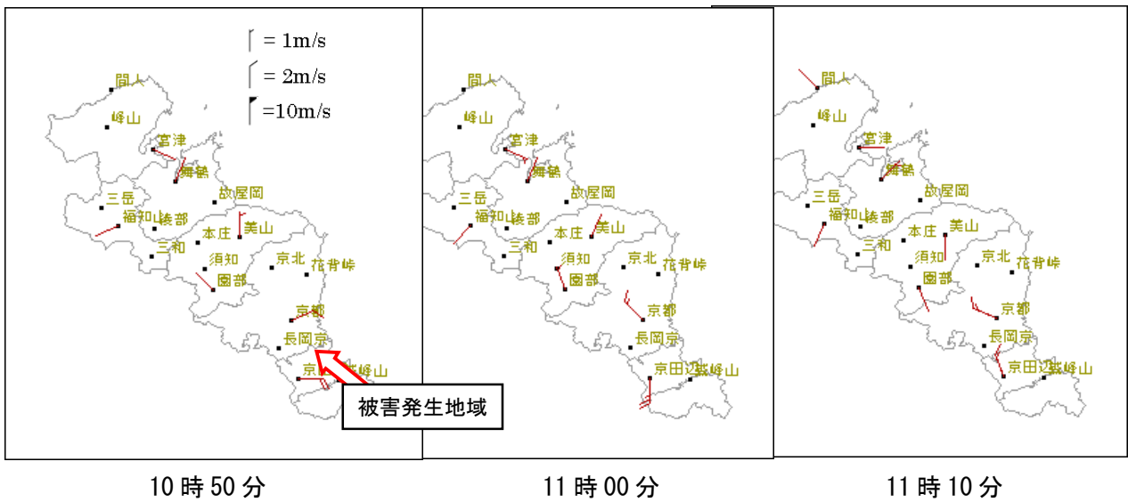
図 6 アメダス地点における風向風速分布図 (8 月 1 日)
