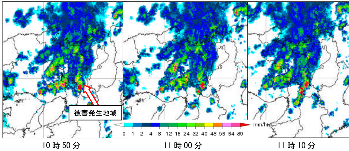
図 7 気象レーダー画像 (8 月 1 日)
