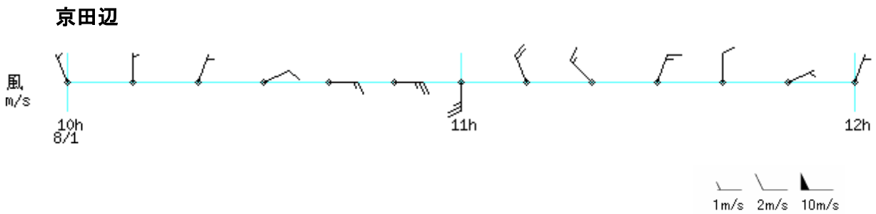
図 8 アメダス風向・風速時系列グラフ (8 月 1 日 10 時 ~ 12 時)
