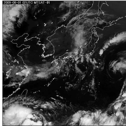
図 5 気象衛星赤外面像 (8 月 1 日 11 時)
