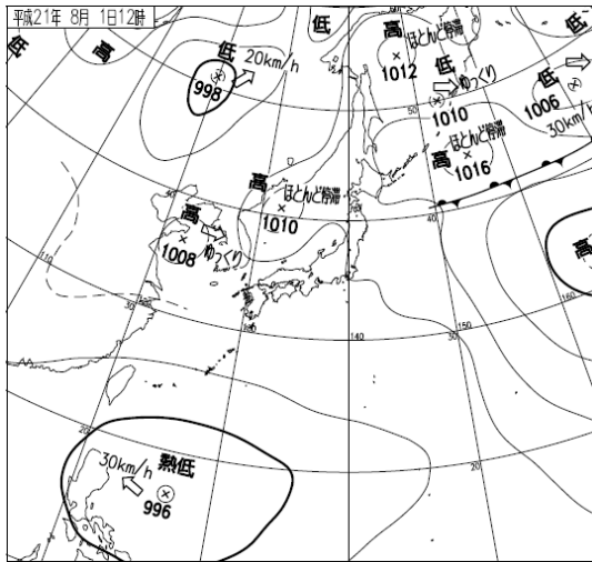
図 4 地上天気図 (8 月 1 日 12 時)
