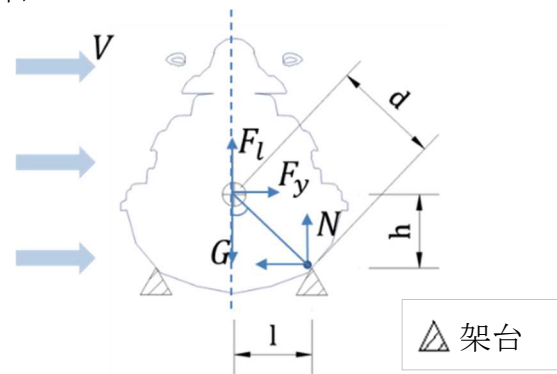
風速算定 (架台のスパンは 2l とする)
