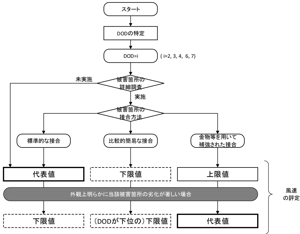
図 DOD=2,3,4,6,7 の風速の評定フロー ((3)②の手順は省略している)
