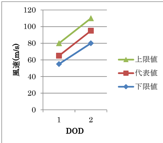
200<AA×CC の電柱の場合
