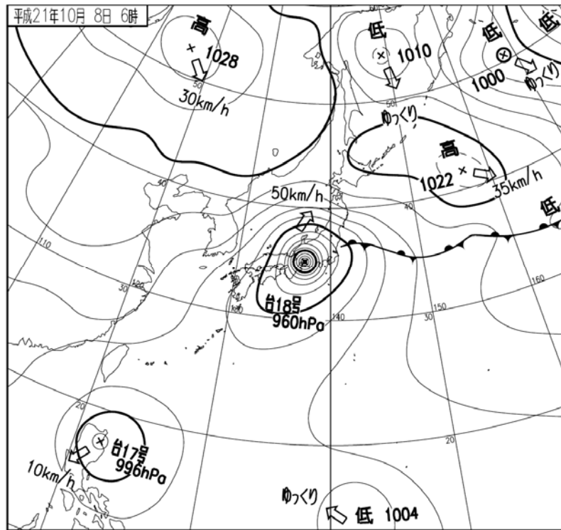
地上天気図 平成 21 年 10 月 8 日 06 時 (日本時間)
