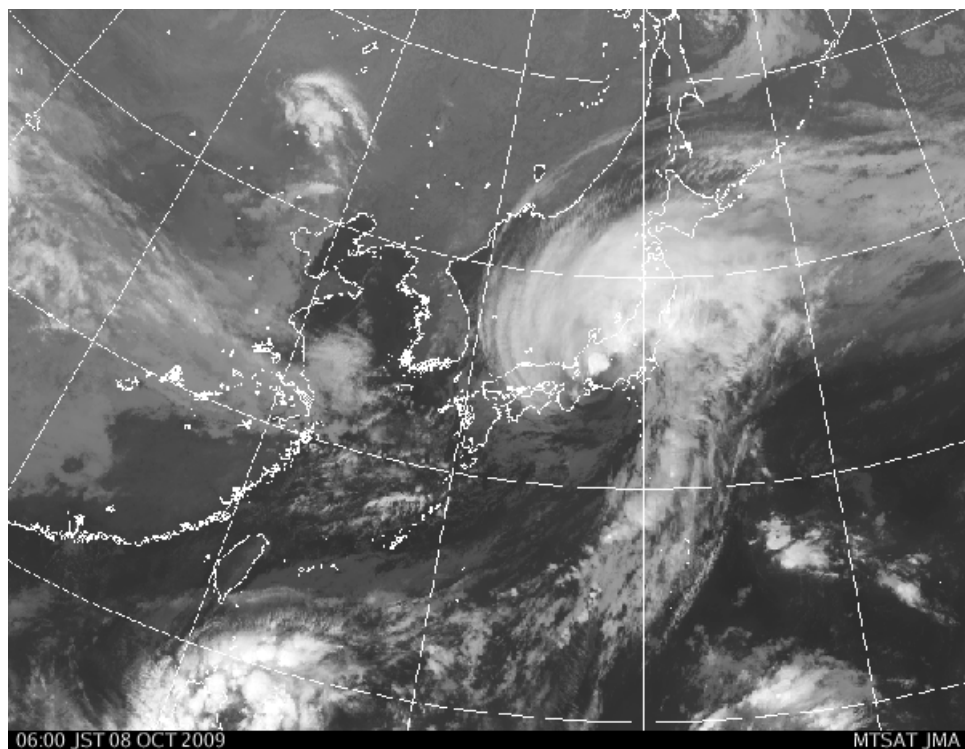
衛星画像(赤外) 平成 21 年 10 月 8 日 06 時 (日本時間)
