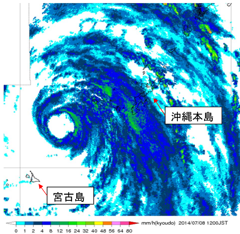
気象レーダー (降水強度) 2014年7月8日12時
