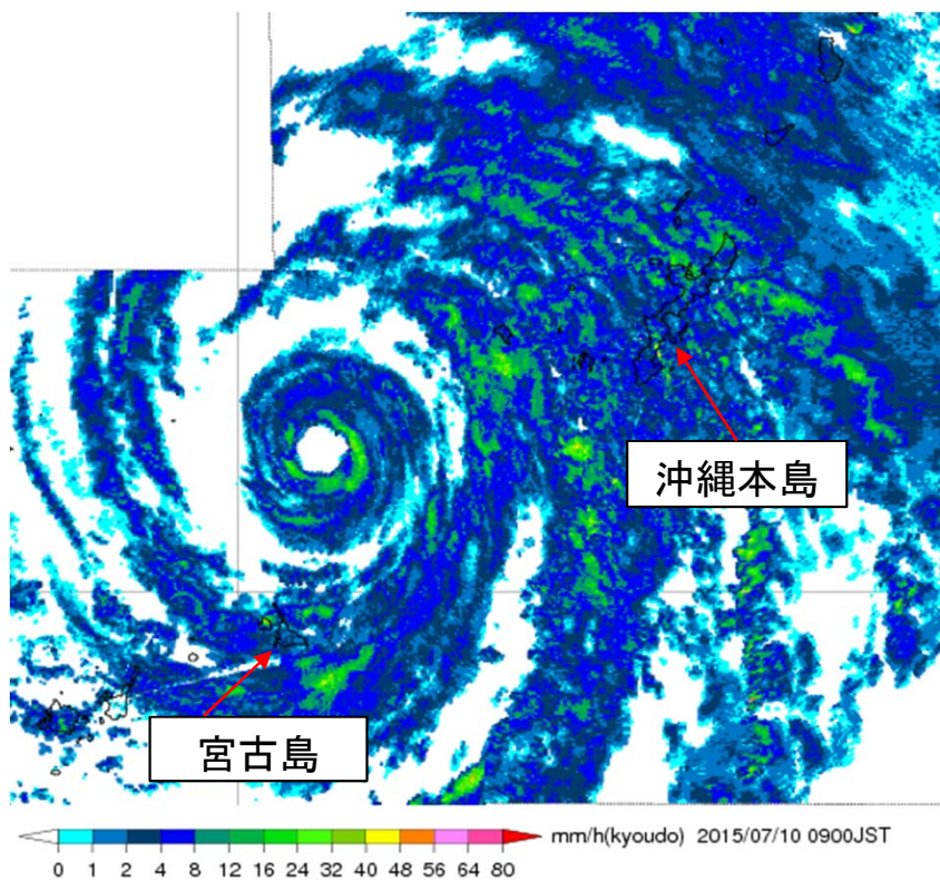
気象レーダー（降水強度）2015年7月10日09時
