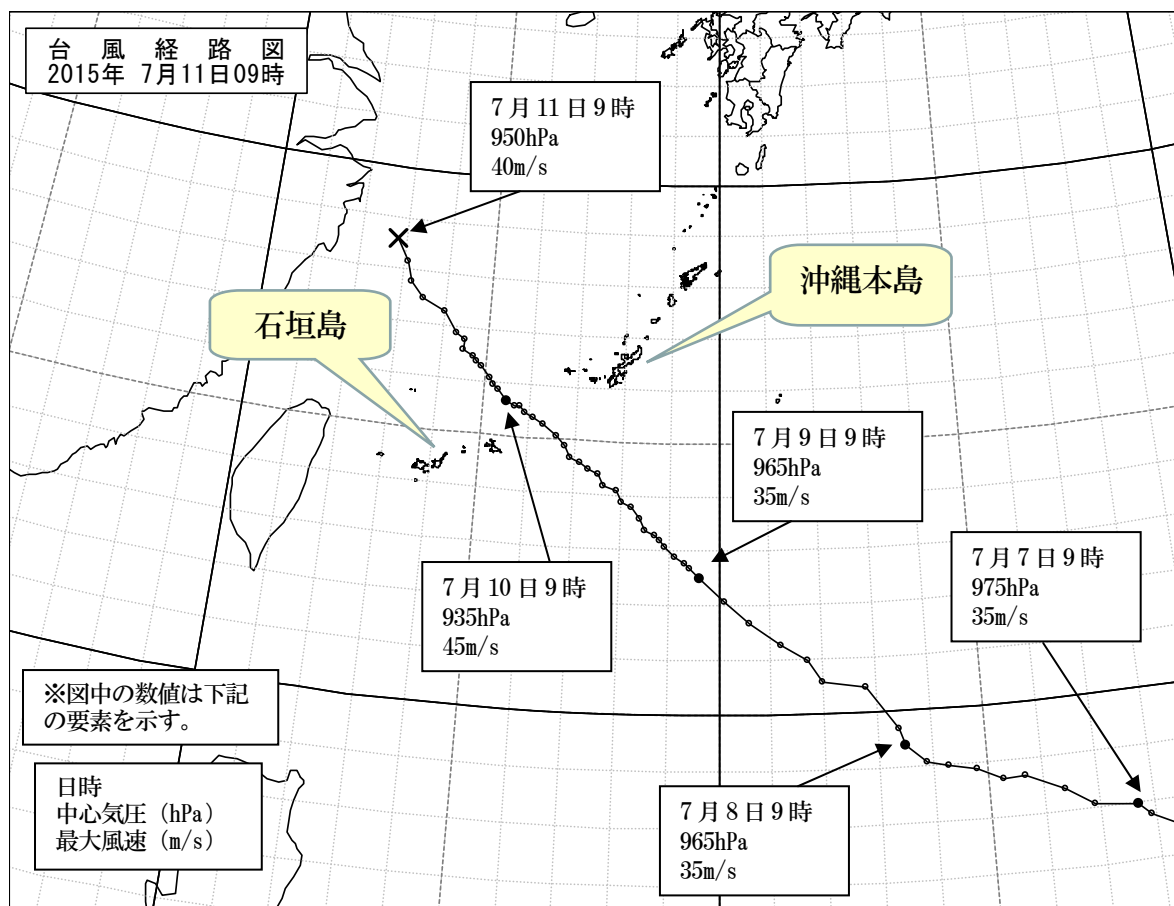
台風第9号経路図（2015年7月11日09時現在 速報値）
