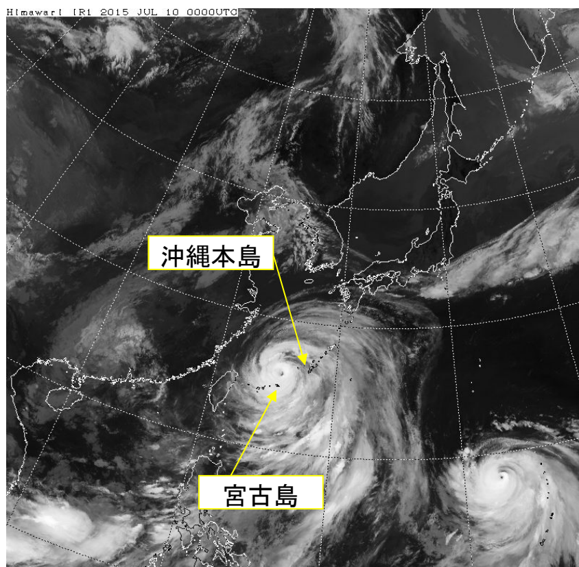
気象衛星画像（赤外）2015年7月10日09時
