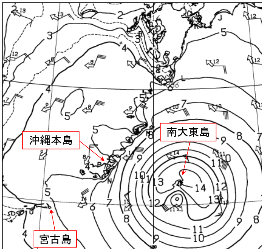
沿岸波浪実況図 2020年9月5日21時
