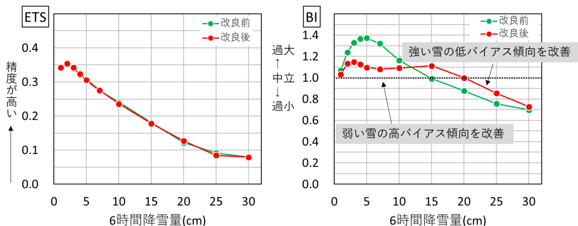
第5図 6時間降雪量予測値のアメダス観測値に対する（左）エクイタブルスコア（ETS）と（右）バイアススコア（BI）。
