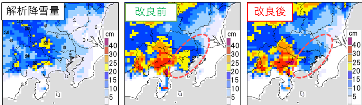
第4図 令和6年2月5日22時（日本時間）までの6時間降雪量。（左）解析降雪量、（中）改良前の降雪短時間予報、（右）改良後の降雪短時間予報。（左）解析降雪量は本改良を適用したものであり、数字はアメダスの観測値による。
