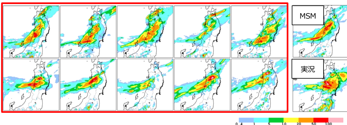
第1図 MEPSによる前6時間積算降水量(mm/6h)の予測例(赤枠内)。平成29年07月22
