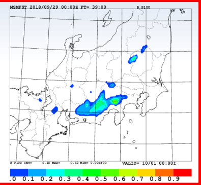
MEPS100mm/3h以上の確率 東海地方での確率を表現。
