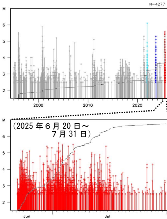
図2-3 領域a内のM-T図及び回数積算図
