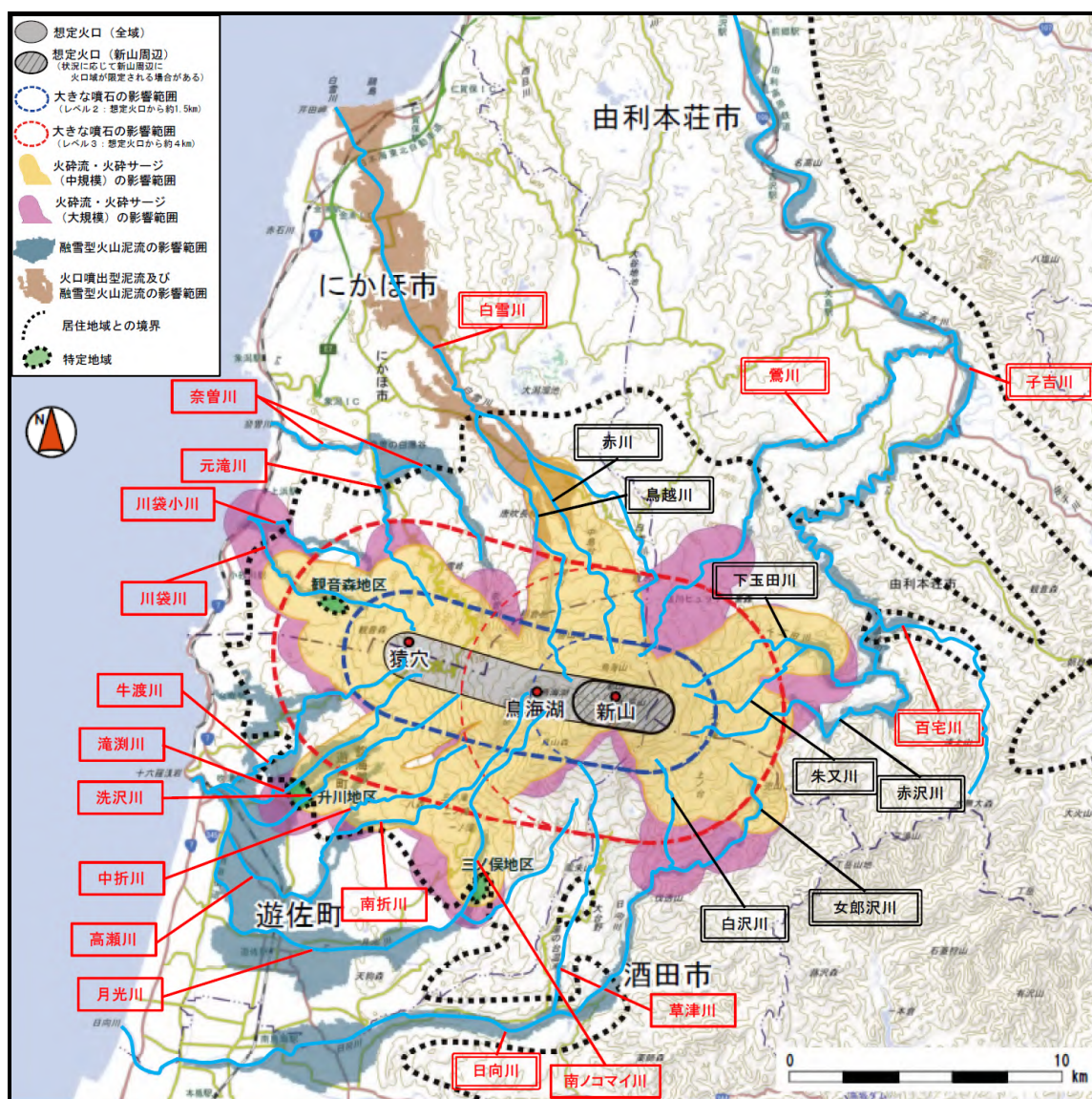
図2 噴火に伴う現象及び警戒が必要な範囲（想定火口が全域の場合）
