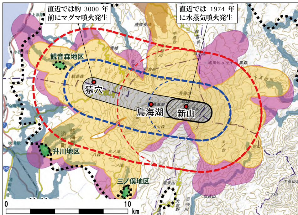
図1 鳥海山の想定火口域と想定される噴石飛散範囲
