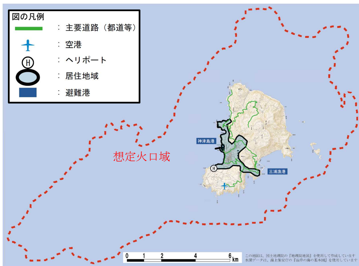
図1 想定火口域
