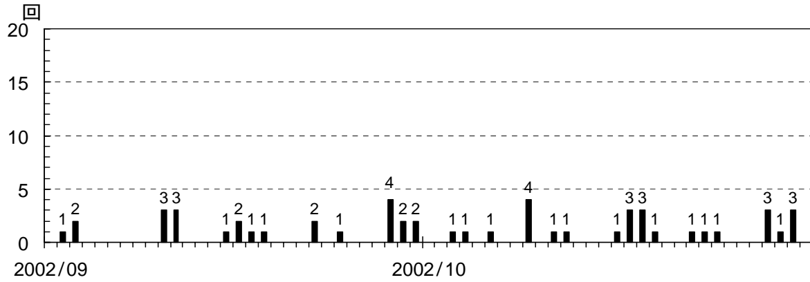
図3 A型地震の発生回数(2002年9月1日~10月31日)
