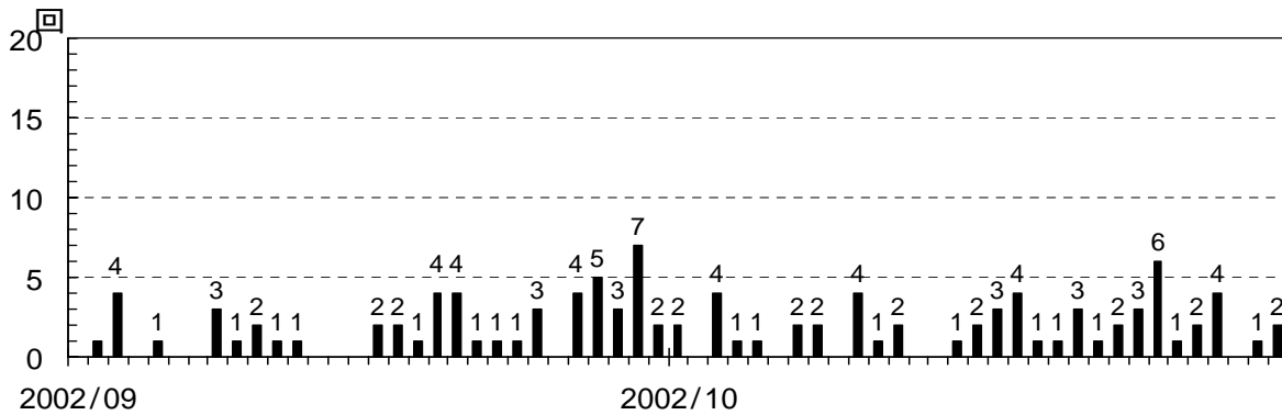
図5 B型地震の発生回数(2002年9月1日~10月31日)
