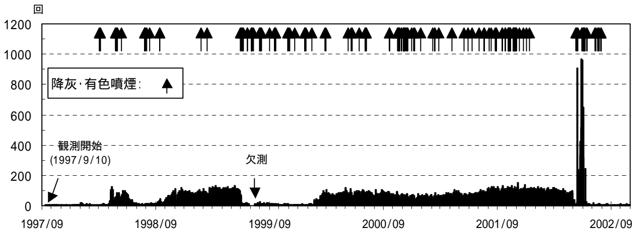
図 2 地震発生回数(1997 年 9 月 ~ 2002 年 10 月)
