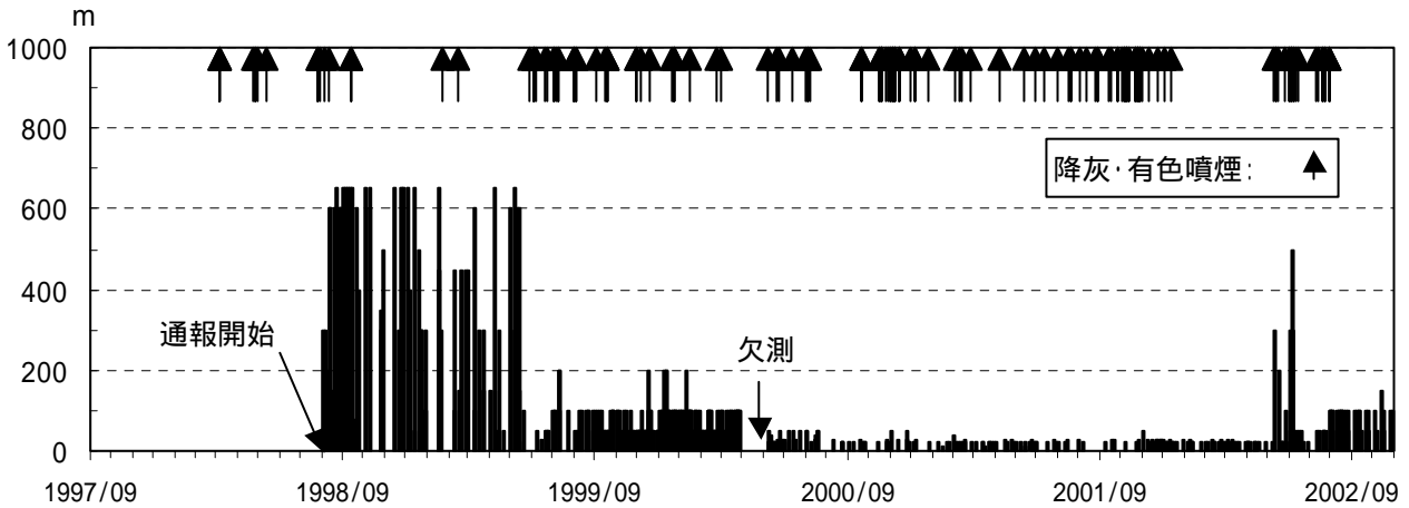
図 1 噴煙の日最高高度(1998 年 8 月 ~ 2002 年 10 月 : 三島村役場硫黄島出張所による)
