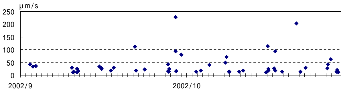
図4 A型地震の最大振幅 (U-D成分)(2002年9月1日~10月31日)
