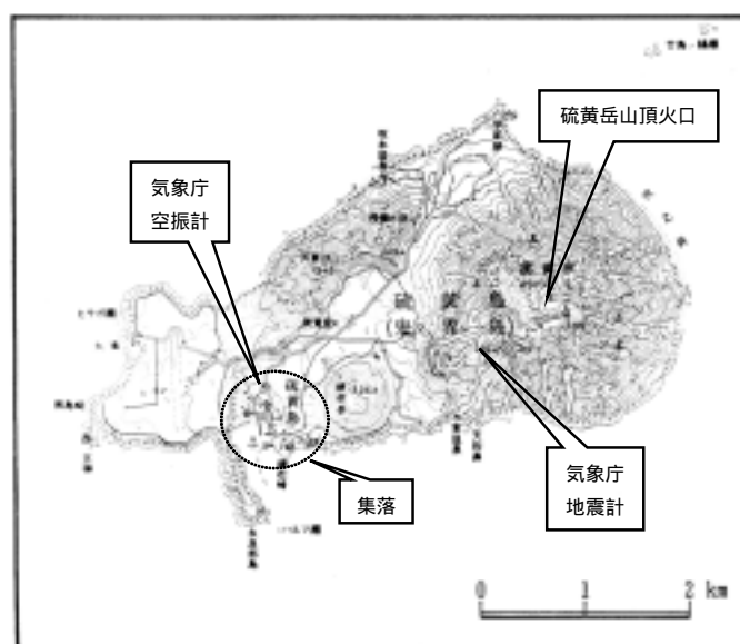
図8 観測点位置図
