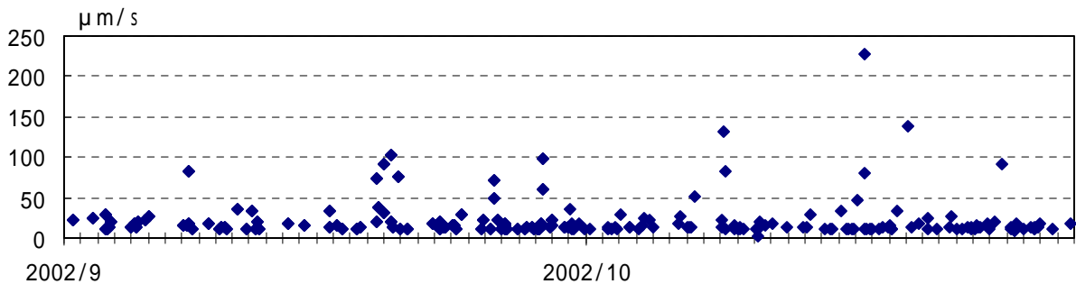
図6 B型地震の最大振幅 (U-D成分)(2002年9月1日~10月31日)
