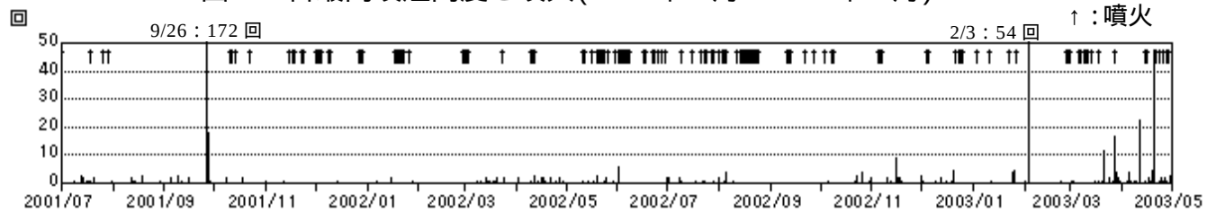
図 2 A 型地震の日別回数(2001 年 7 月～2003 年 4 月)
