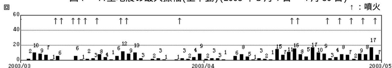
図8 B型地震の日別発生回数(2003年3月1日～4月30日)
