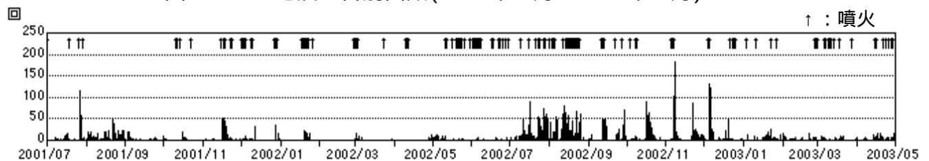
図 3 B 型地震の日別回数(2001 年 7 月～2003 年 4 月)
