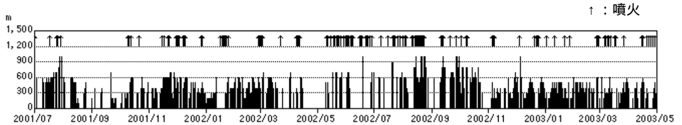
図 1 日最高噴煙高度と噴火(2001 年 7 月～2003 年 4 月)
