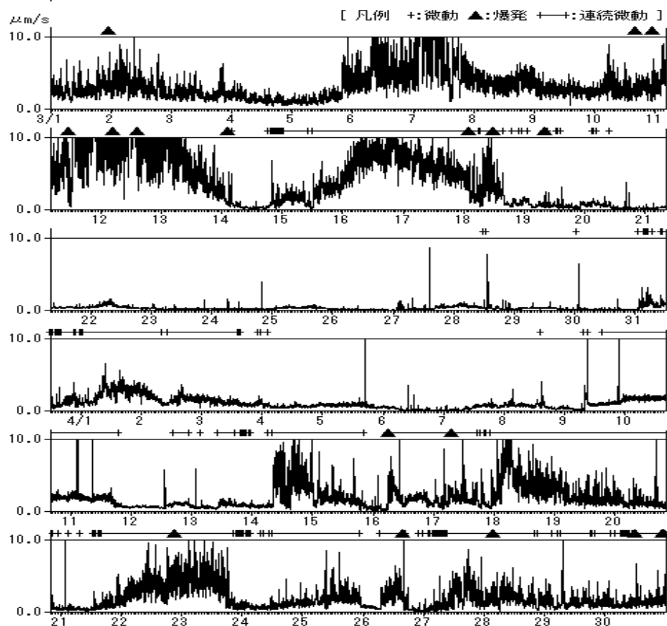
図 4 1 分間平均振幅の時間変化(上下動)(2003 年 3 月 1 日～4 月 30 日)
