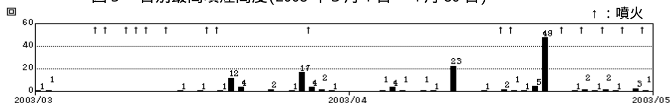
図6 A型地震の日別回数(2003年3月1日～4月30日)
