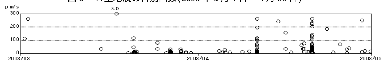
図7 A型地震の最大振幅(上下動)(2003年3月1日～4月30日)
