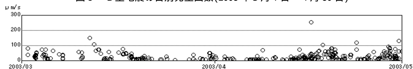
図9 B型地震の最大振幅(上下動)(2003年3月1日～4月30日)
