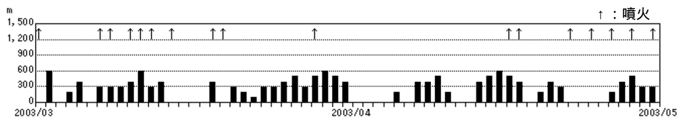
図5 日別最高噴煙高度(2003年3月1日～4月30日)
