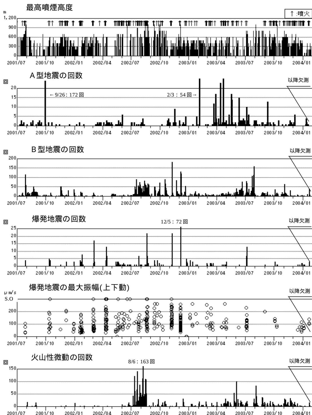
図2 火山活動経過図(2001年7月～2004年1月)
