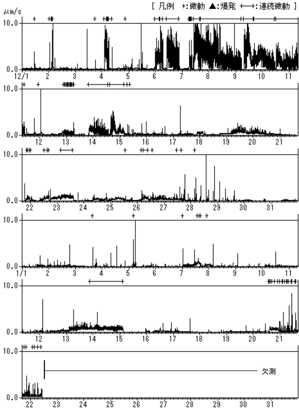
図4 地震計(上下動)の1分間平均振幅の変化(2003年12月1日～1月31日) 2004年1月22日から機器故障のため欠測しています。
