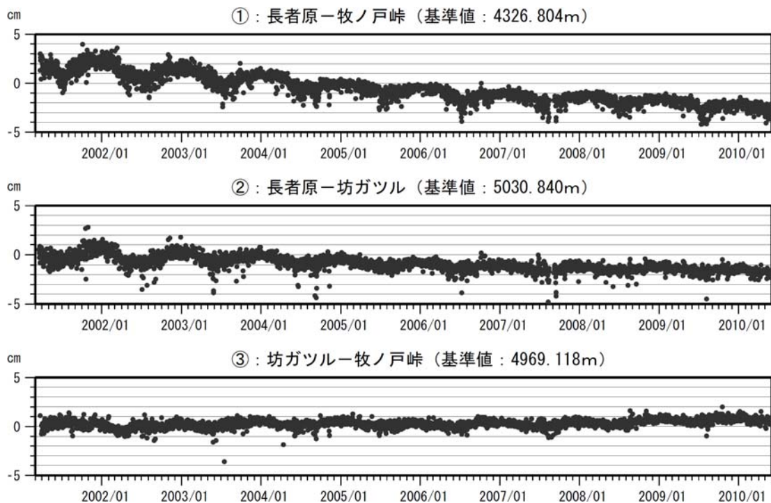
図 3 九重山 GPS 連続観測による基線長変化（2001 年 3 月～2010 年 5 月）
