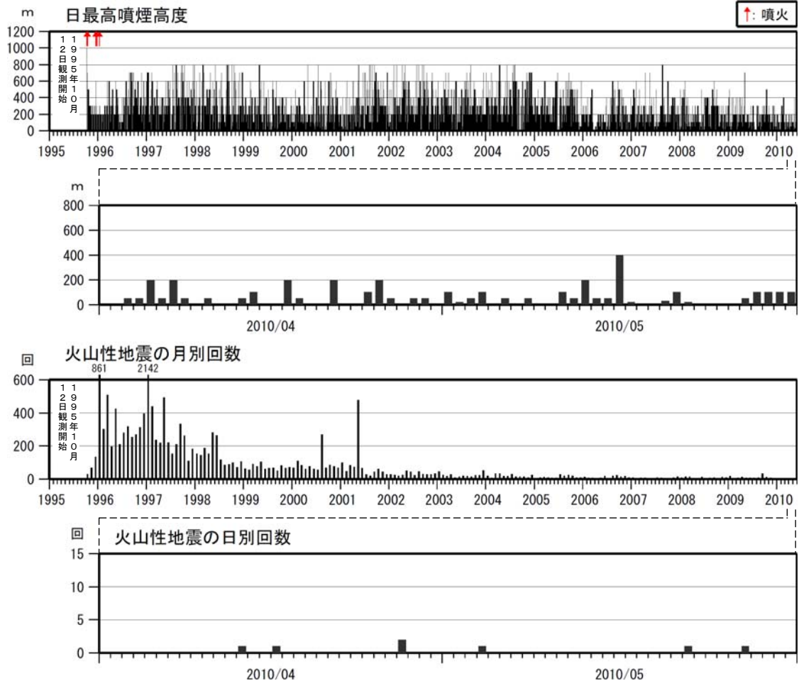
図 2 九重山 火山活動経過図（1995 年 10 月～2010 年 5 月）
