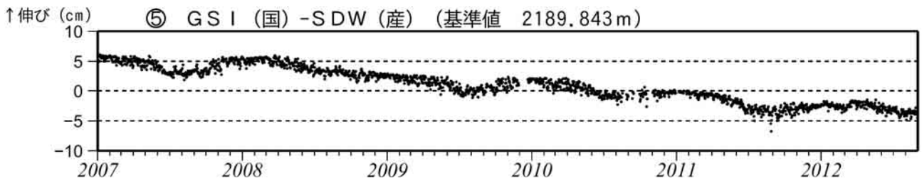
図 3※ 口永良部島 GPS 連続観測による基線長変化（2007 年 1 月～2012 年 8 月） GPS 連続観測では、火山活動によると思われる変化は認められませんでした。
