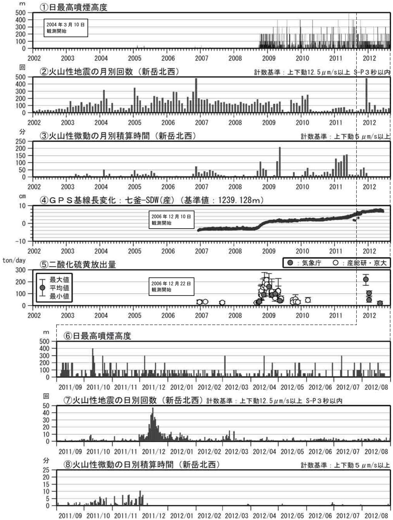
図2 口永良部島 火山活動経過図（2002年1月～2012年8月）
