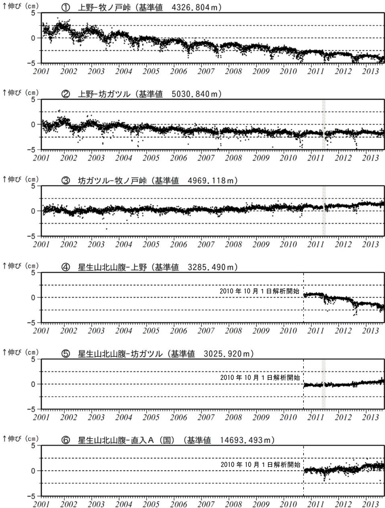
図3 九重山 GPS 連続観測による基線長変化 (2001年3月～2013年8月) 火山活動によると考えられる変化は認められませんでした。
