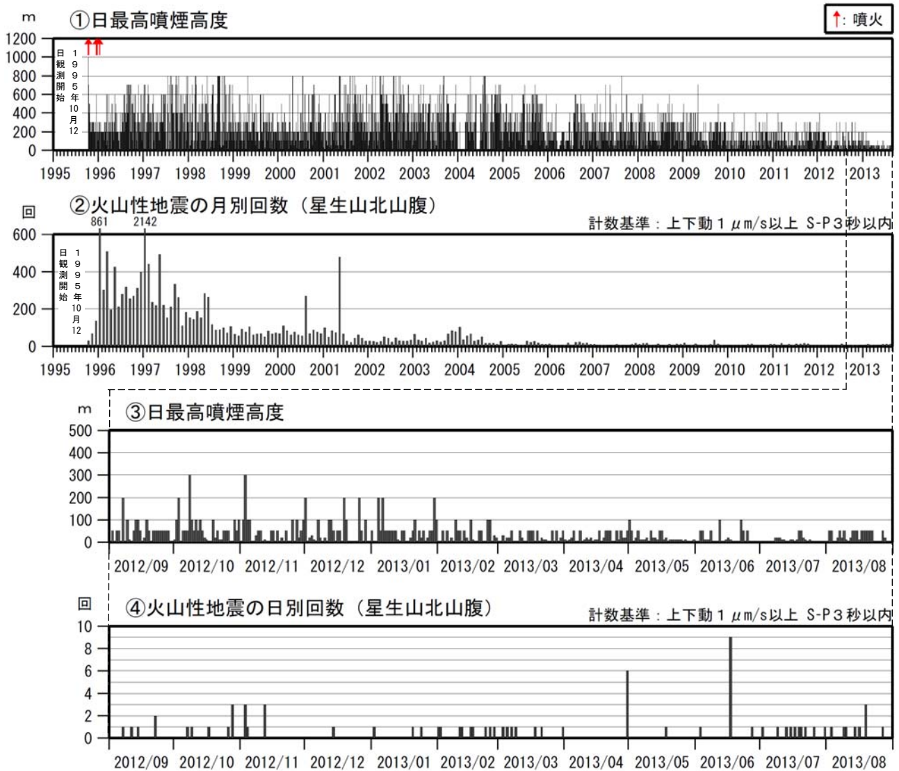
図 2 九重山 火山活動経過図（1995 年 10 月～2013 年 8 月）
