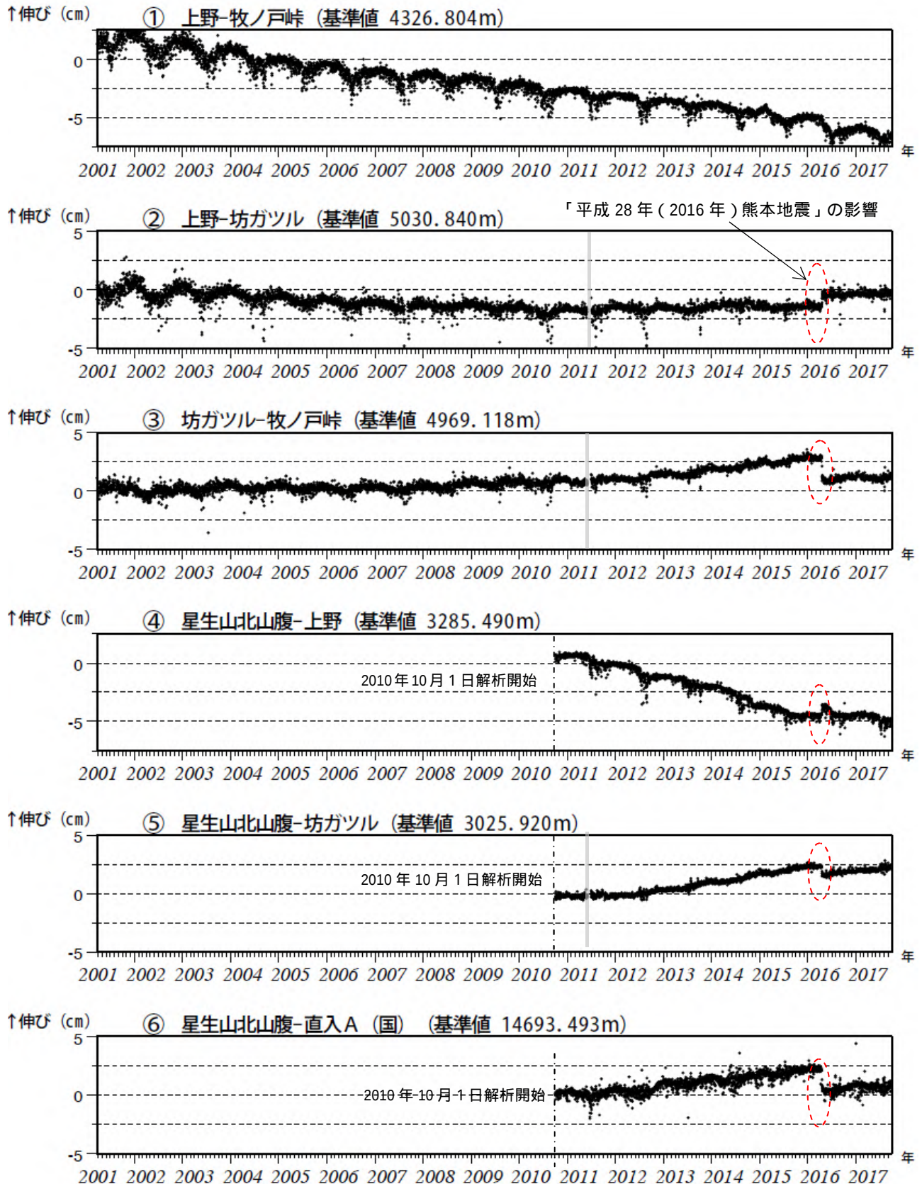
図 6 九重山 GNSS 連続観測による基線長変化 (2001 年 3 月～2017 年 9 月)
