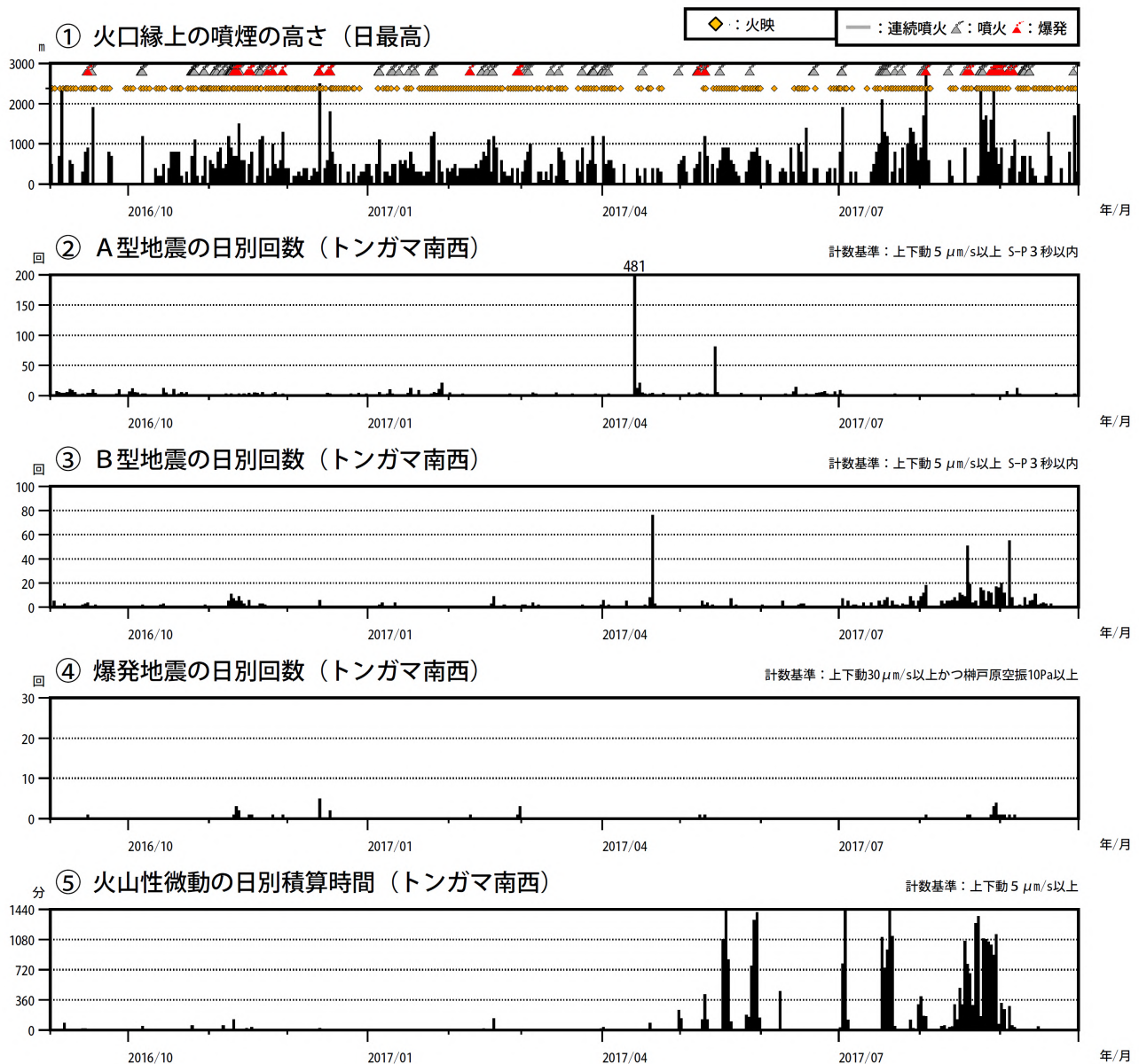
図 3 諏訪之瀬島 最近の火山活動経過図（2016 年 9 月～2017 年 9 月）
