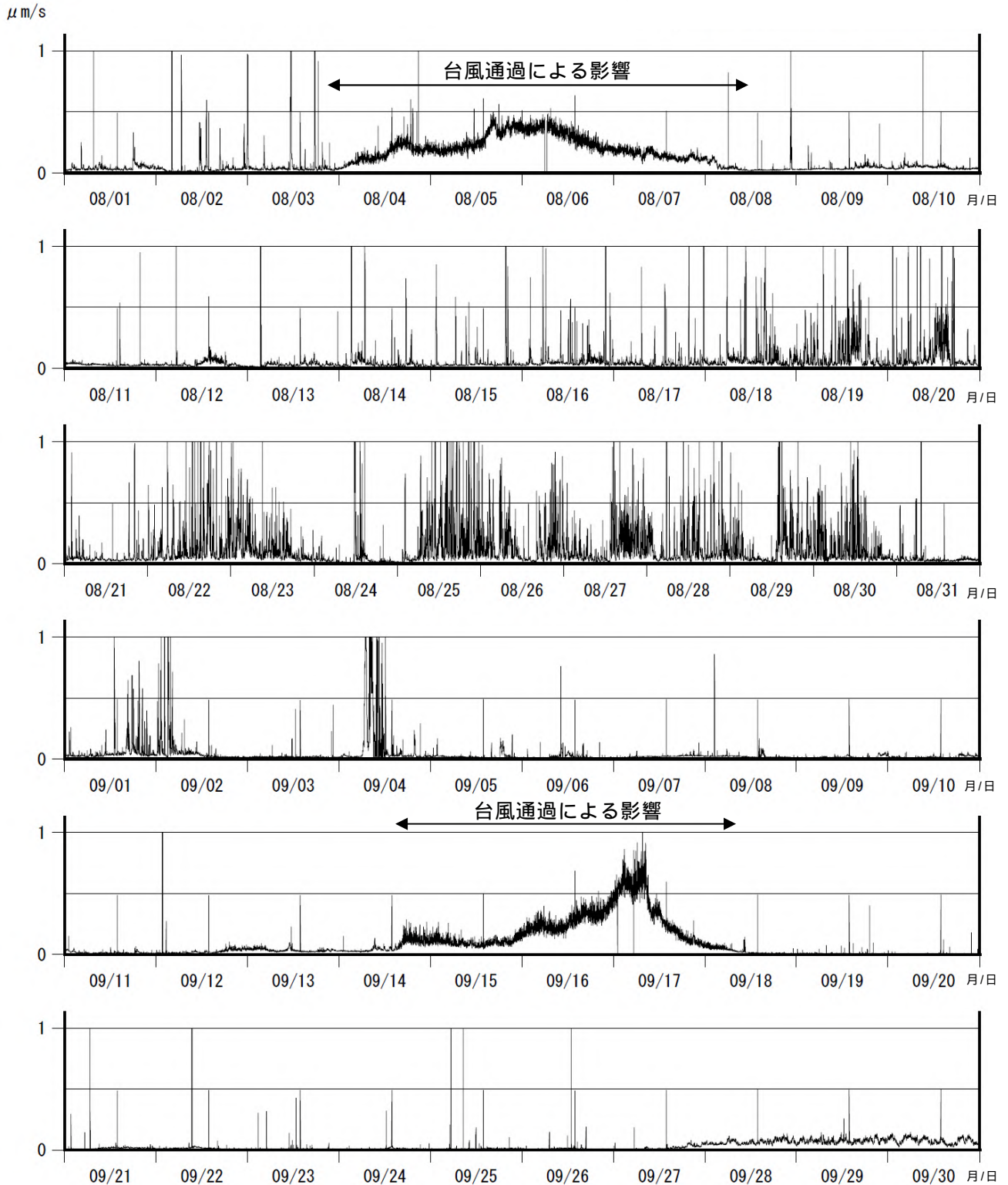
図4 諏訪之瀬島 1分間平均振幅の時間変化（ナベタオ観測点上下動成分、2017年8月～9月）
