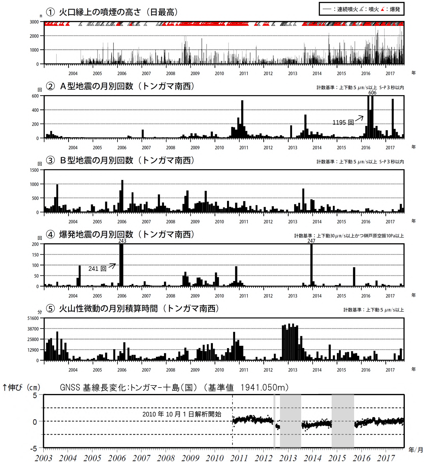
図 2 諏訪之瀬島 長期の火山活動経過図（2003 年 1 月～2017 年 9 月）
