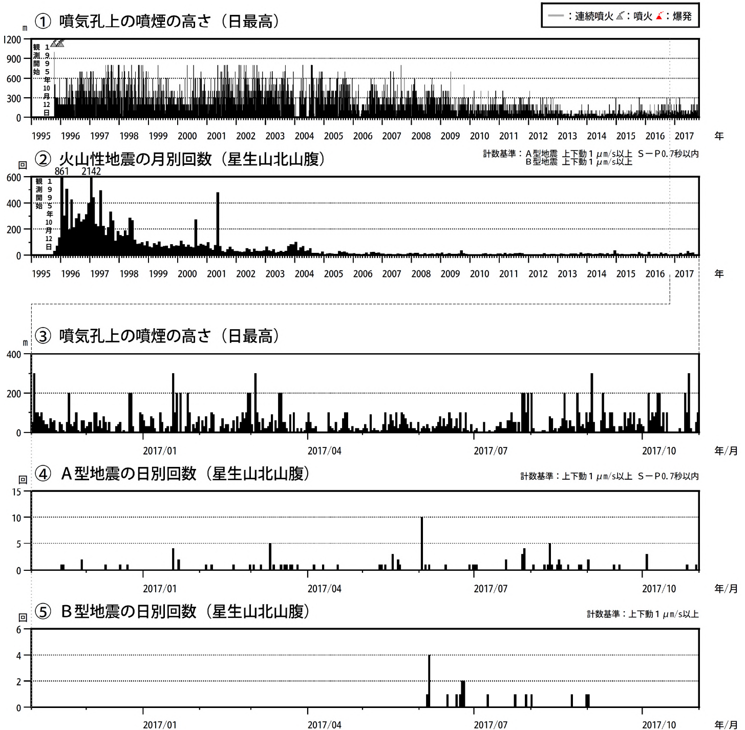
図3 九重山 火山活動経過図（1995 年 10 月～2017 年 10 月）
