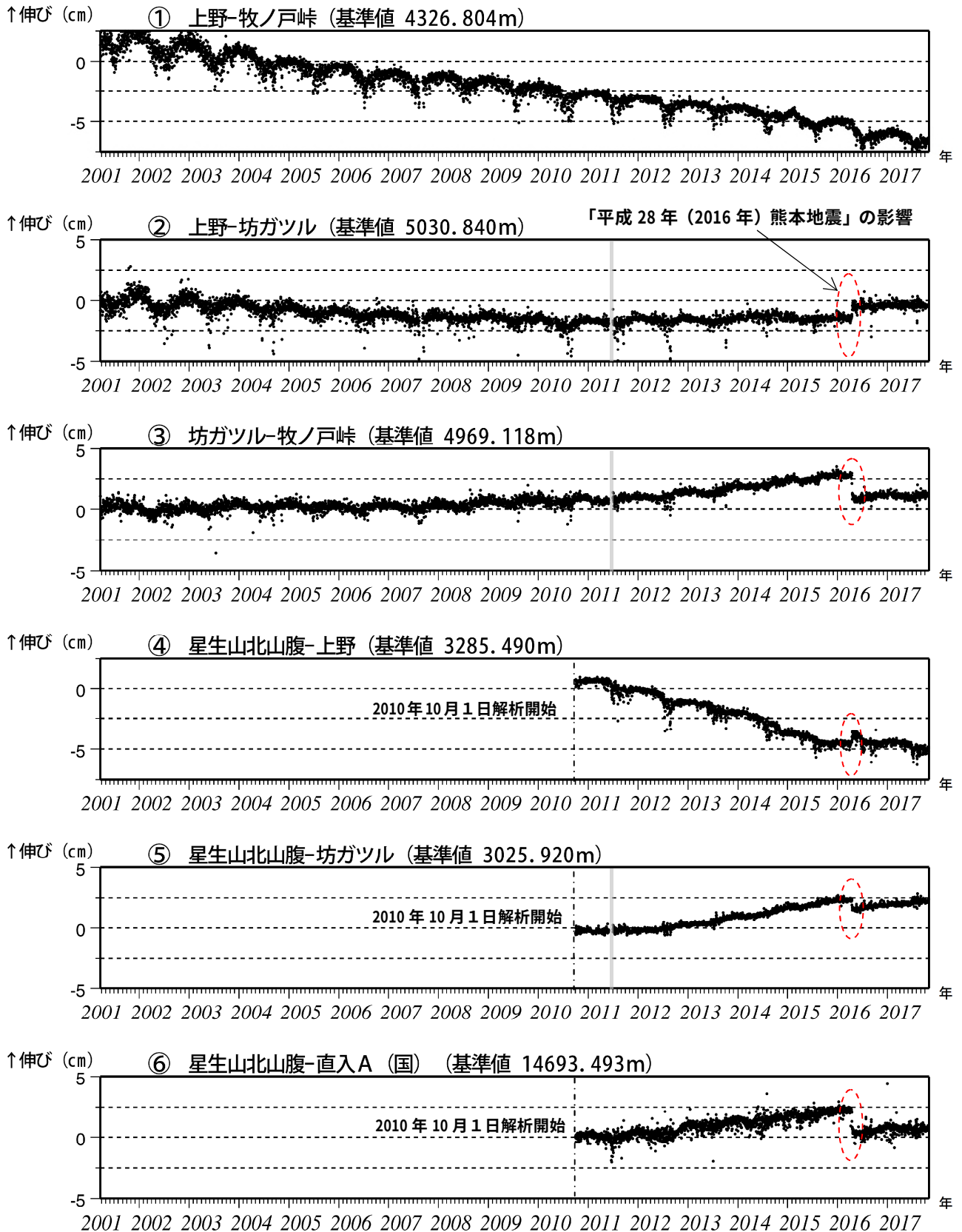
図 4 九重山 GNSS 連続観測による基線長変化 (2001 年 3 月～2017 年 10 月)
