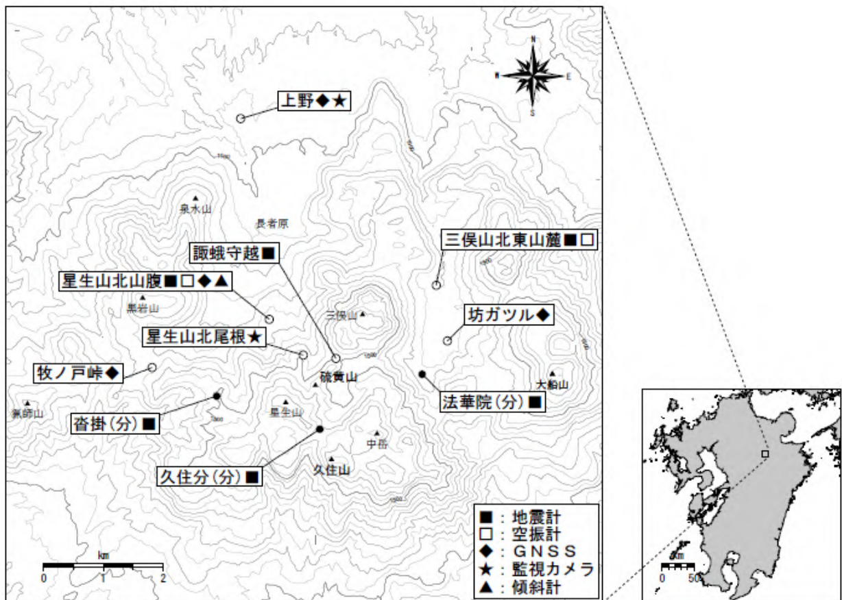
図 6 九重山 観測点配置図
