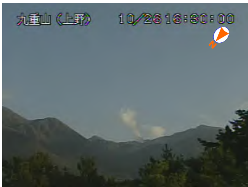
図1 九重山 噴煙の状況（10月26日、上野監視カメラによる）
