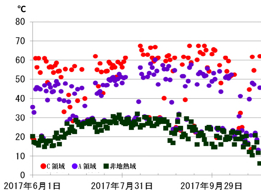
図2 九重山 赤外熱映像装置による日別最高温度（2017年6月1日～10月31日） （星生山北尾根監視カメラによる）
