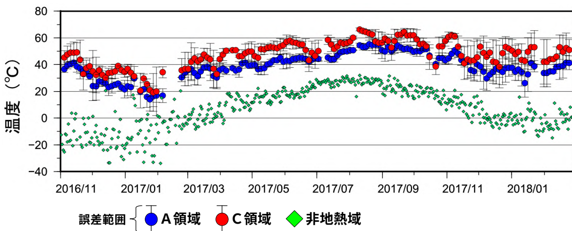
図 2-2 九重山 星生山北尾根赤外熱映像装置による日別最高温度の 7 日間移動平均値 （2016 年 11 月～2018 年 2 月）
