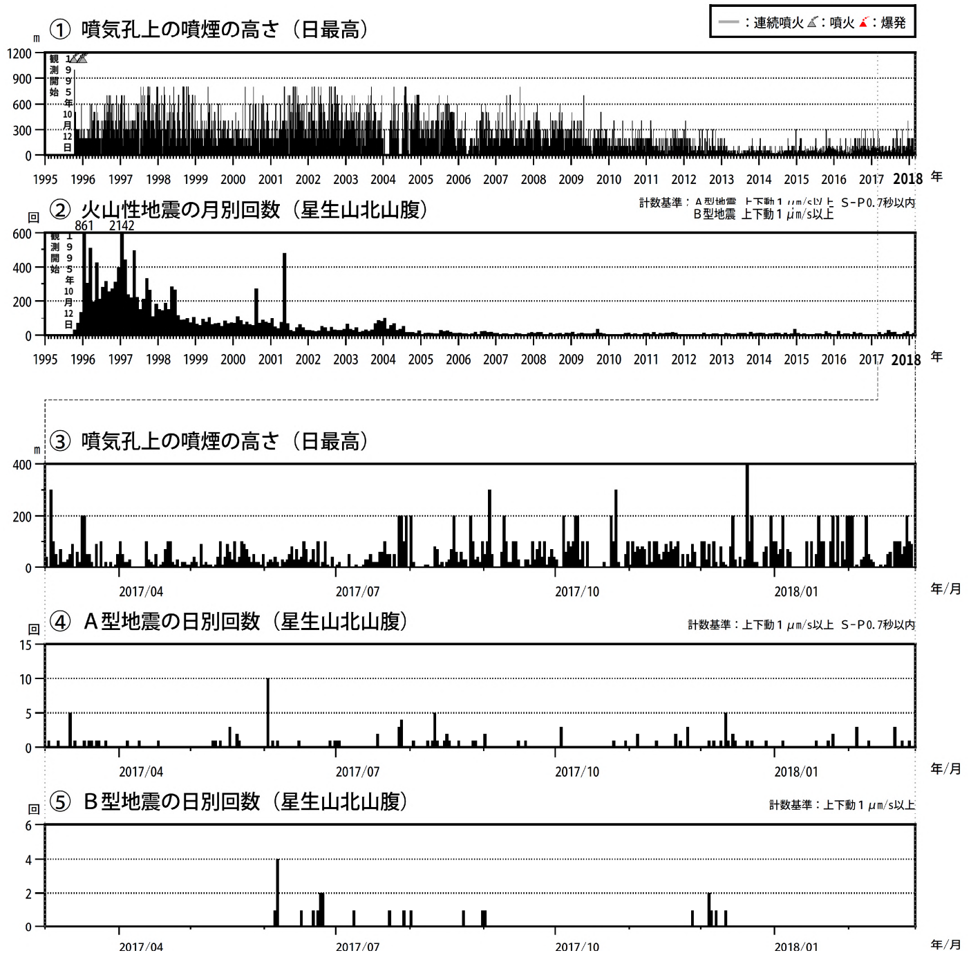
図3 九重山 火山活動経過図（1995 年 10 月～2018 年 2 月）
