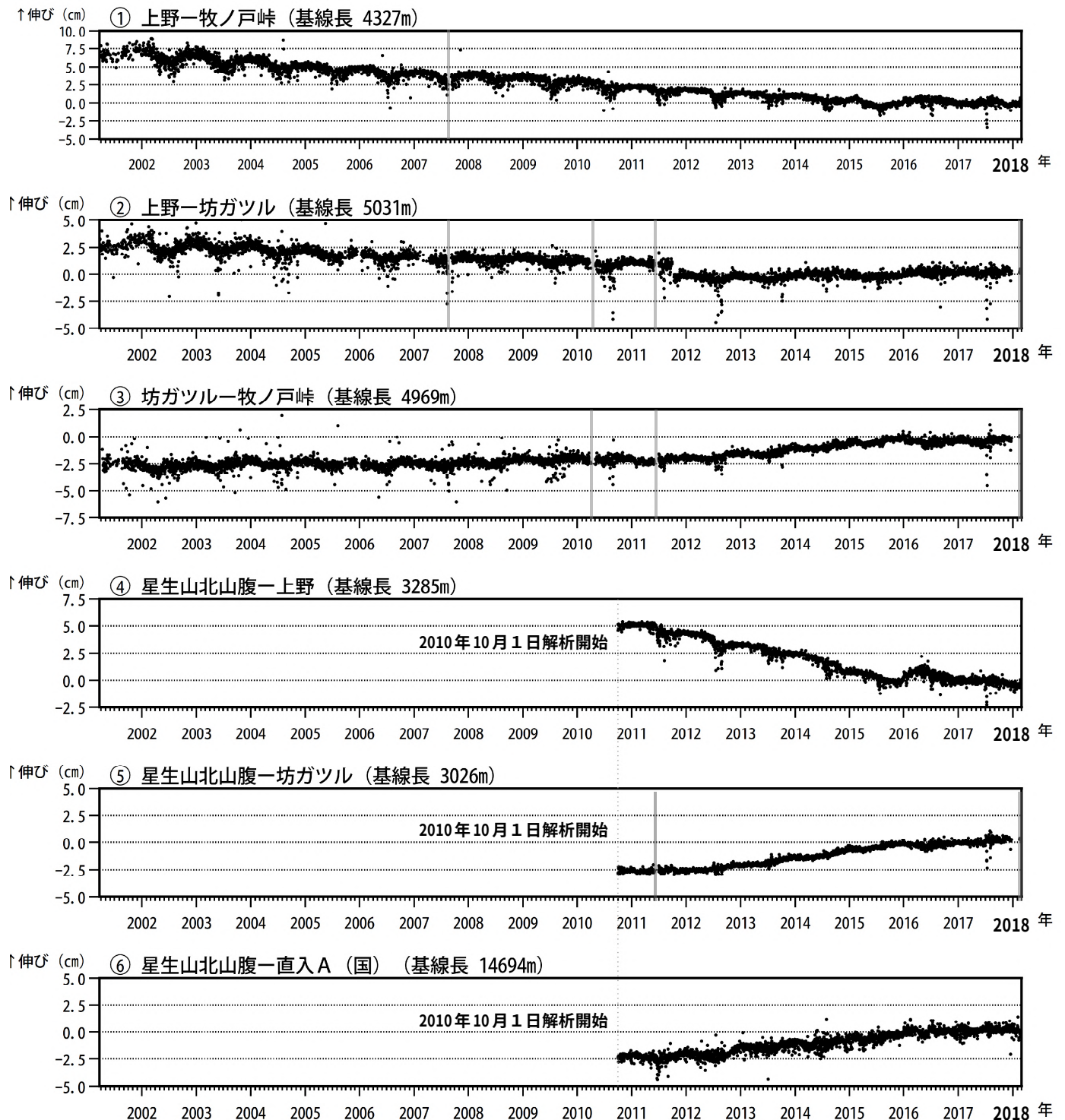
図5 九重山 GNSS 連続観測による基線長変化 (2001 年 3 月～2018 年 2 月)
