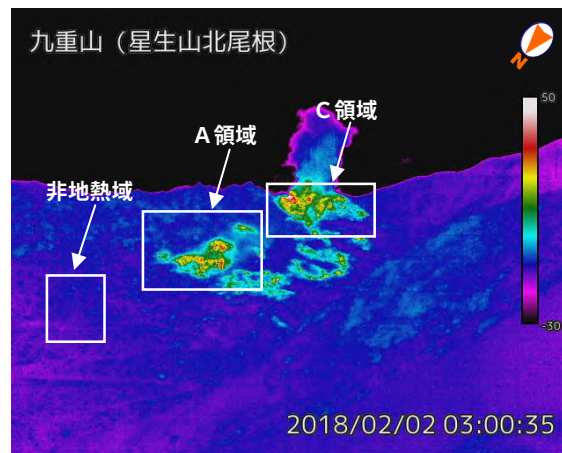
図 2-1 九重山 地熱域の状況（2月2日、星生山北尾根赤外熱映像装置による）
