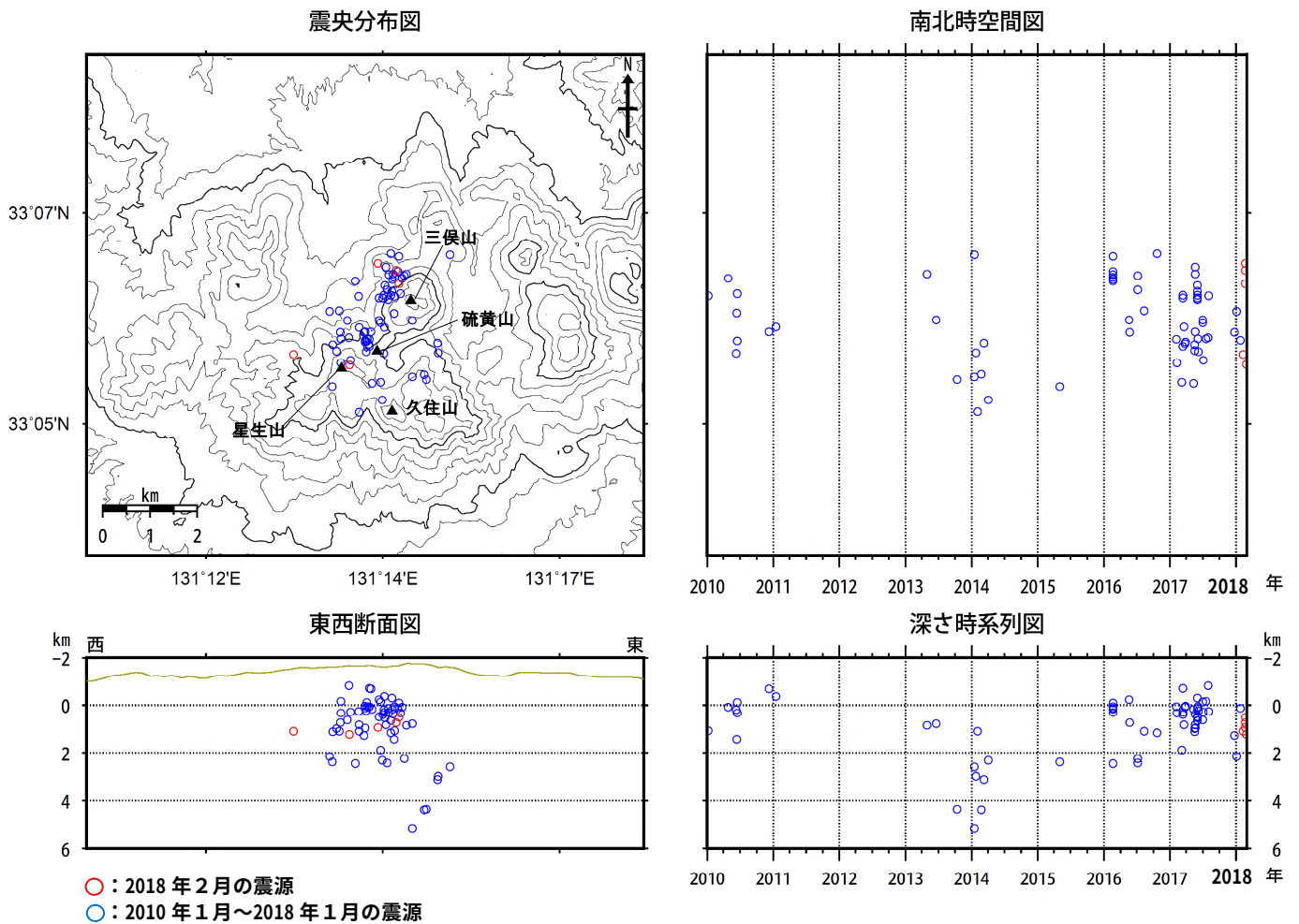
図 4 九重山 震源分布図（2010 年 1 月～2018 年 2 月）
