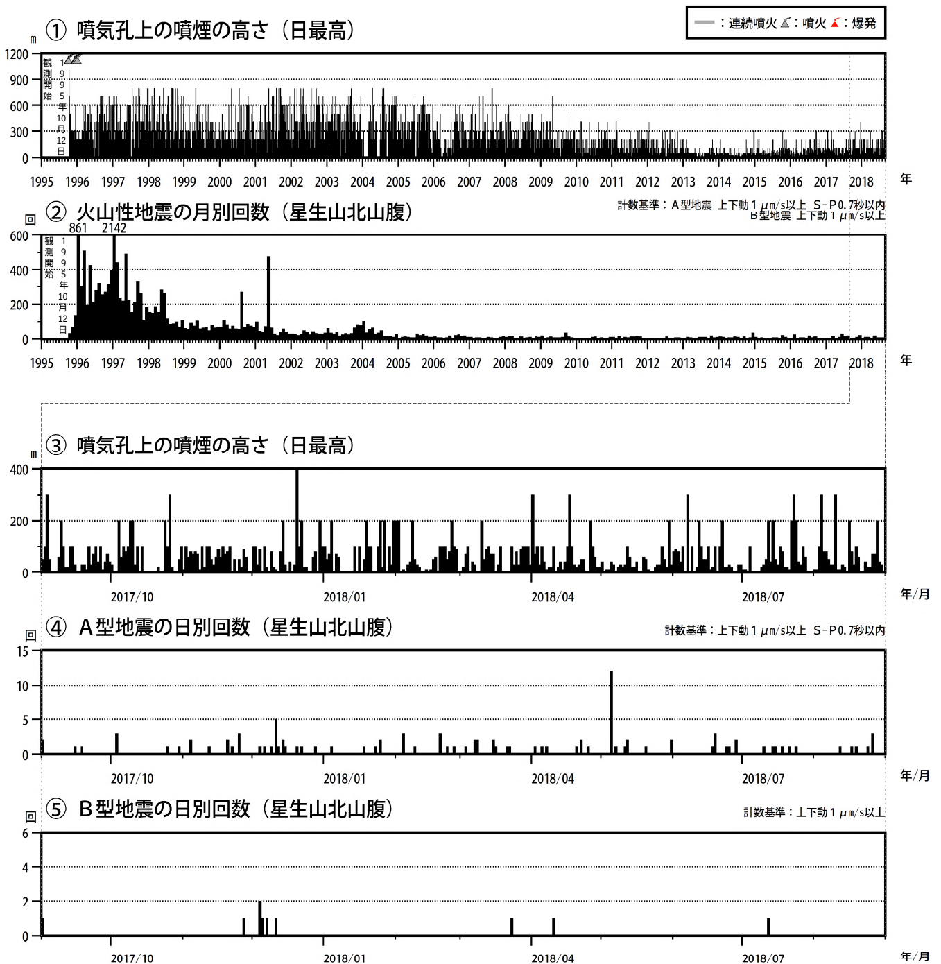
図3 九重山 火山活動経過図（1995年10月～2018年8月）
