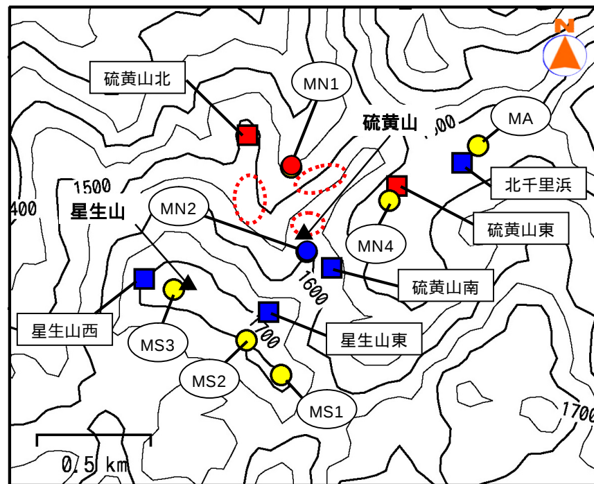
図 6 九重山 全磁力観測点配置図
