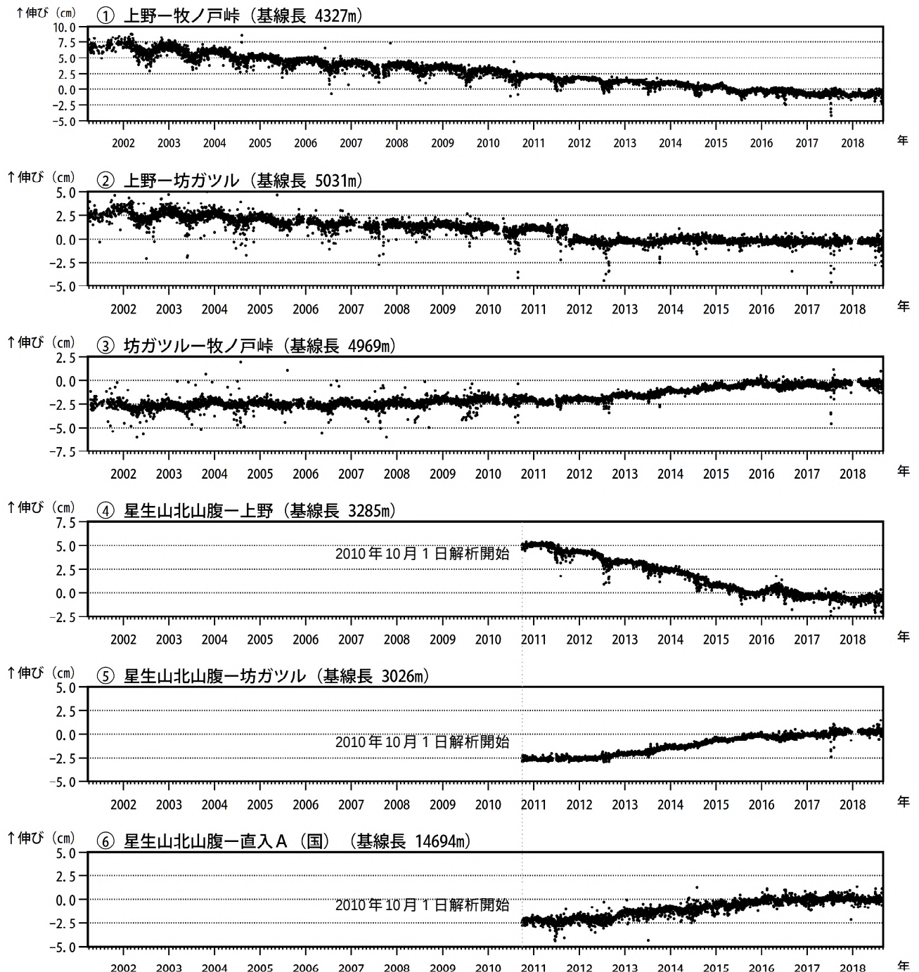
図 8-1 九重山 GNSS 連続観測による基線長変化（2001 年 3 月～2018 年 8 月）
