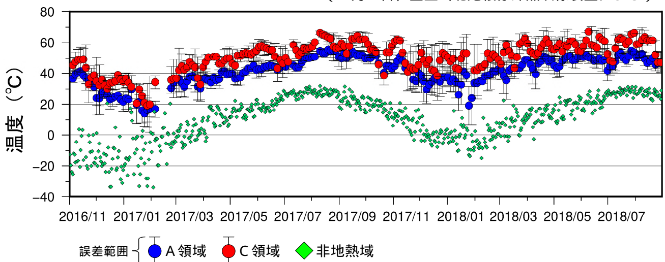
図 2-2 九重山 星生山北尾根赤外熱映像装置による日別最高温度の7日間移動平均値 (2016年11月～2018年8月)
