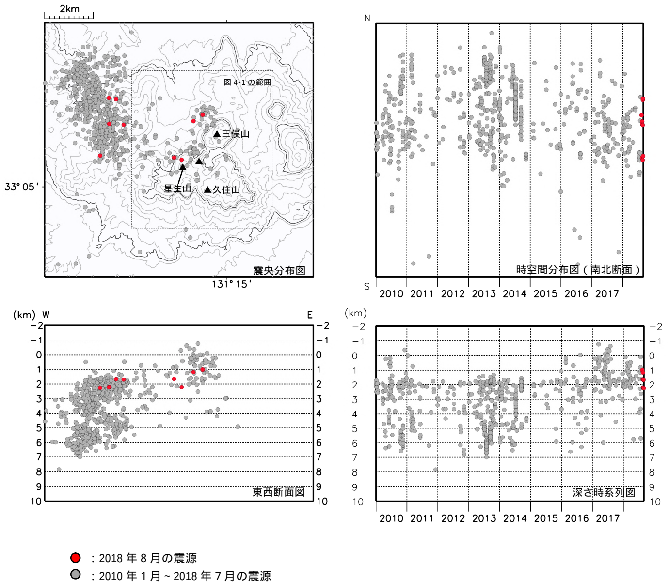
図 4-2 九重山 震源分布図（広域）（2010 年 1 月～2018 年 8 月）
