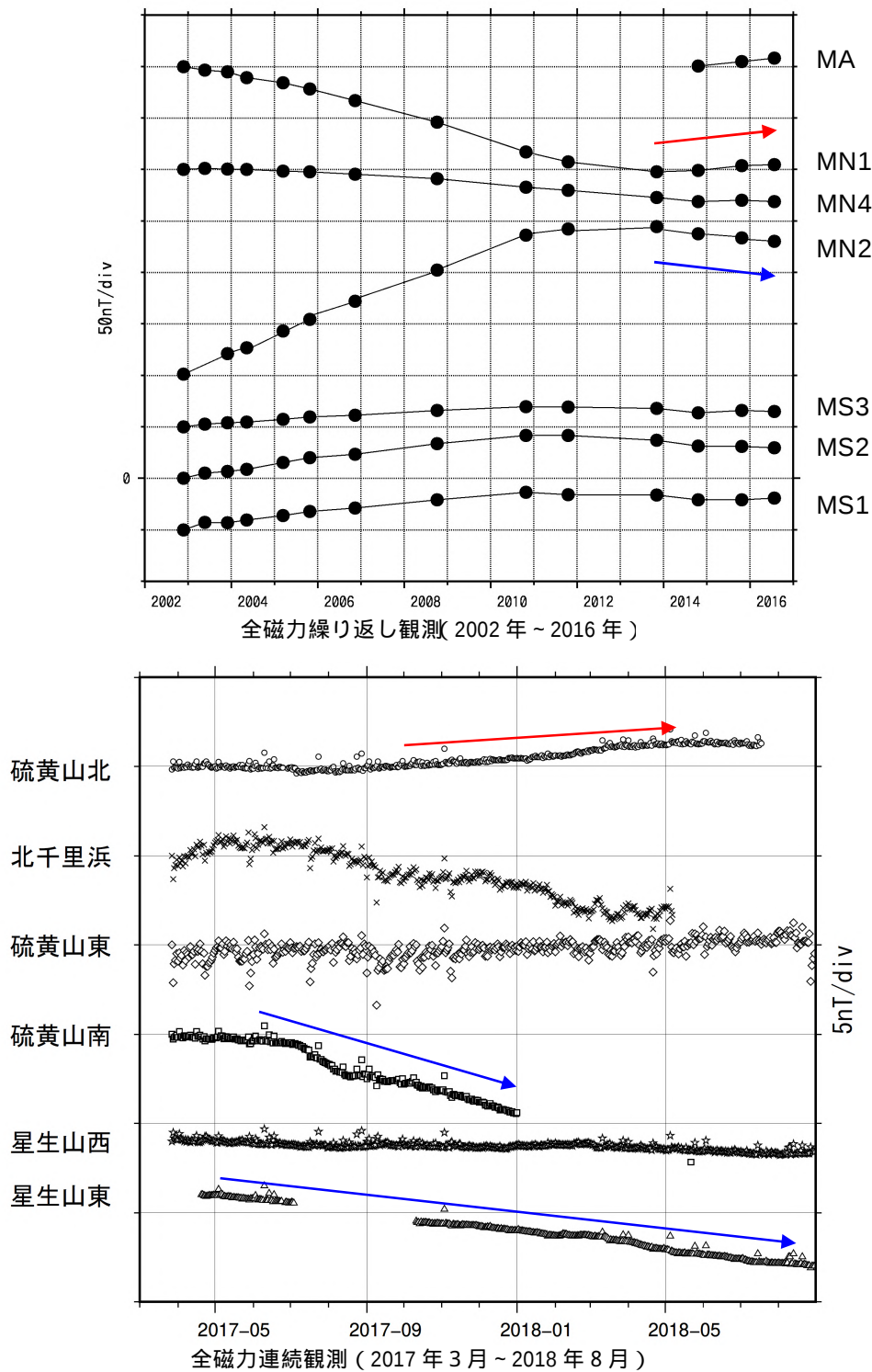
図 5 九重山 全磁力観測による値の変化
