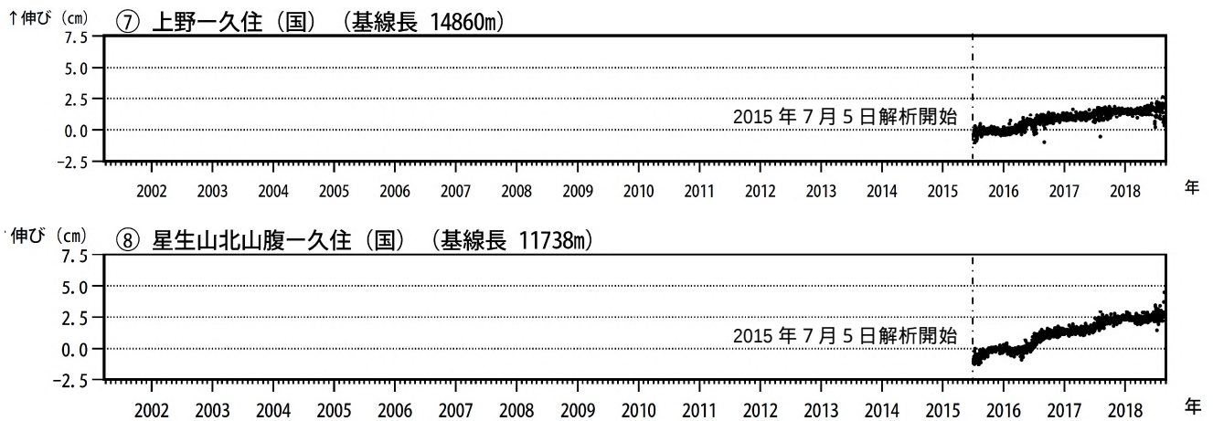
図 8-2 九重山 GNSS 連続観測による基線長変化（2001 年 3 月～2018 年 8 月）
