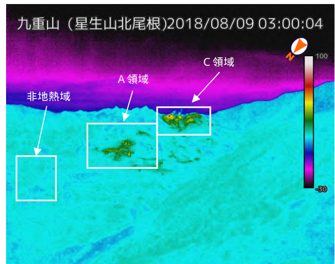
図 2-1 九重山 地熱域の状況 (8月9日、星生山北尾根赤外熱映像装置による)
