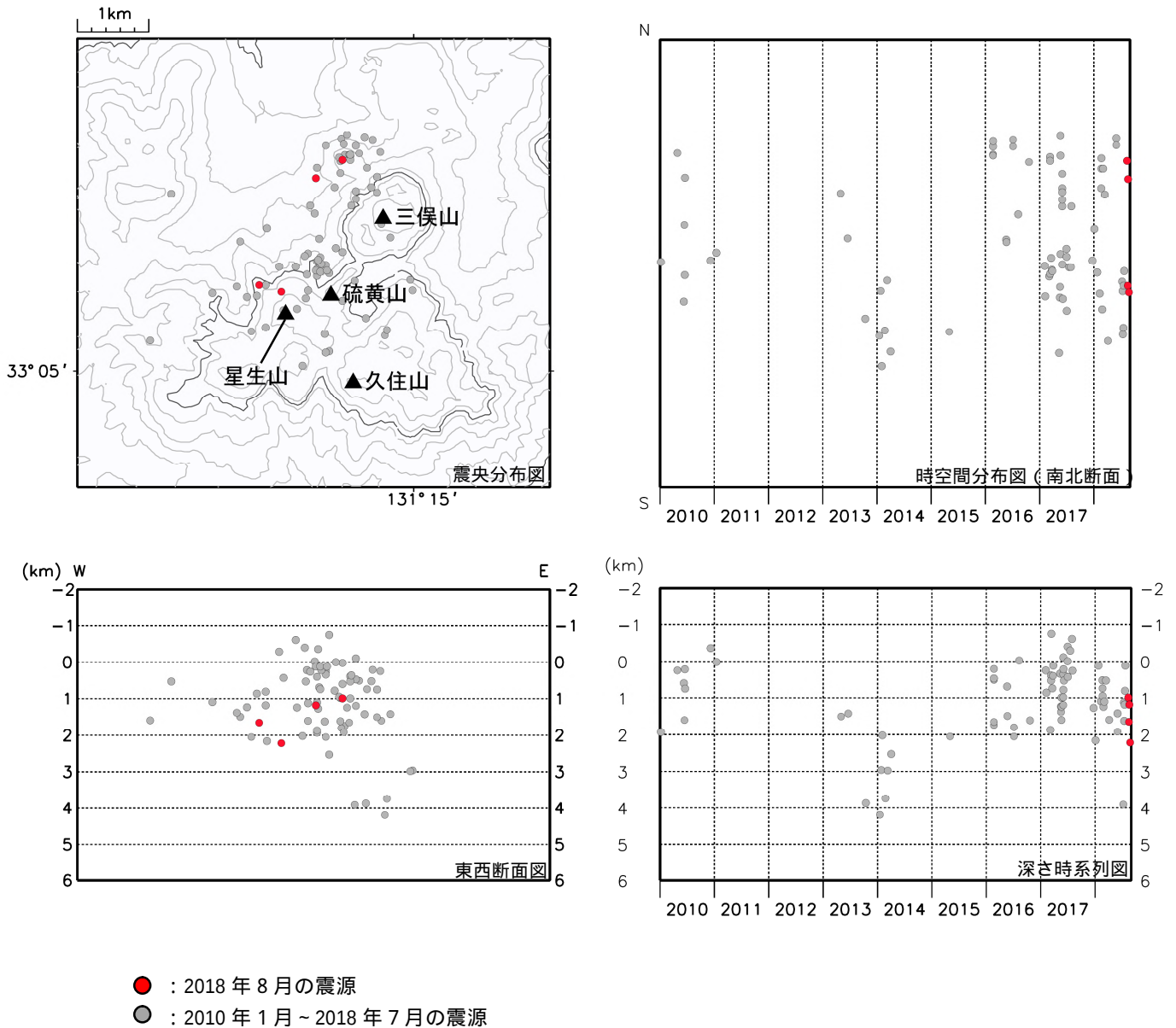
図 4-1 九重山 震源分布図（硫黄山付近の火山性地震）（2010 年 1 月～2018 年 8 月）
