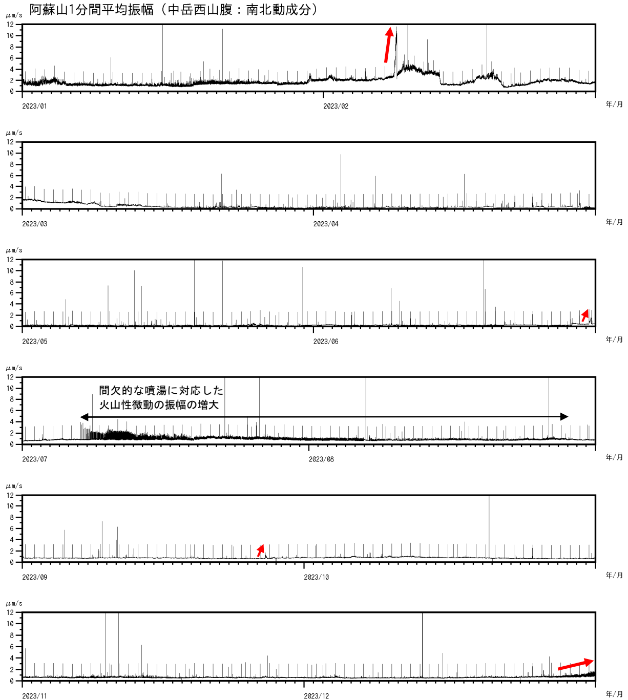
図7 阿蘇山 火山性微動の振幅の時間変化
