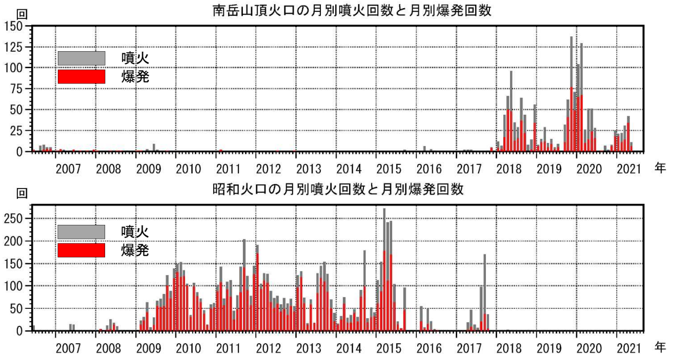
図3 桜島 南岳山頂火口（上図）と昭和火口（下図）の月別噴火回数と月別爆発回数 （2006年6月～2021年8月）
