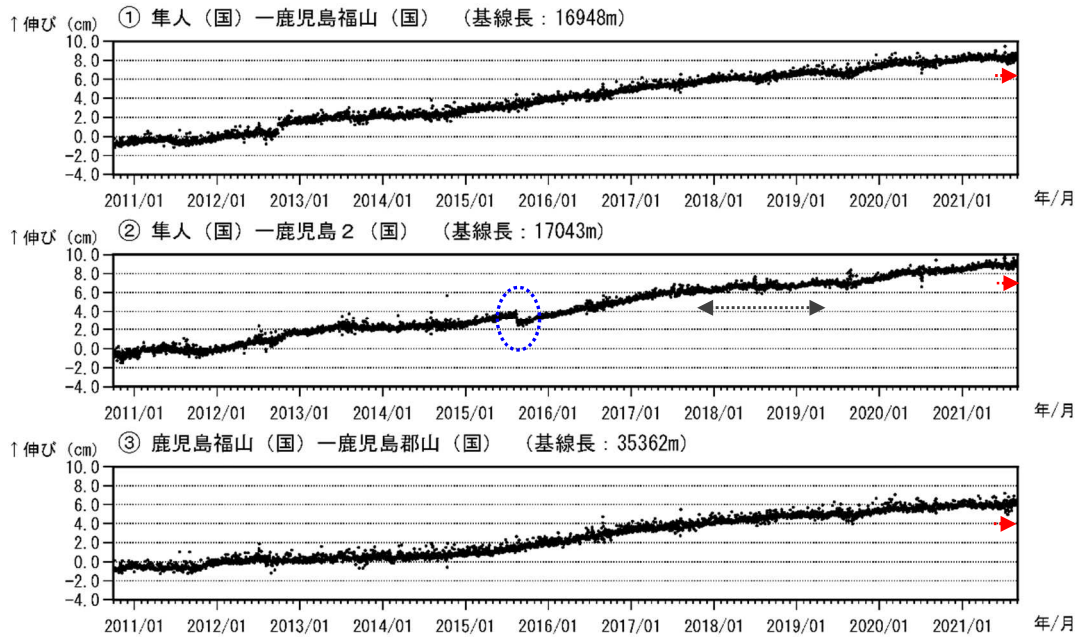
図7-1 桜島 GNSS連続観測による基線長変化（2010年10月～2021年8月）
