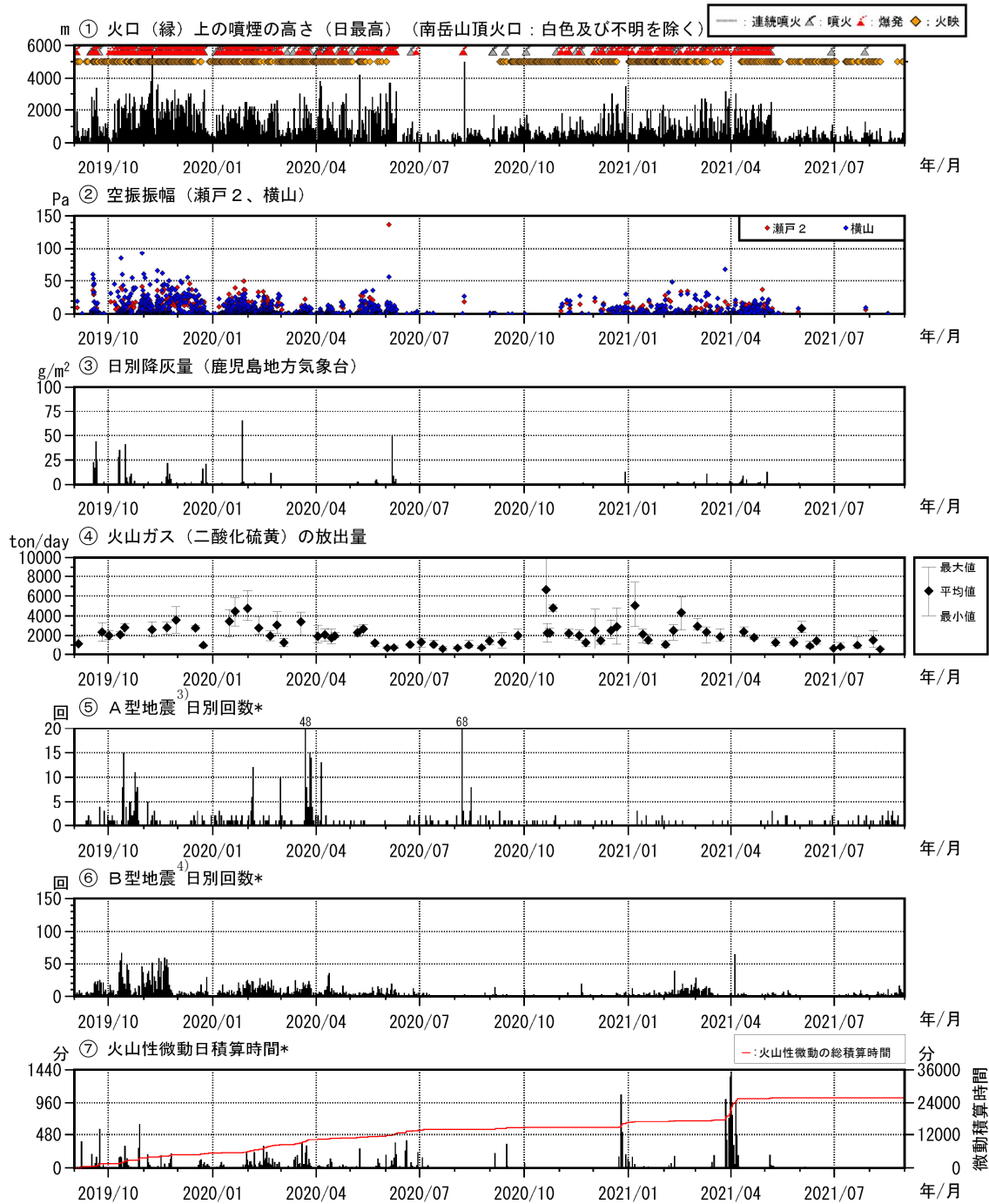
図5 桜島 最近2年間の活動経過図（2019年9月～2021年8月）
