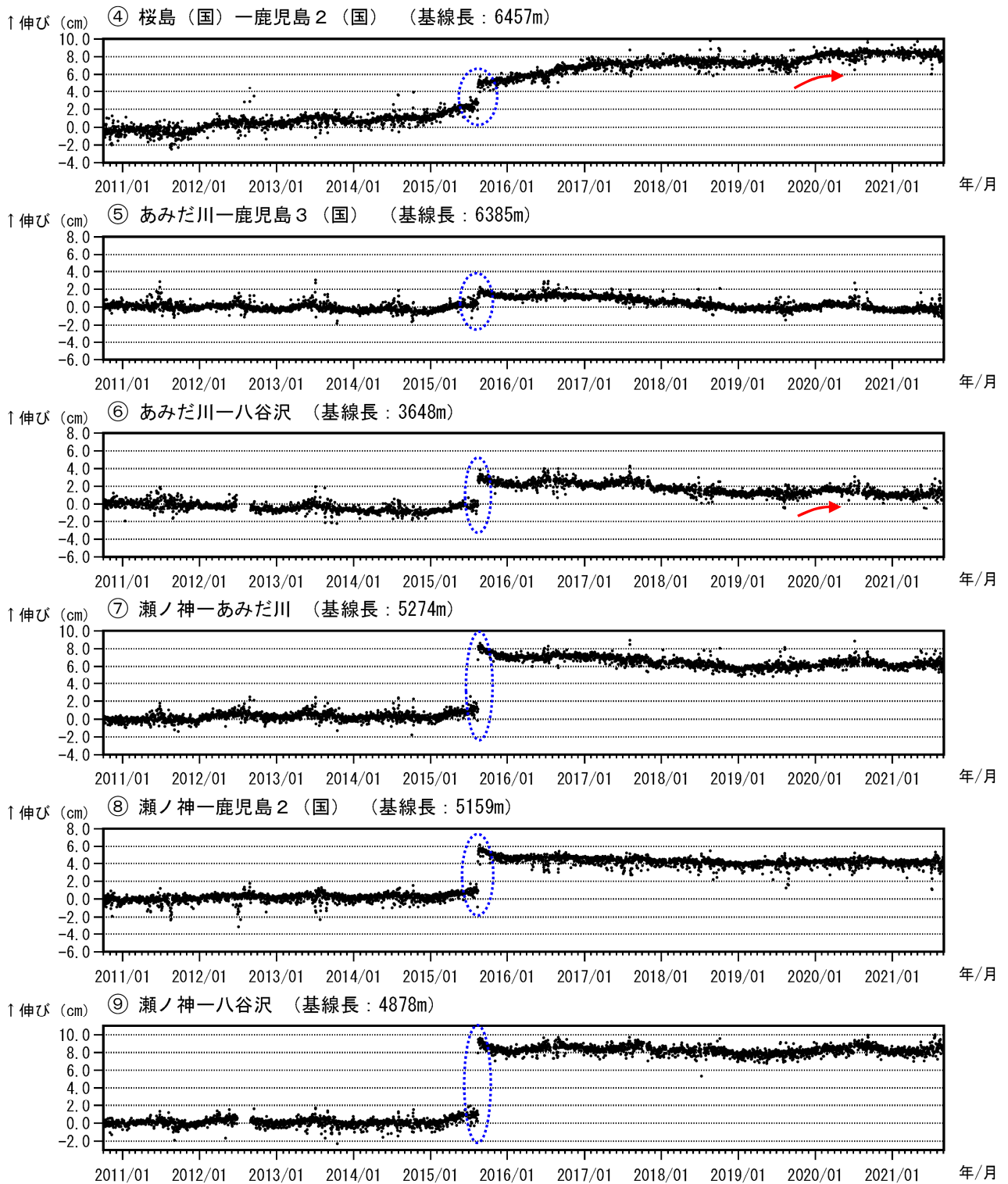
図7-2 桜島 GNSS連続観測による基線長変化 (2010年10月～2021年8月)
