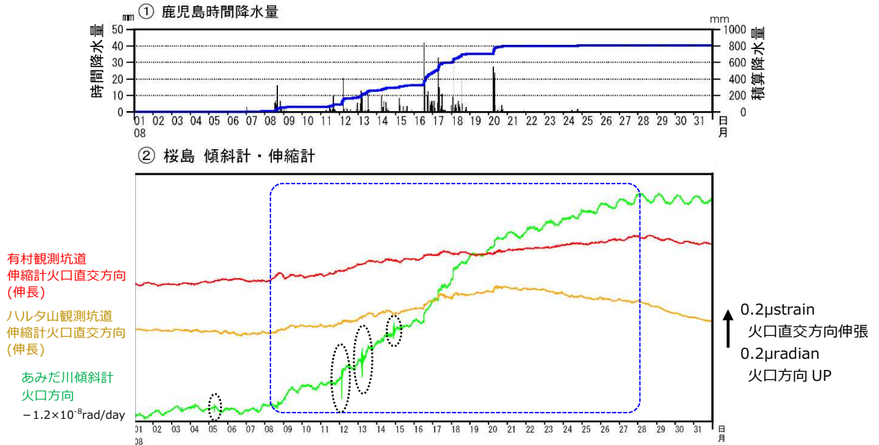
図6 桜島 傾斜計及び伸縮計による地殻変動の状況（2021年8月）
