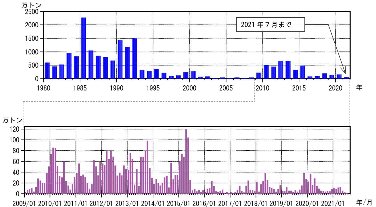
図4 桜島 鹿児島県が実施している降灰の観測データから推定した火山灰の総噴出量 （上段：1980年1月～2021年7月の年別値、下段：2009年1月～2021年7月の月別値）
