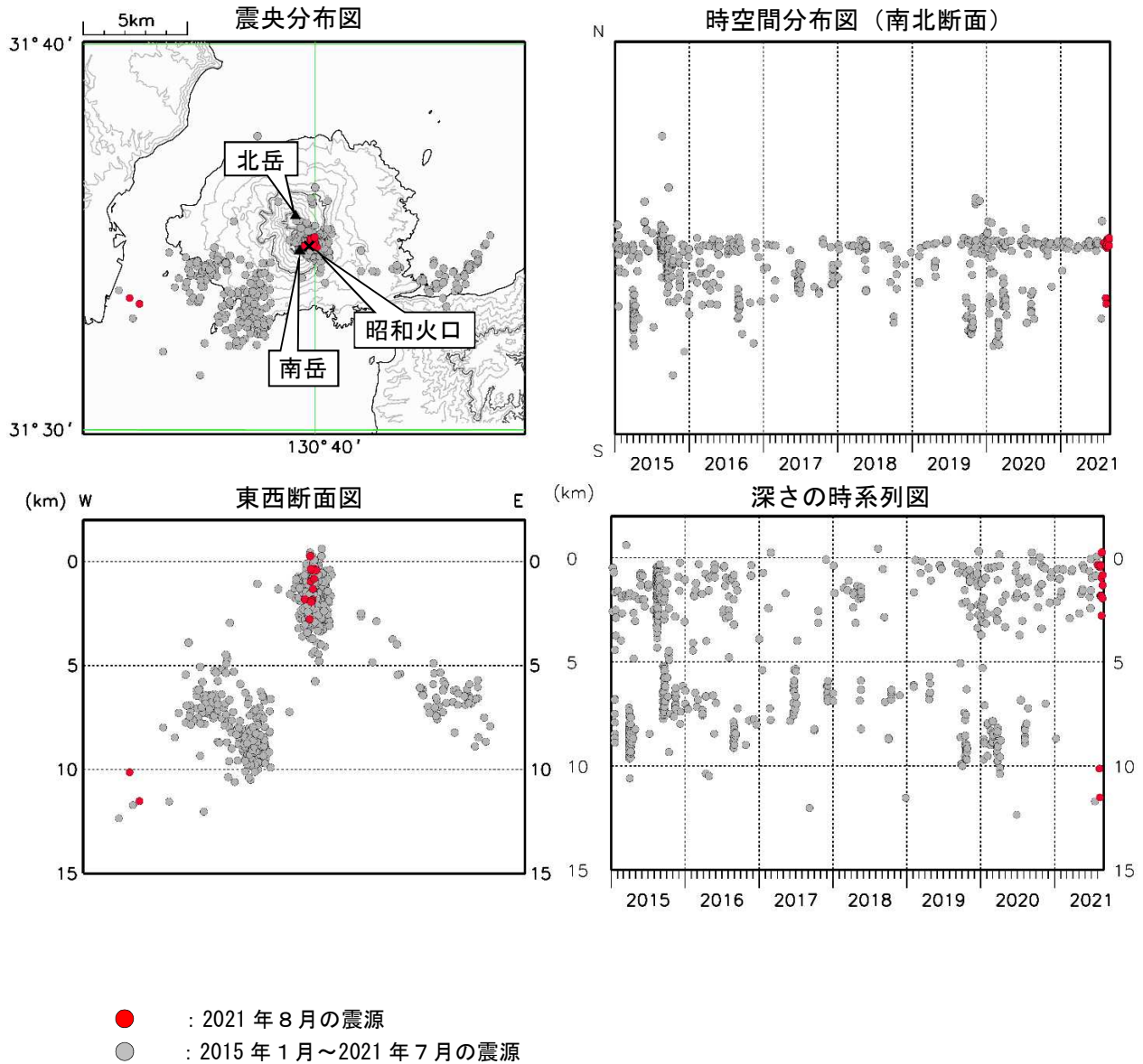
図2 桜島 震源分布図（2015年1月～2021年8月）
