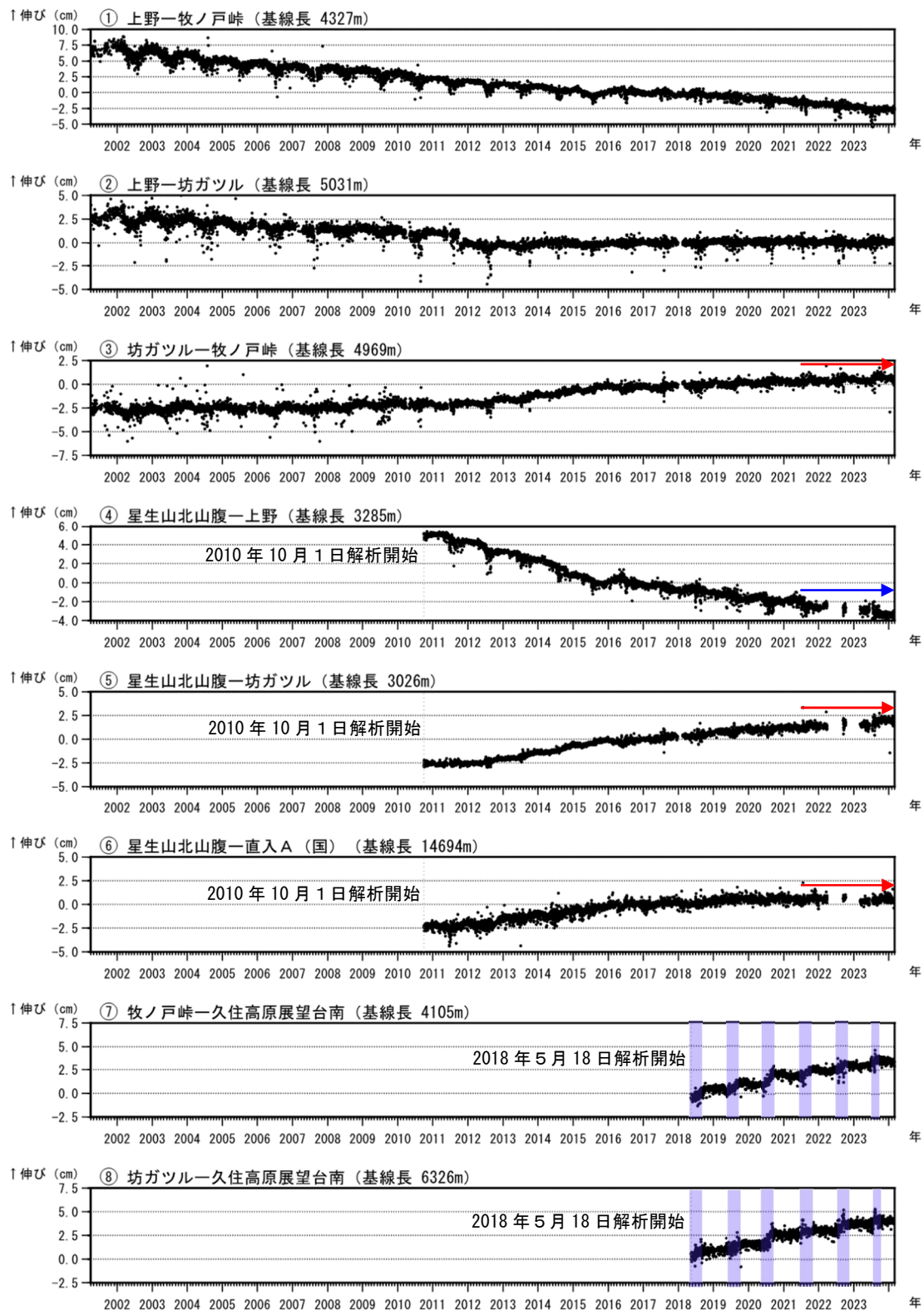
図5 九重山 GNSS 連続観測による基線長変化（2001年4月～2024年2月）
