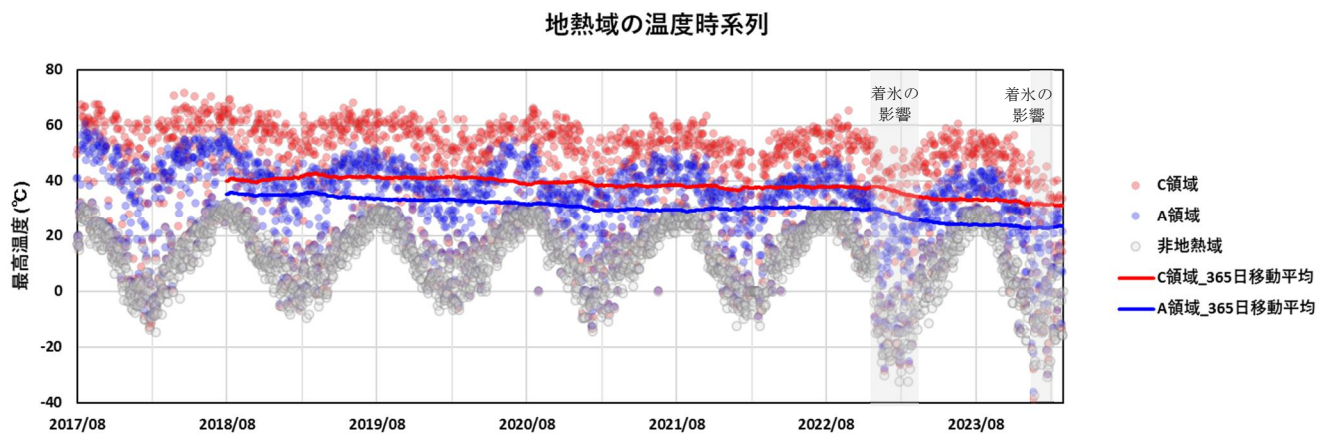
図 1-2 九重山 星生山北尾根の赤外熱映像装置による日別最高温度（2017年8月～2024年2月）
