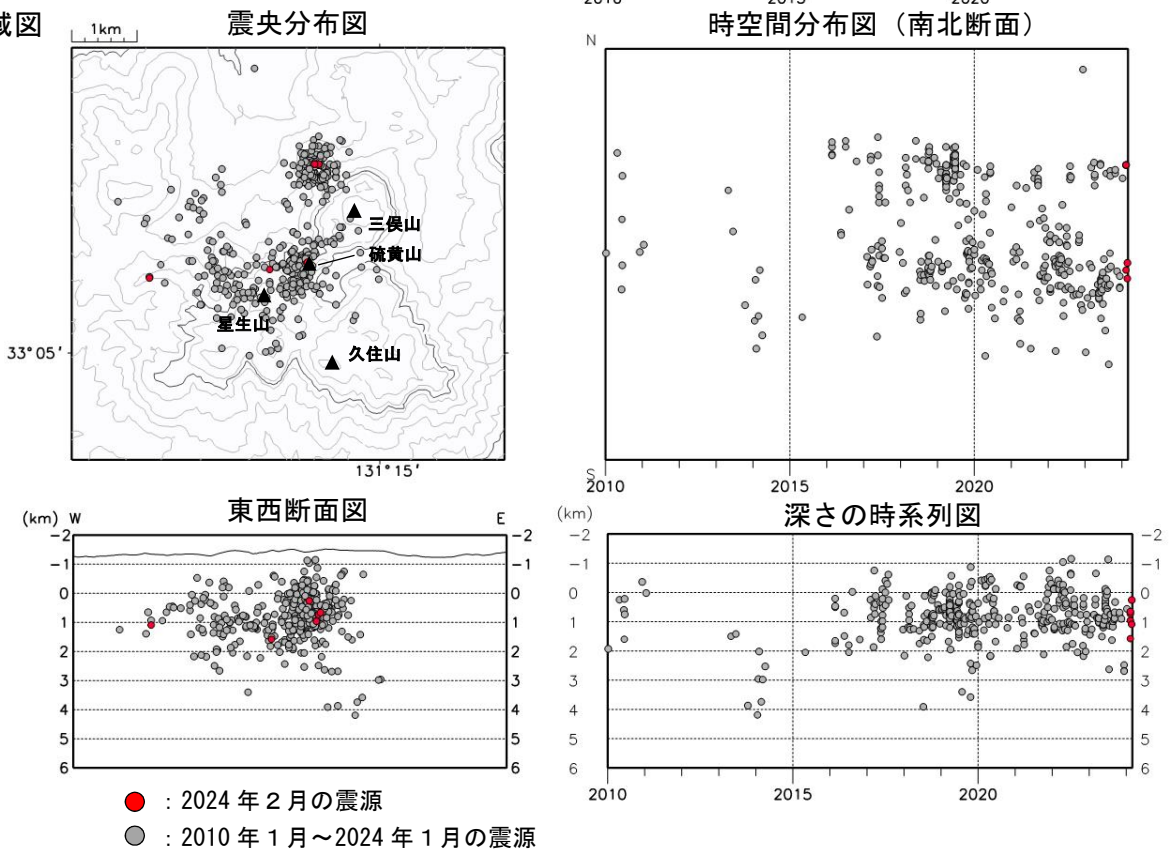
図3 九重山 震源分布図 ①広域図 ②狭域図（2010年1月～2024年2月）
