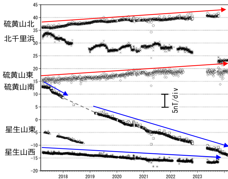
図 4-1 九重山 連続観測による全磁力の変化 (2017年3月～2024年2月)
