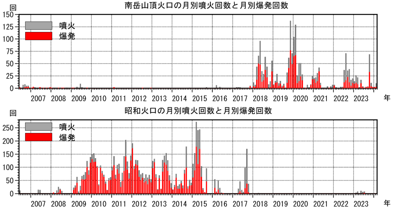
図4 桜島 南岳山頂火口（上図）と昭和火口（下図）の月別噴火回数と月別爆発回数 （2006年6月～2024年2月）
