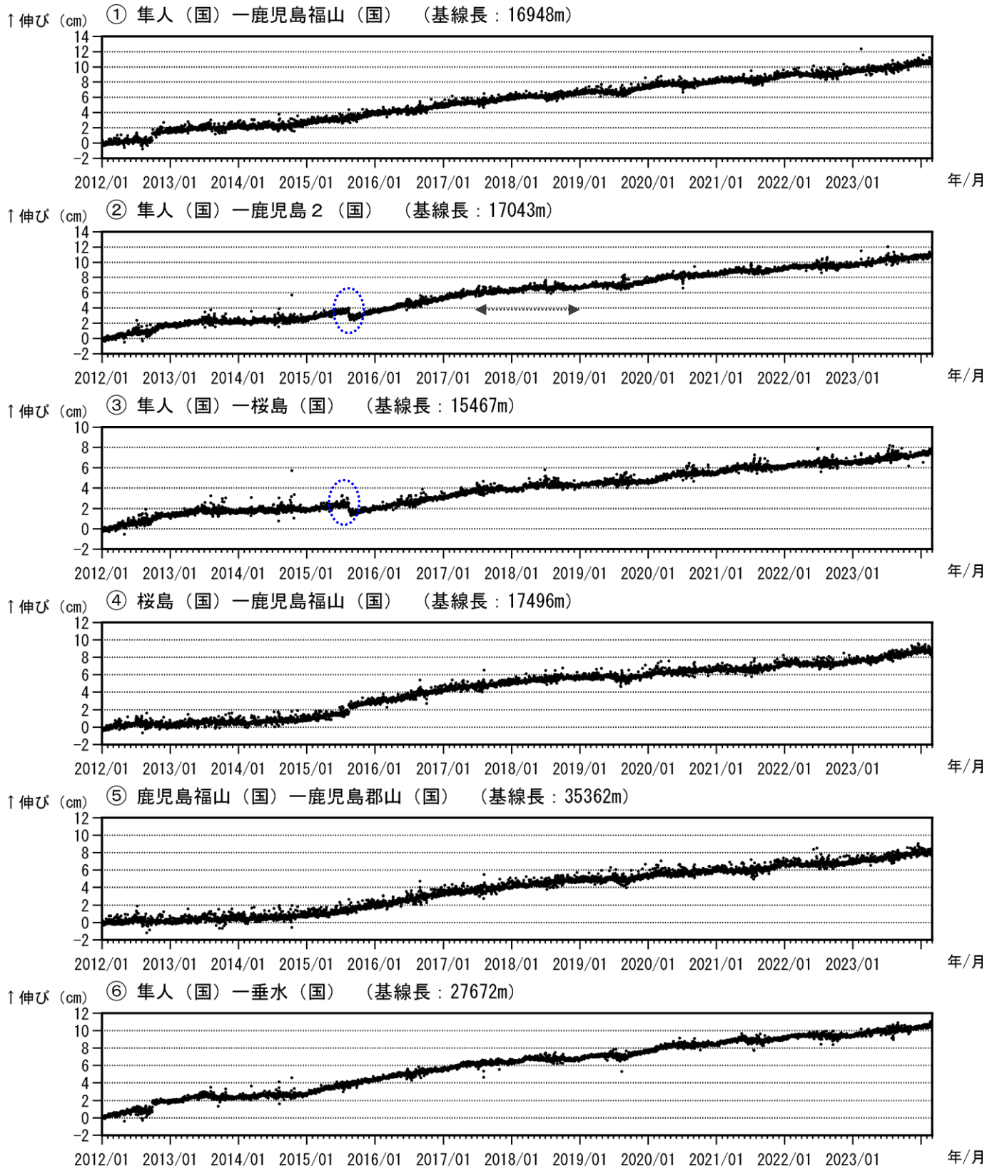
図 8-1 桜島 GNSS 連続観測による基線長変化 (2012 年 1 月～2024 年 2 月)
