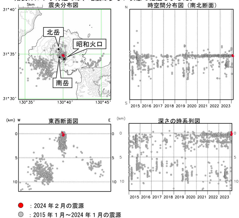
図 3-2 桜島 桜島付近の震源分布図（2015 年 1 月～2024 年 2 月）
