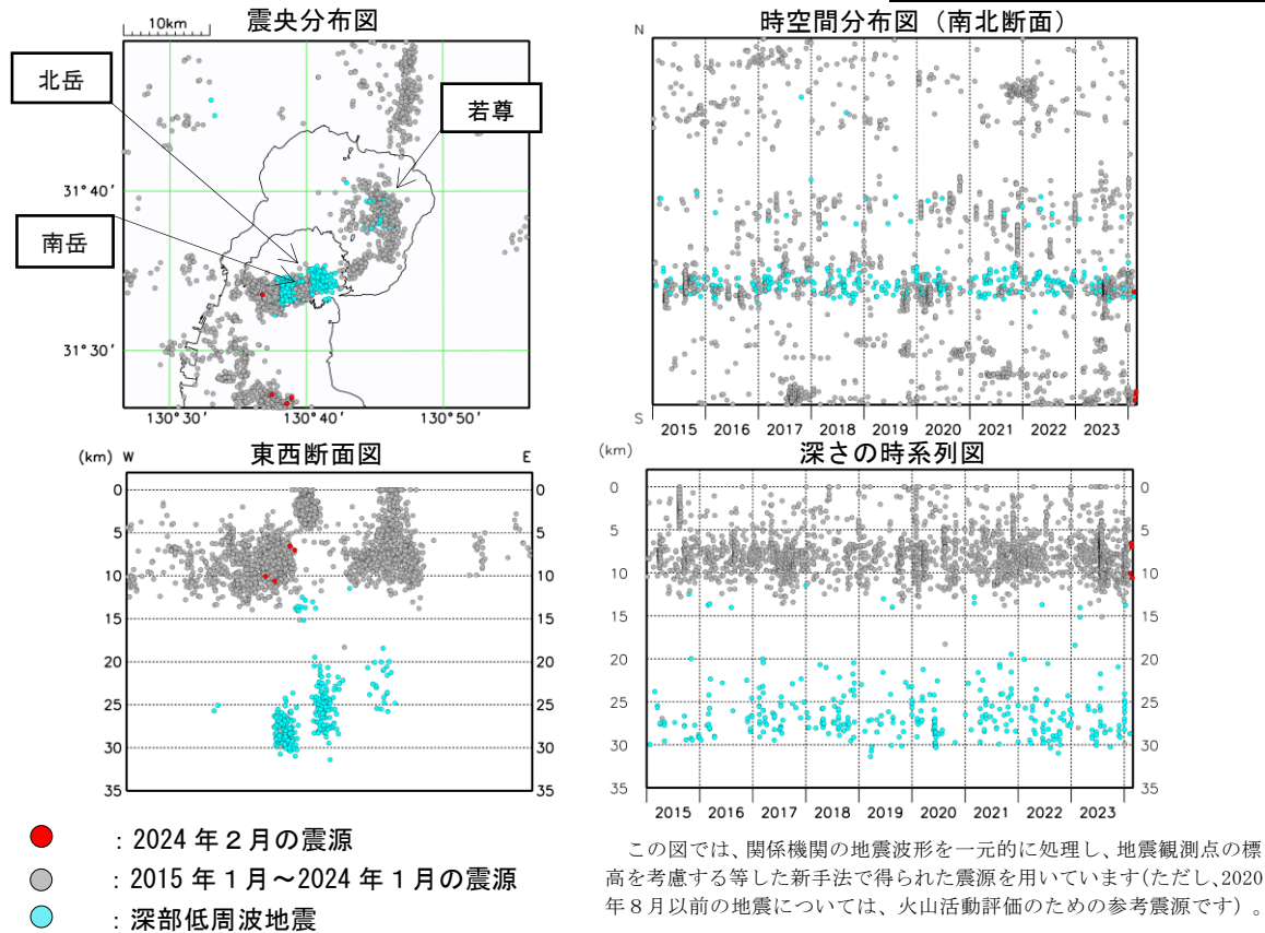
図 3-1 桜島 始良カルデラ周辺の震源分布図（2015 年 1 月～2024 年 2 月）
