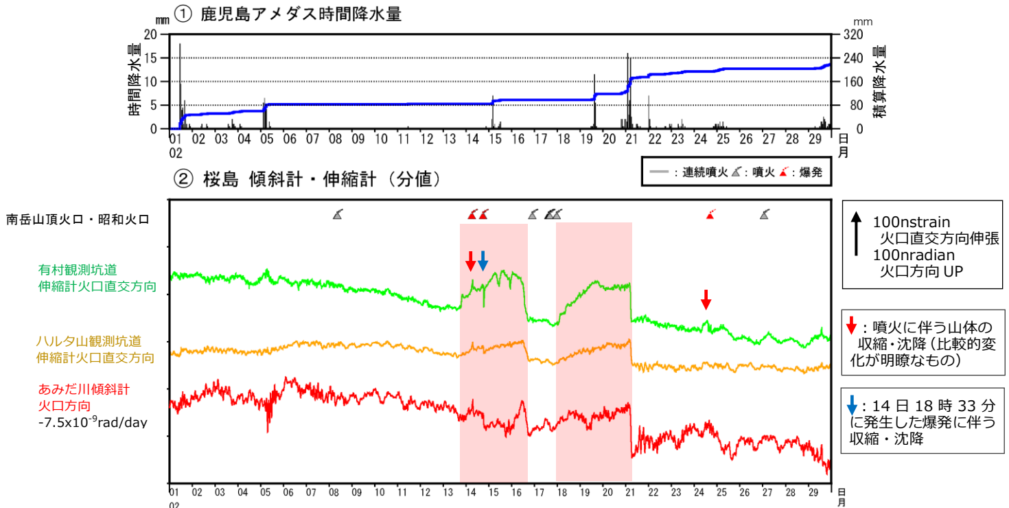
図7 桜島 傾斜計及び伸縮計による地殻変動の状況（2024年2月）
