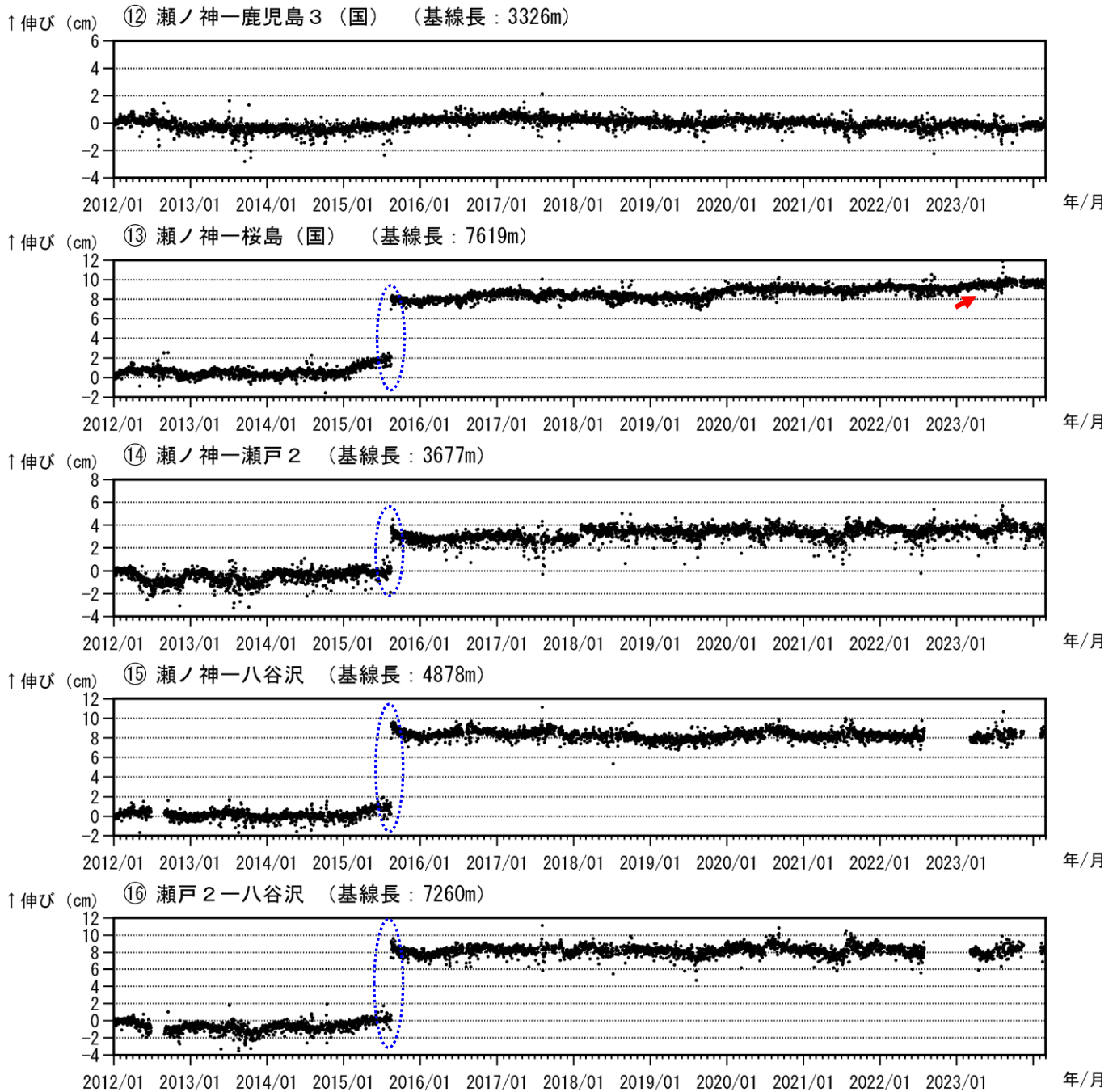
図 8-3 桜島 GNSS 連続観測による基線長変化 (2012 年 1 月～2024 年 2 月)
