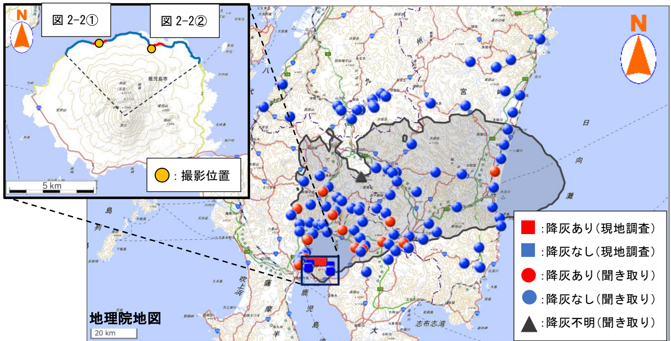
図 2-1 桜島 14 日 18 時 33 分の爆発に伴う降灰調査及び図 2-2 の撮影位置
