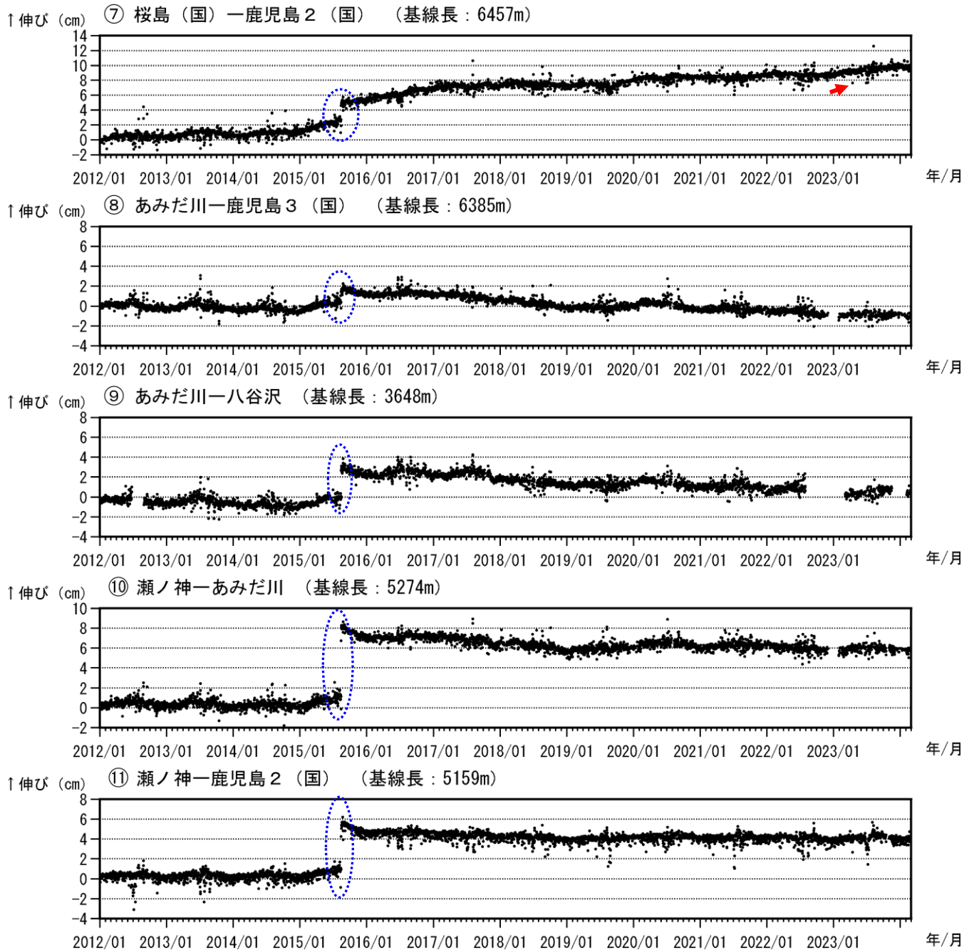
図 8-2 桜島 GNSS 連続観測による基線長変化 (2012 年 1 月～2024 年 2 月)
