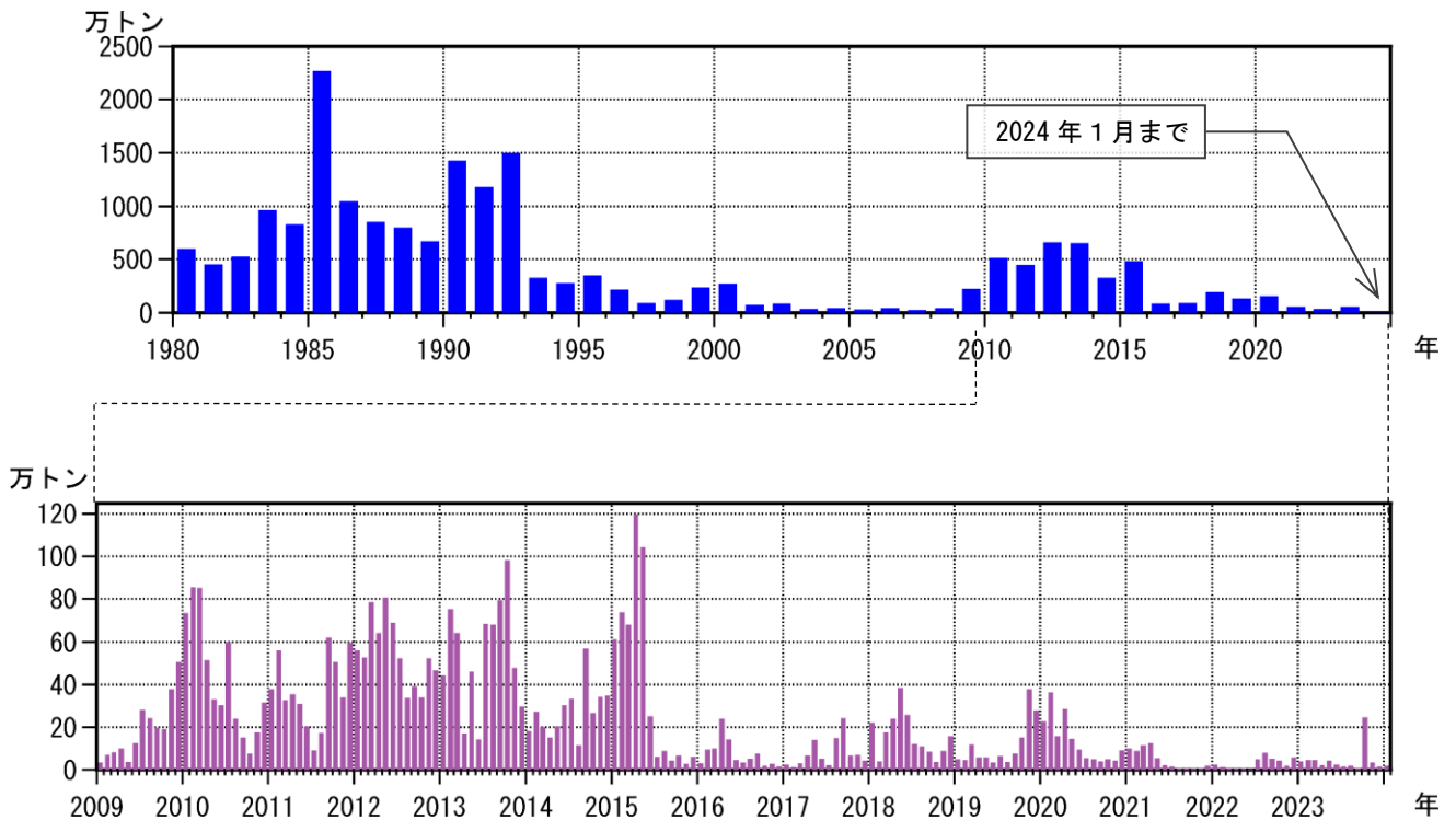
図5 桜島 鹿児島県が実施している降灰の観測データから推定した火山灰の総噴出量 （上段：1980年1月～2024年1月の年別値、下段：2009年1月～2024年1月の月別値）
