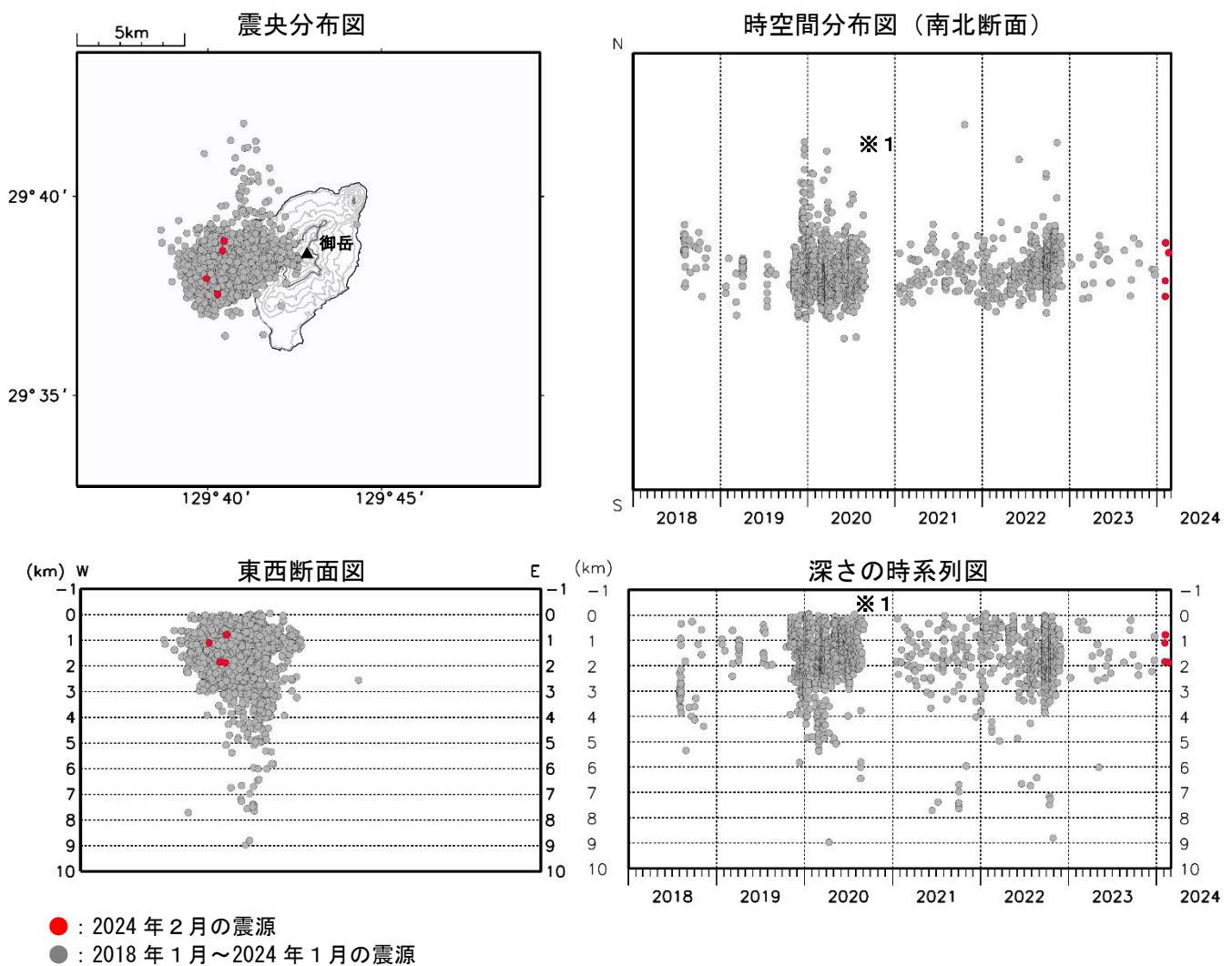
図4 諏訪之瀬島 震源分布図（2018年1月～2024年2月）
