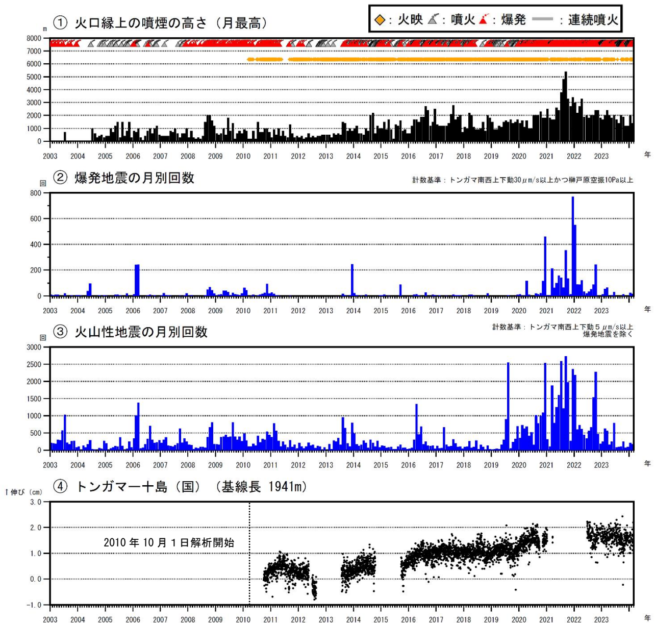
図2 諏訪之瀬島 長期の火山活動経過図（2003年1月～2024年2月）
