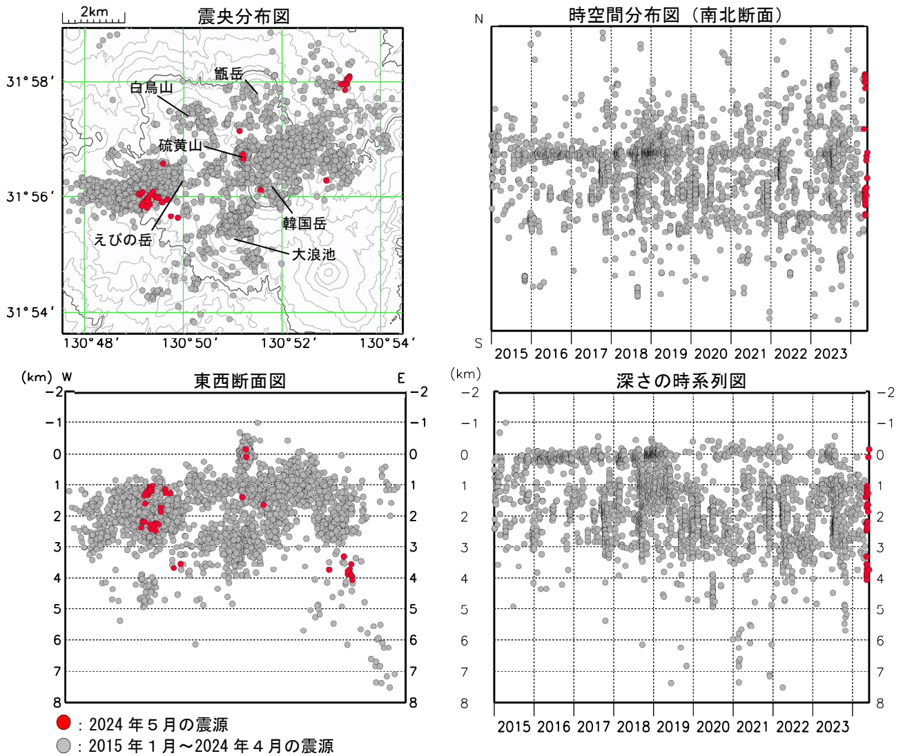
図5 霧島山（えびの高原（硫黄山）周辺） 震源分布図（2015 年 1 月～2024 年 5 月）
