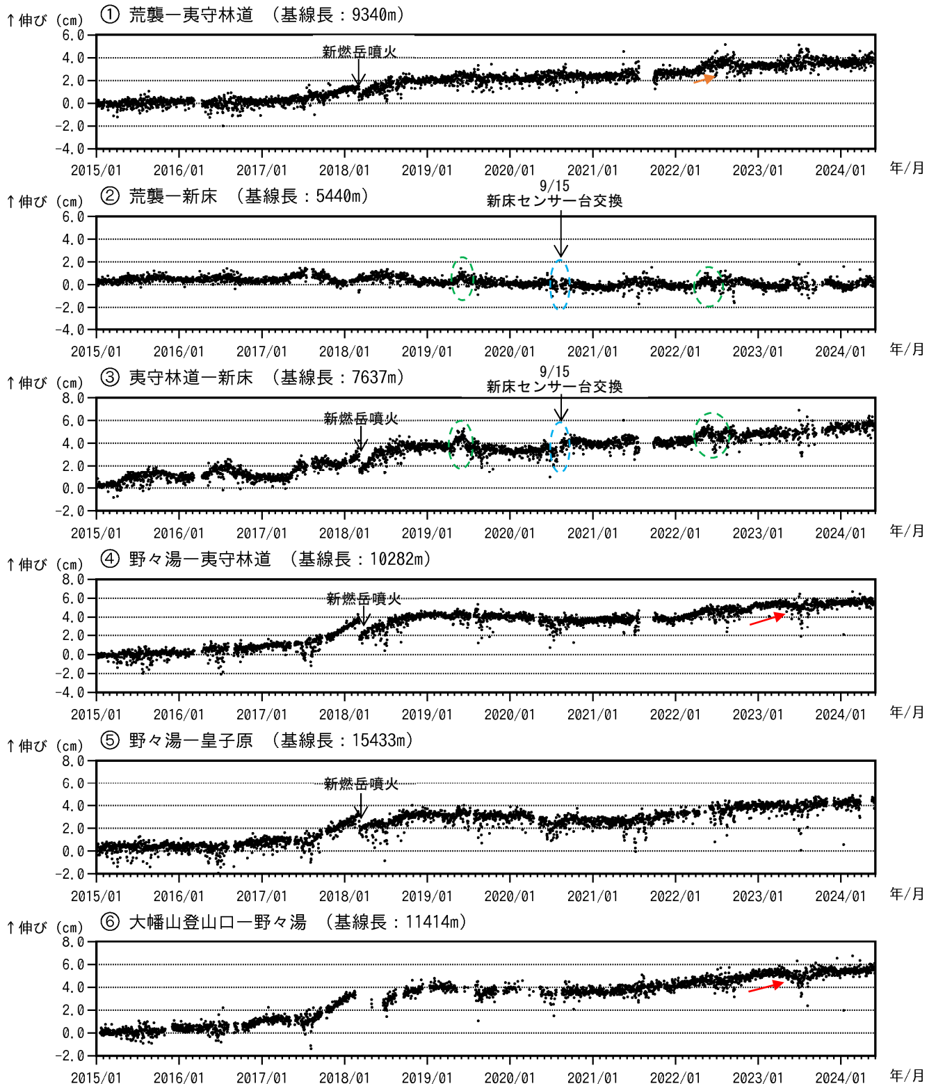
図4 霧島山（新燃岳） GNSS 連続観測による基線長変化（2015年1月～2024年5月）
