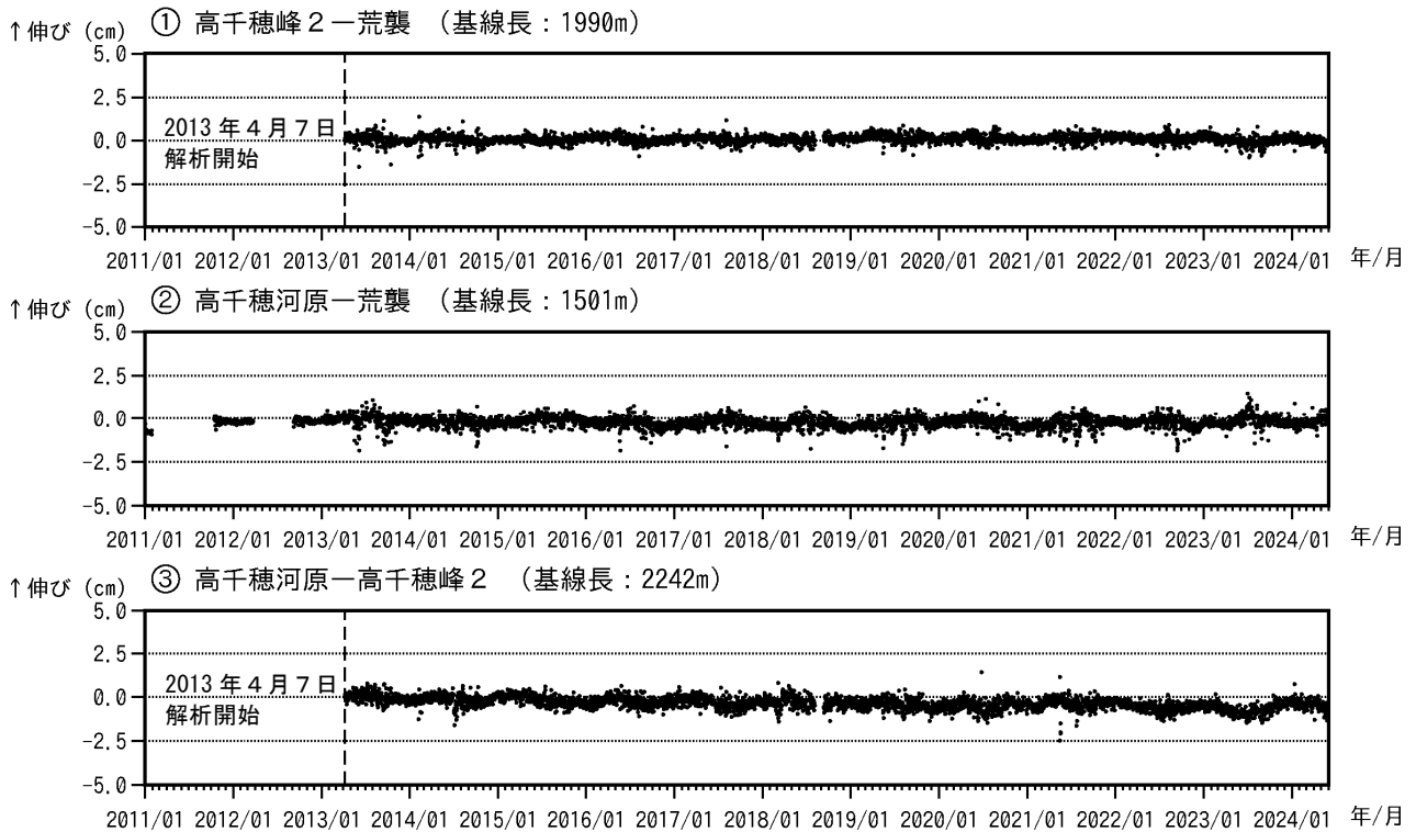
図4 霧島山（御鉢） GNSS 連続観測による基線長変化（2011年1月～2024年5月）
