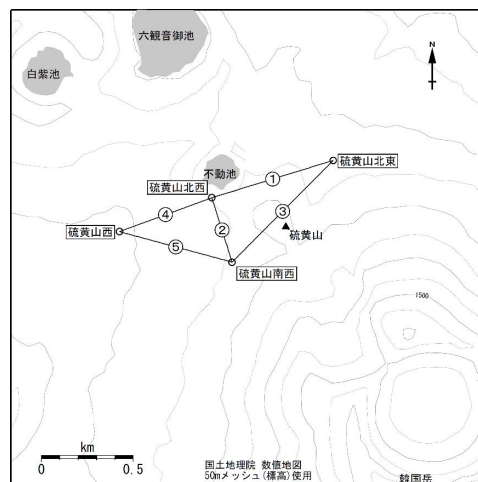
図6 霧島山（えびの高原（硫黄山）周辺） 図4及び図7のGNSS連続観測点と基線番号 白丸（○）は気象庁の観測点位置を示しています。
