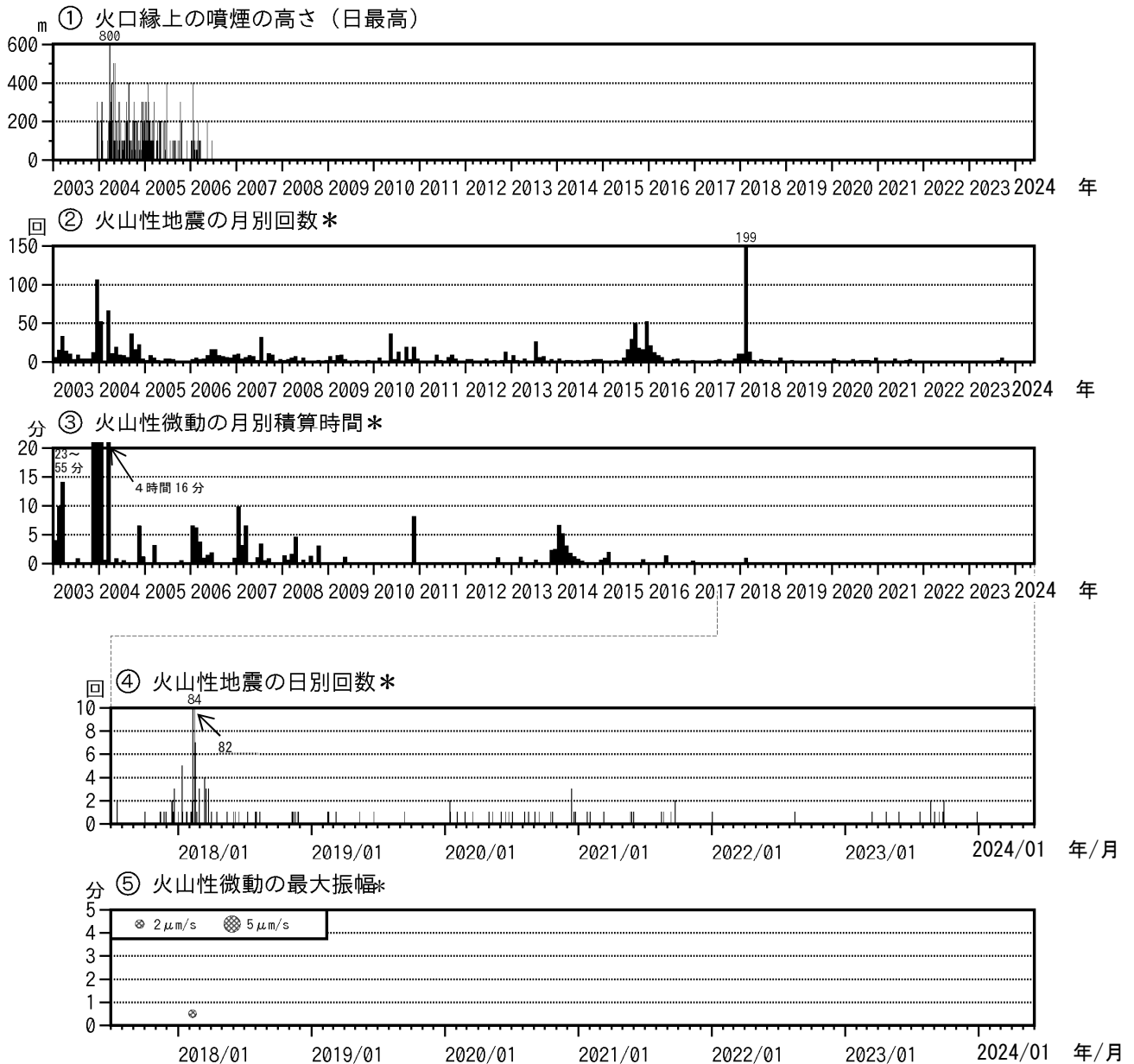
図3 霧島山（御鉢） 火山活動経過図（2003年1月～2024年5月）
