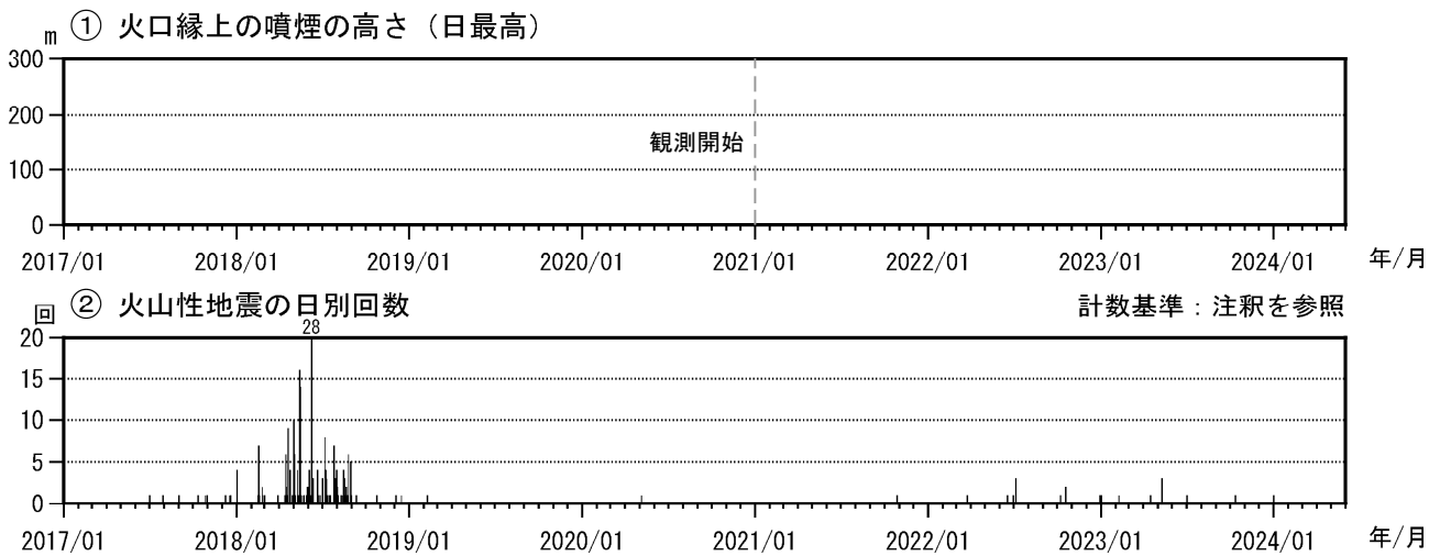
図2 霧島山（大幡池） 火山活動経過図（2017年1月～2024年5月）
