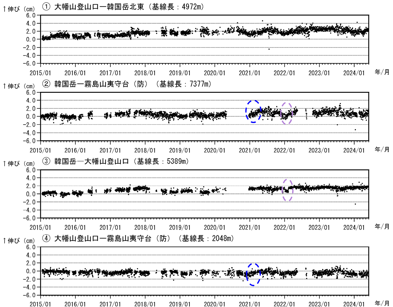
図4 霧島山（大幡池） GNSS 連続観測による基線長変化（2015年1月～2024年5月）
