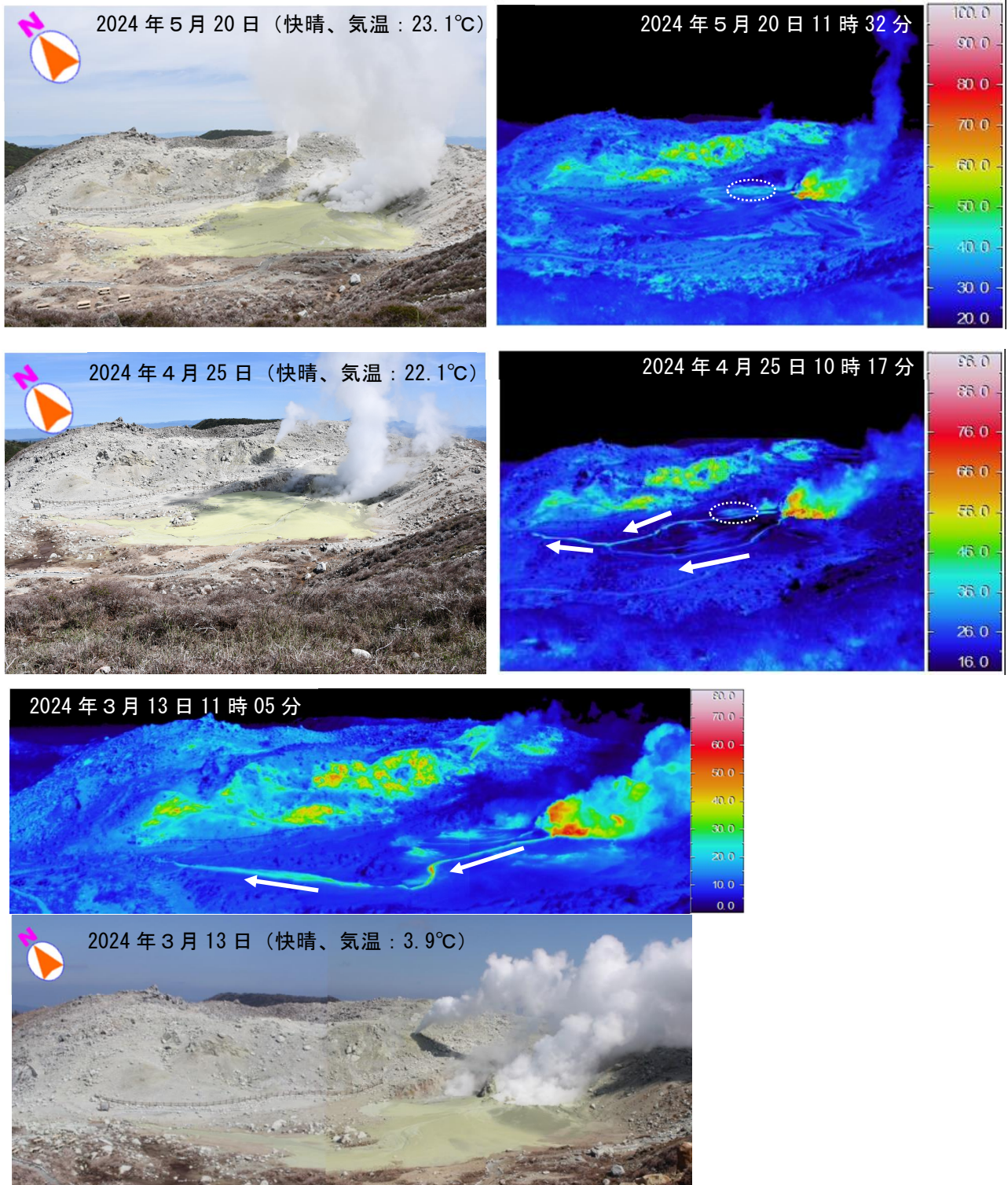
図3 霧島山（えびの高原（硫黄山）周辺） 硫黄山の南側の噴気及び地熱域の状況 （硫黄山南2全磁力観測点付近（図2）から観測）
