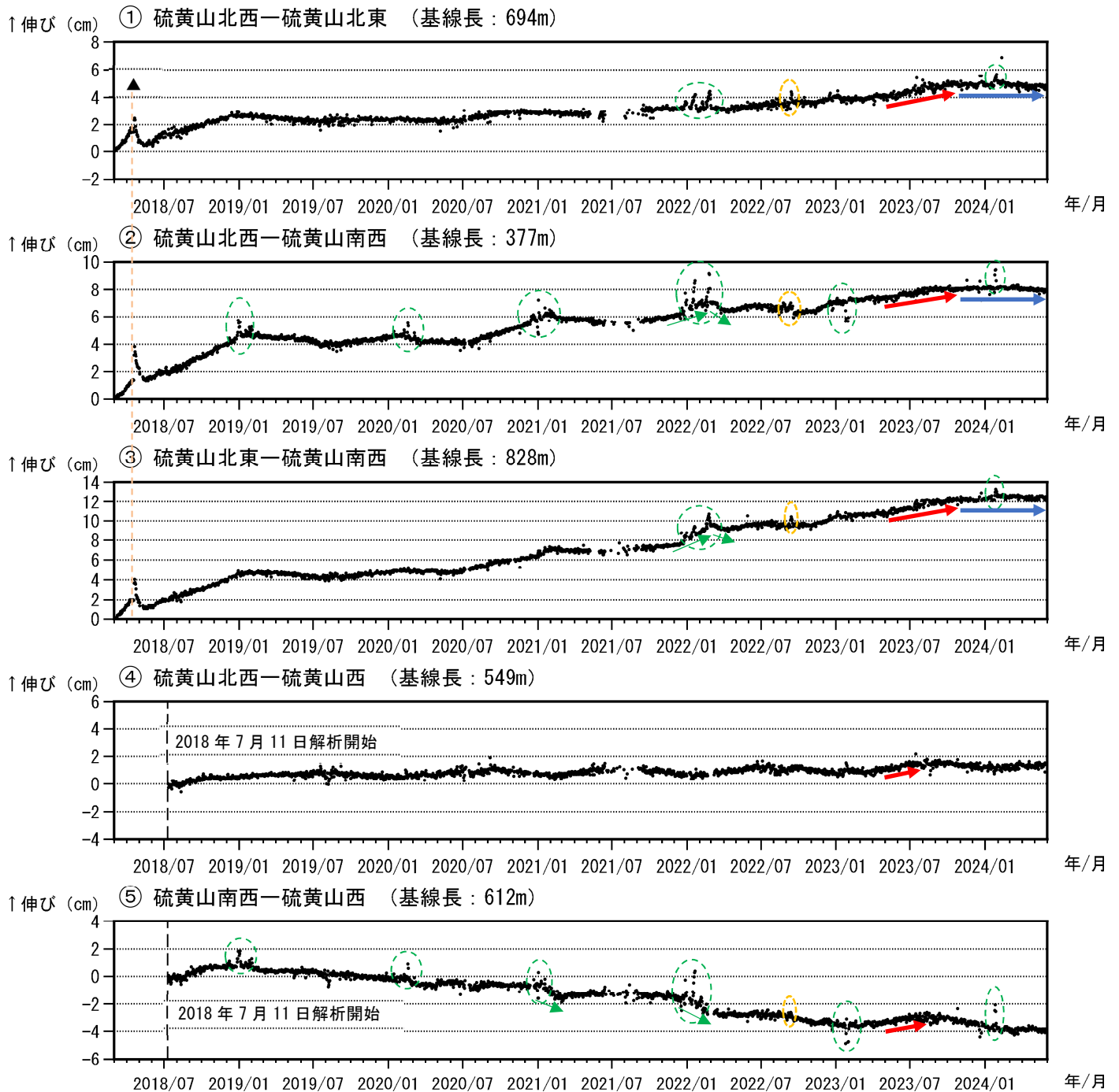
図7 霧島山（えびの高原（硫黄山）周辺） GNSS 連続観測による基線長変化 (2018年3月～2024年5月)
