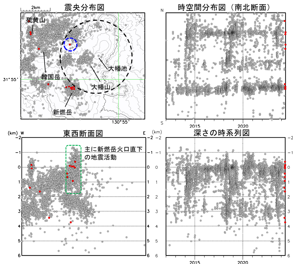
図3 霧島山（大幡池） 震源分布図（2012年1月～2024年5月）
