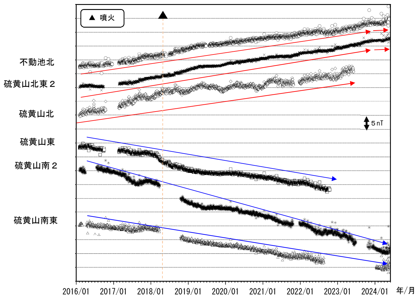
図 8-2 霧島山（えびの高原（硫黄山）周辺） 全磁力観測点で観測された全磁力変動 （2016 年 1 月～2024 年 5 月）
