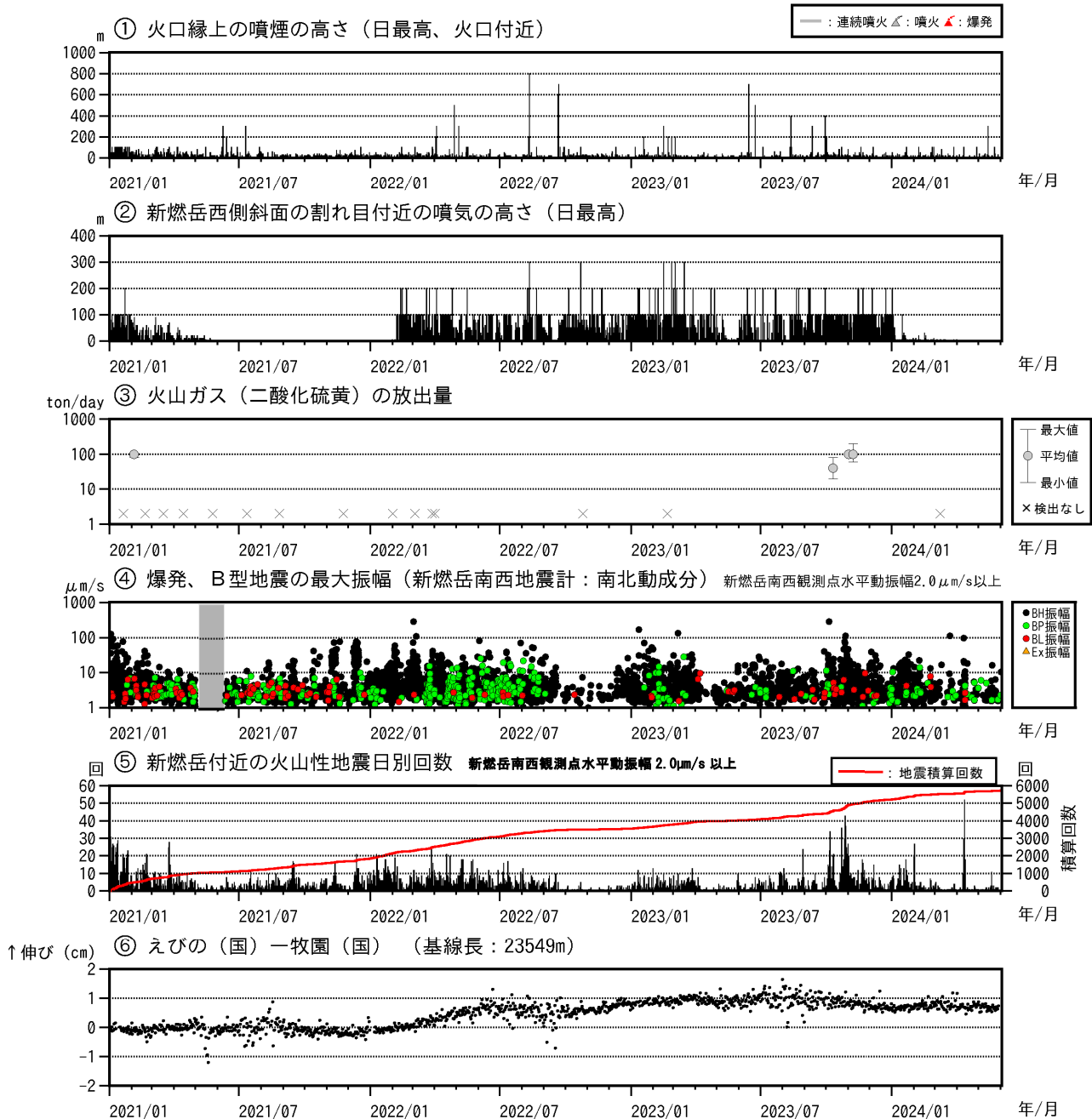
図2 霧島山（新燃岳） 火山活動経過図（2021年1月～2024年5月）
