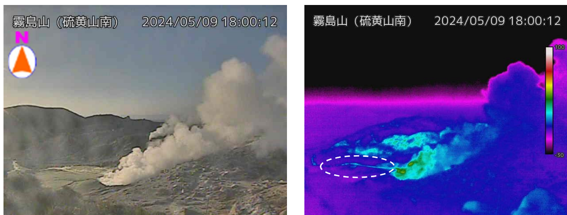
図 1-2 霧島山（えびの高原（硫黄山）周辺） 硫黄山南側の状況 （5月9日、硫黄山南監視カメラ）
