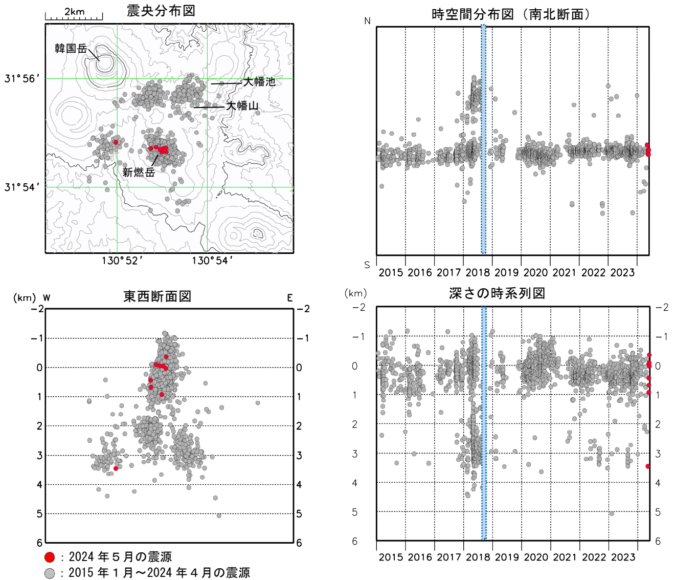
図3 霧島山（新燃岳） 震源分布図（2015 年 1 月～2024 年 5 月）
