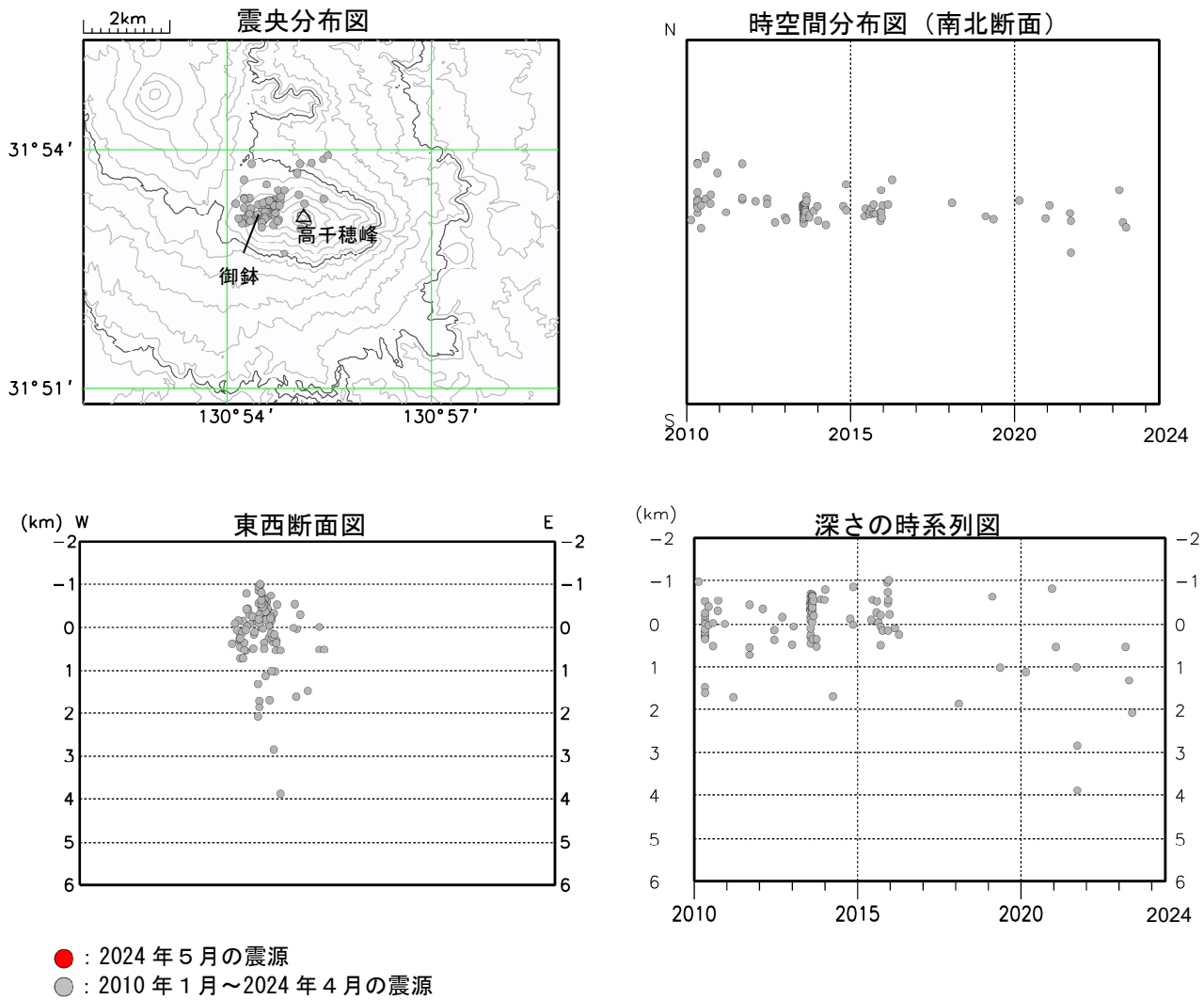
図2 霧島山（御鉢） 震源分布図（2010 年 1 月～2024 年 5 月）
