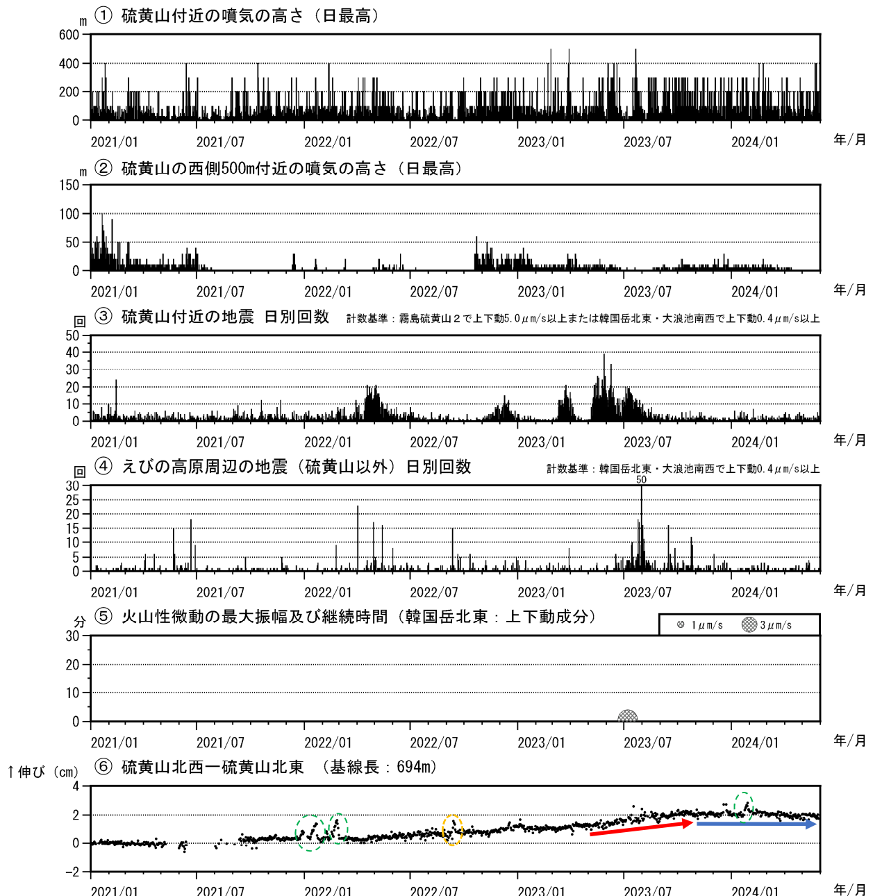
図4 霧島山（えびの高原（硫黄山）周辺） 火山活動経過図（2021年1月～2024年5月）
