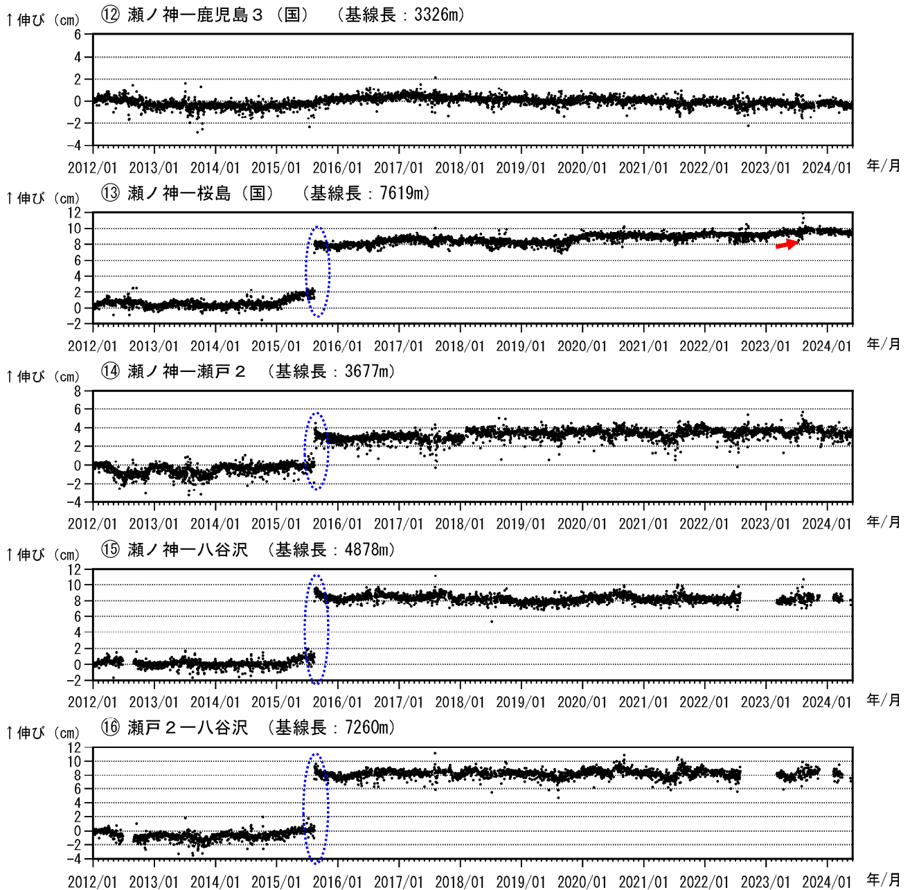
図 7-3 桜島 GNSS 連続観測による基線長変化 (2012 年 1 月～2024 年 5 月)
