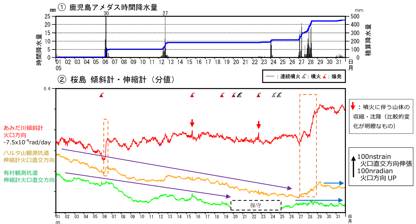
図6 桜島 傾斜計及び伸縮計による地殻変動の状況（2024年5月）
