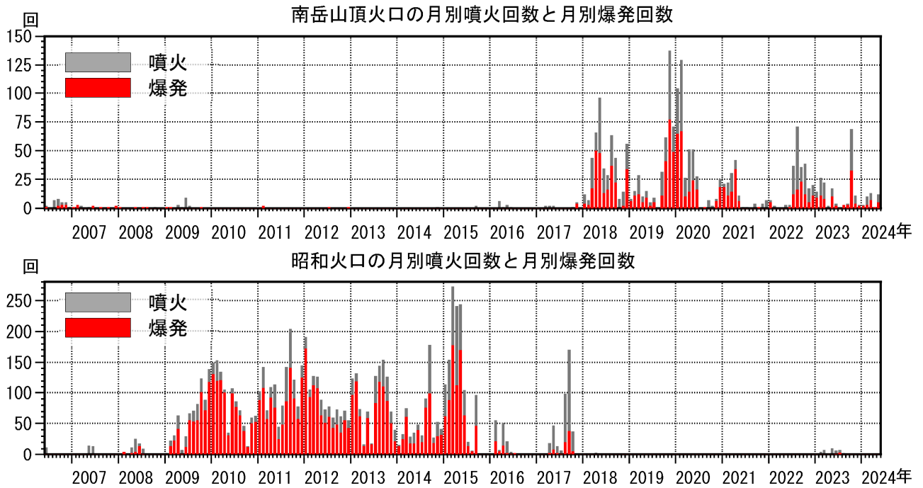
図3 桜島 南岳山頂火口（上図）と昭和火口（下図）の月別噴火回数と月別爆発回数 （2006年6月～2024年5月）
