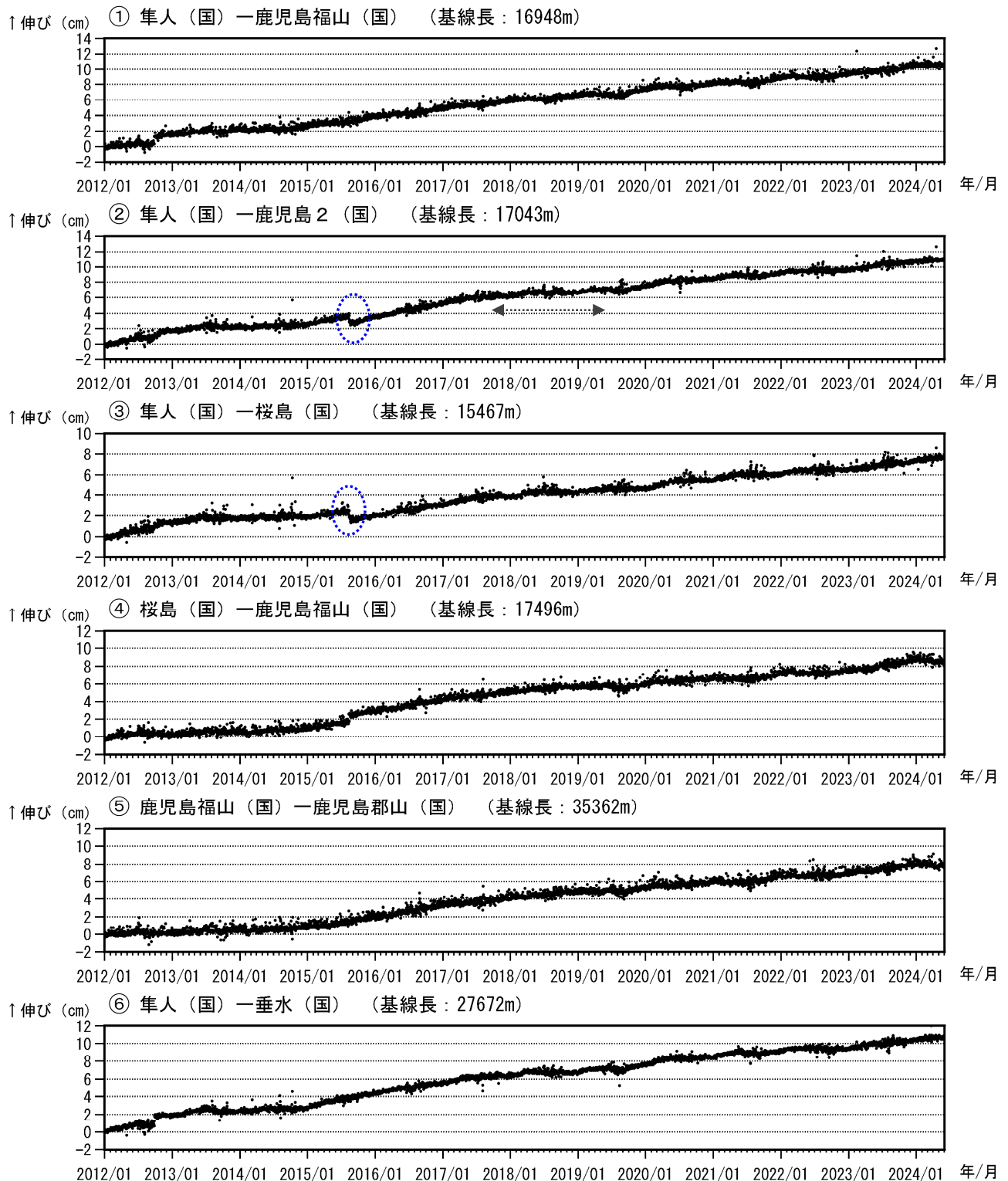
図 7-1 桜島 GNSS 連続観測による基線長変化 (2012 年 1 月～2024 年 5 月)
