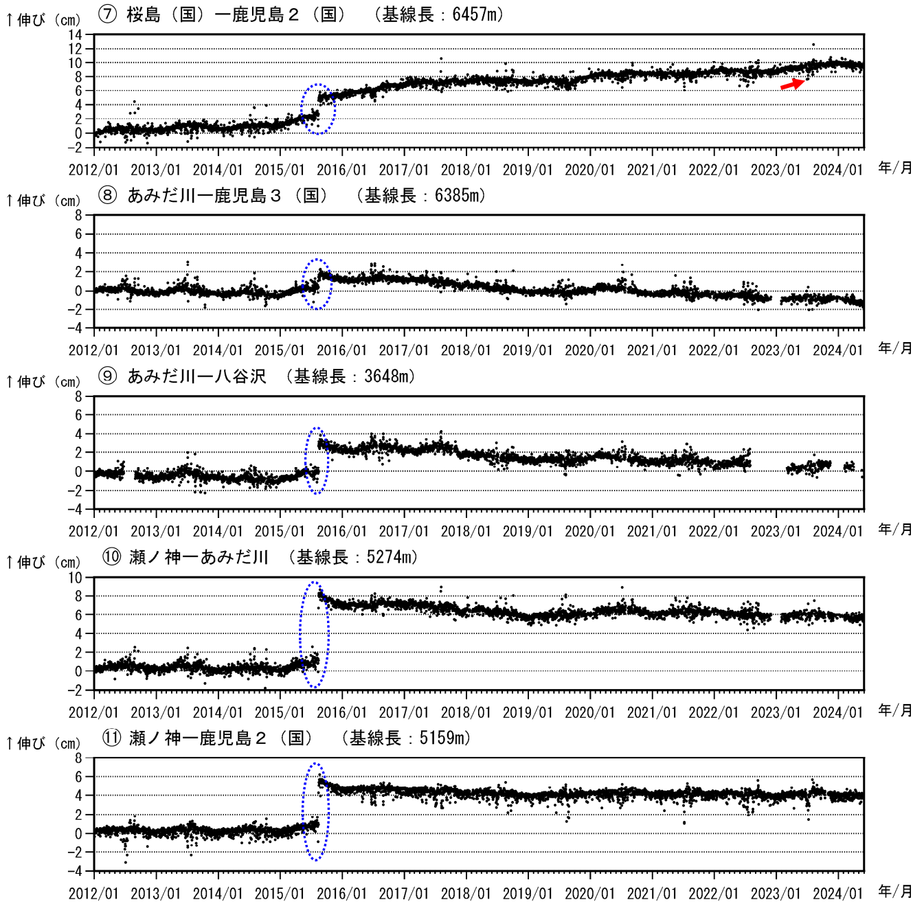
図 7-2 桜島 GNSS 連続観測による基線長変化（2012 年 1 月～2024 年 5 月）
