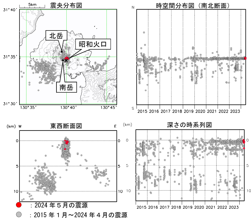
図 2-2 桜島 桜島付近の震源分布図（2015 年 1 月～2024 年 5 月）
