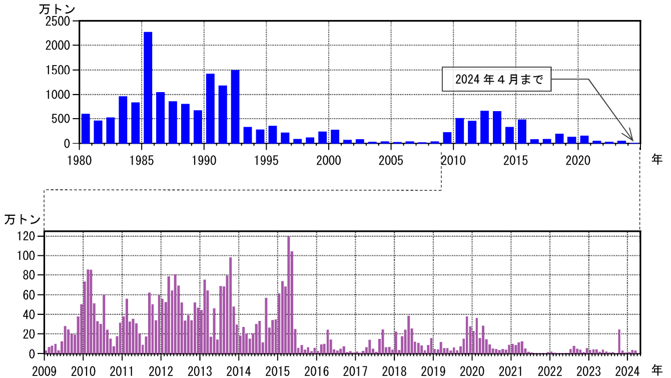
図4 桜島 鹿児島県が実施している降灰の観測データから推定した火山灰の総噴出量 （上段：1980年1月～2024年4月の年別値、下段：2009年1月～2024年4月の月別値）
