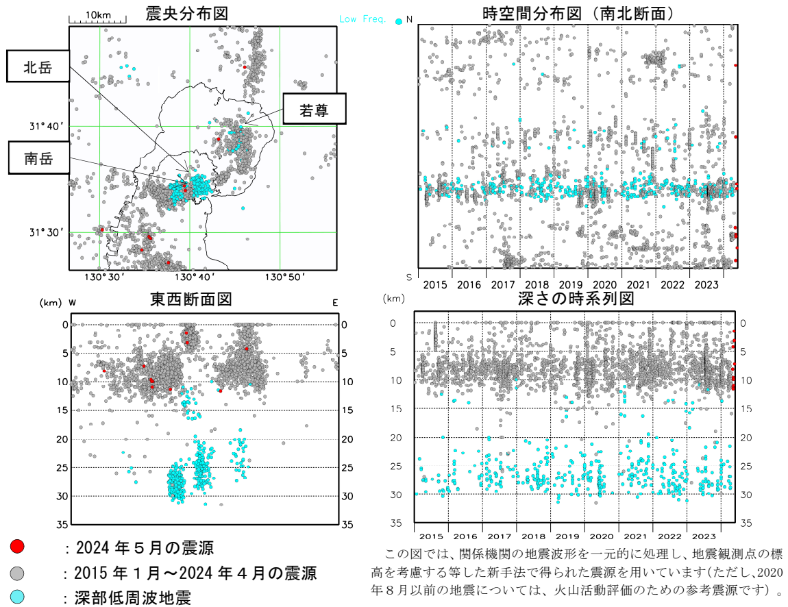
図 2-1 桜島 始良カルデラ周辺の震源分布図（2015 年 1 月～2024 年 5 月）
