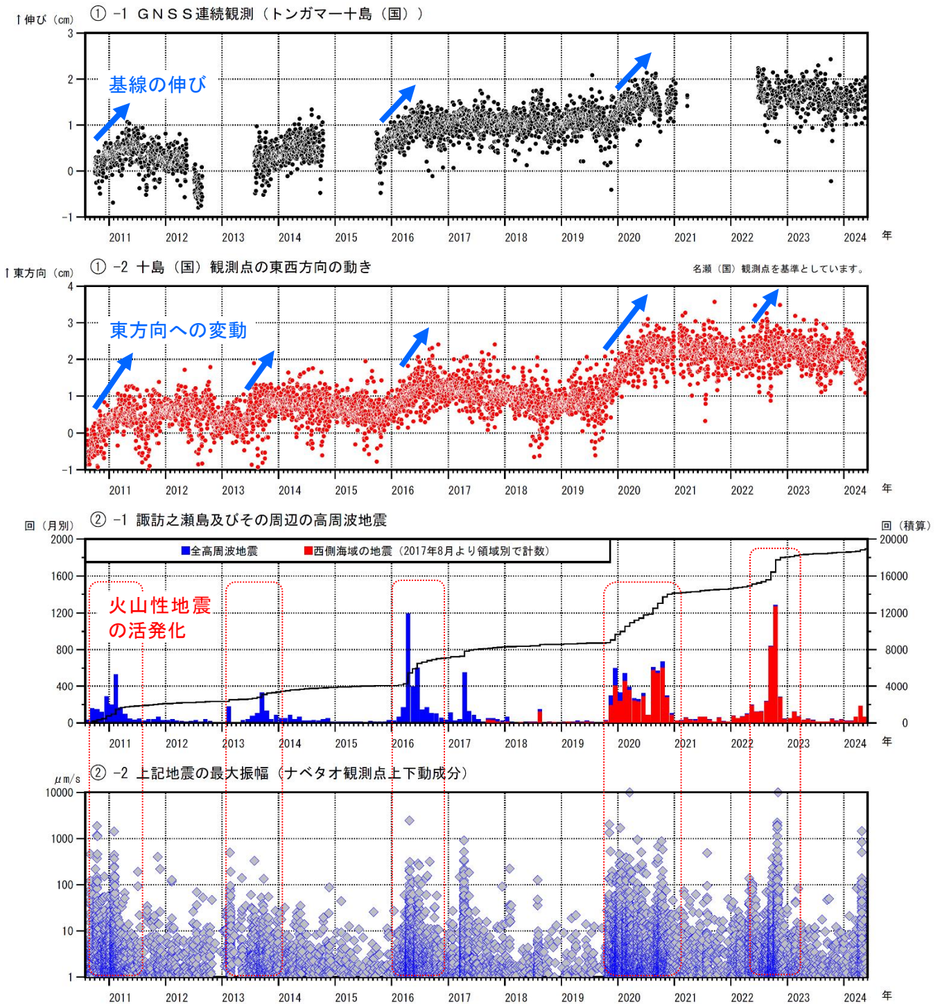
図6 諏訪之瀬島 GNSS連続観測と周辺の火山性地震（2010年8月～2024年5月）
