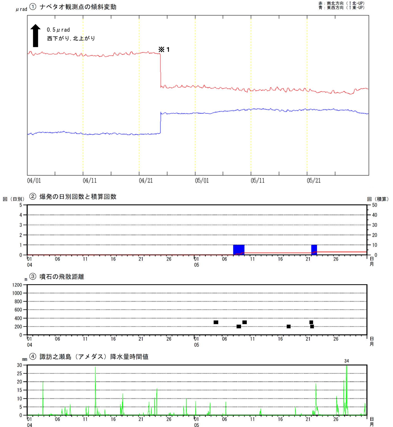
図5 諏訪之瀬島 ナベタオ観測点の傾斜変動と噴火活動（2024年4月～2024年5月）
