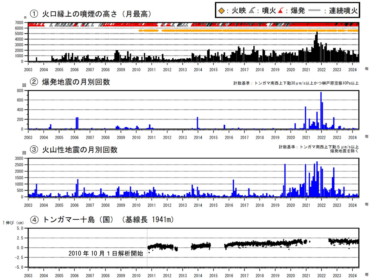
図2 諏訪之瀬島 長期の火山活動経過図（2003年1月～2024年5月）
