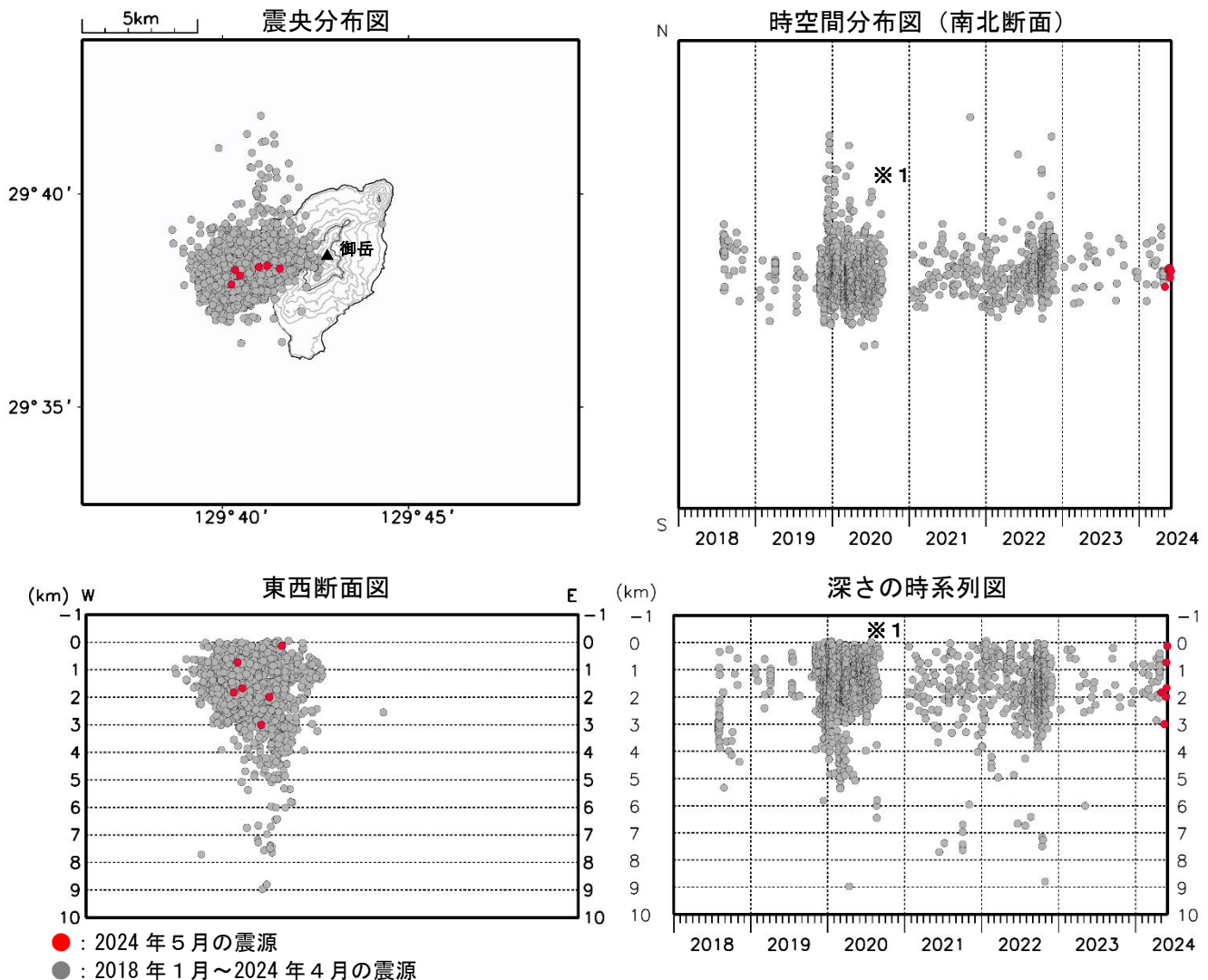
図4 諏訪之瀬島 震源分布図（2018年1月～2024年5月）
