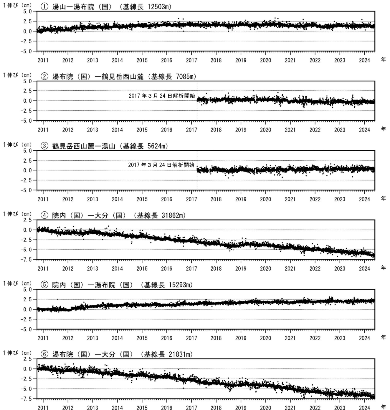
図4 鶴見岳・伽藍岳 GNSS連続観測による基線長変化（2010年10月～2024年5月）
