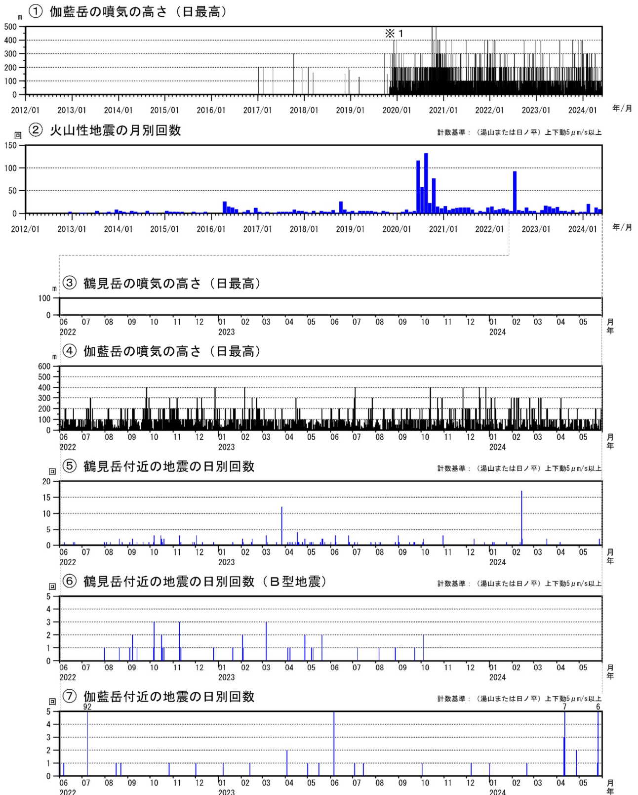
図2 鶴見岳・伽藍岳 火山活動経過図（2012年1月～2024年5月）
