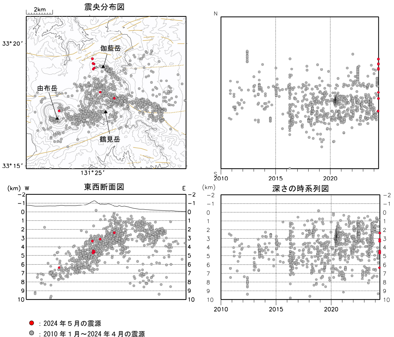
図3 鶴見岳・伽藍岳 震源分布図（2010年1月～2024年5月）
