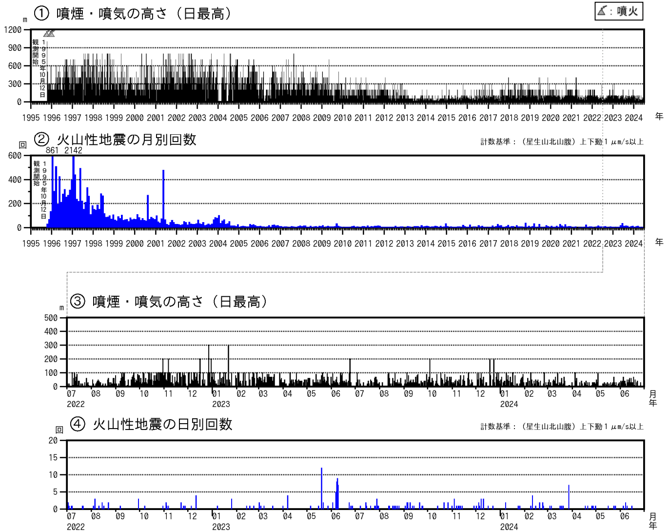
図2 九重山 火山活動経過図（1995年1月～2024年6月）
