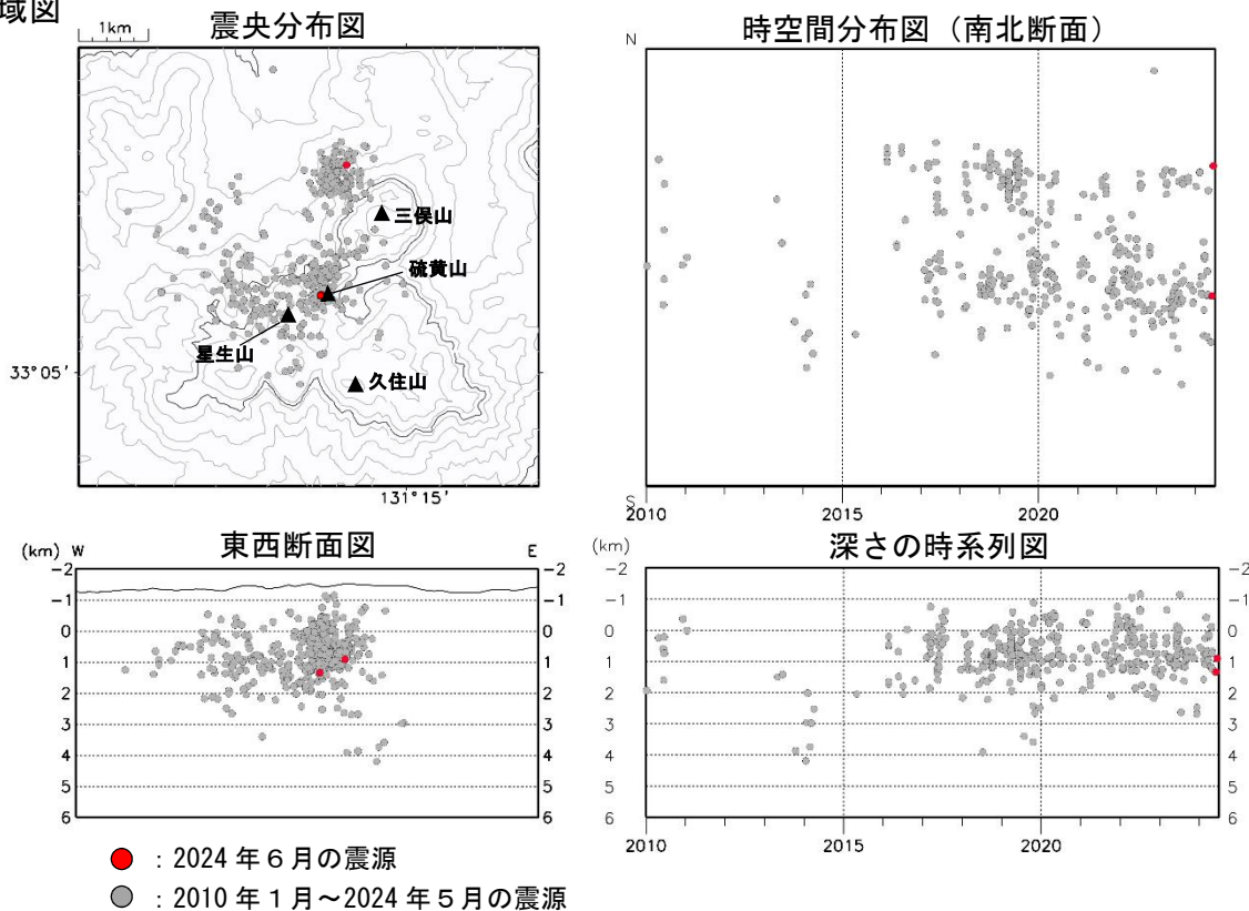
図3 九重山 震源分布図 ①広域図 ②狭域図（2010年1月～2024年6月）
