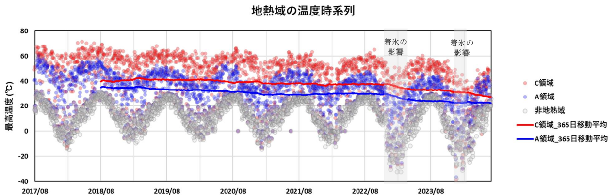
図 1-2 九重山 星生山北尾根の赤外熱映像装置による日別最高温度（2017年8月～2024年6月）
