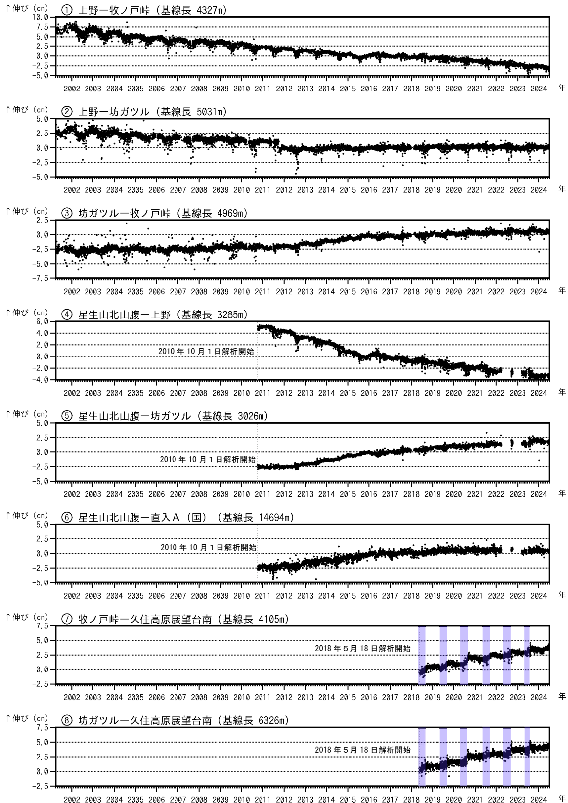
図5 九重山 GNSS 連続観測による基線長変化（2001年4月～2024年6月）
