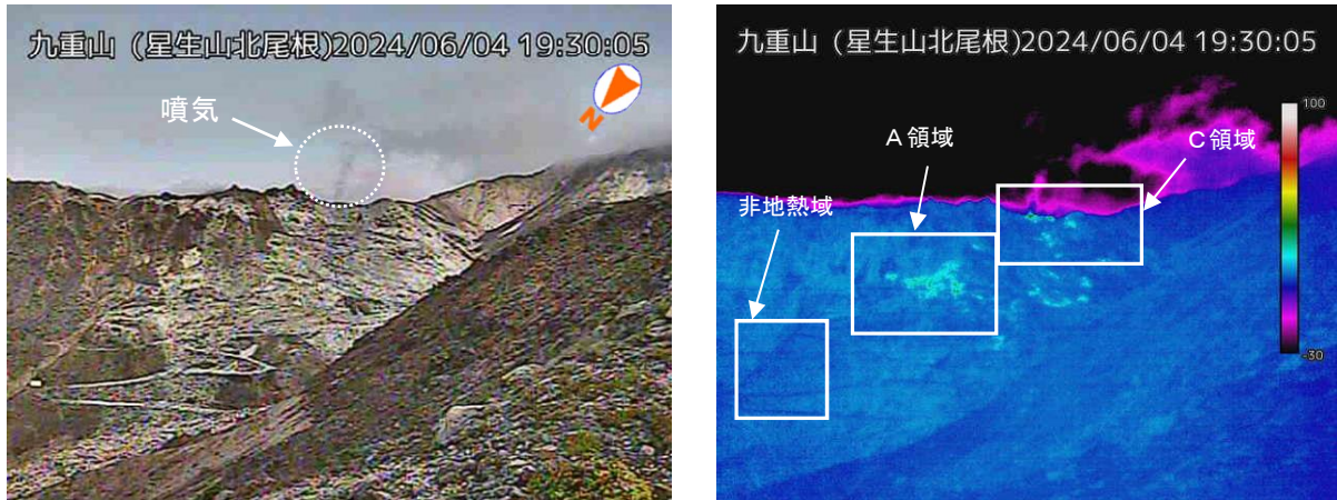
図 1-1 九重山 硫黄山の噴気及び地熱域の状況（6月4日 星生山北尾根監視カメラ）
