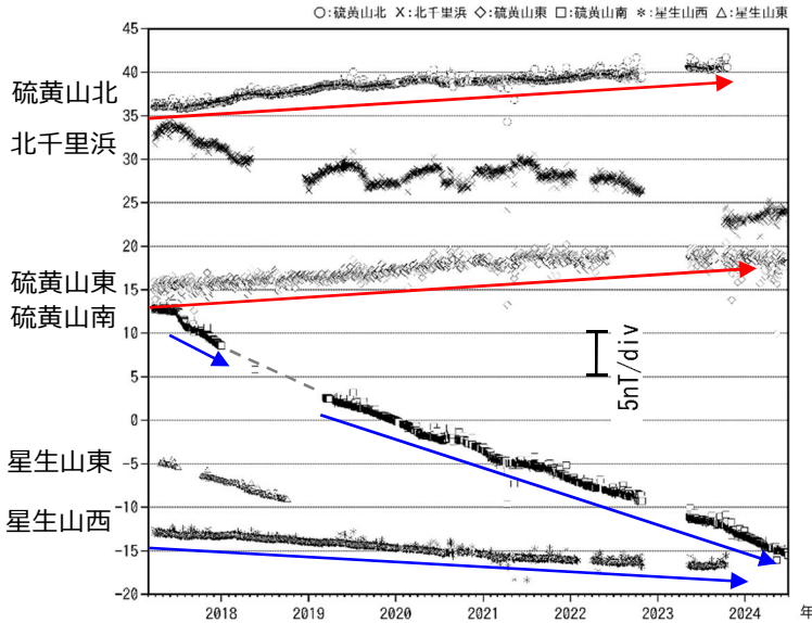
図 4-1 九重山 連続観測による全磁力の変化 (2017年3月～2024年6月)
