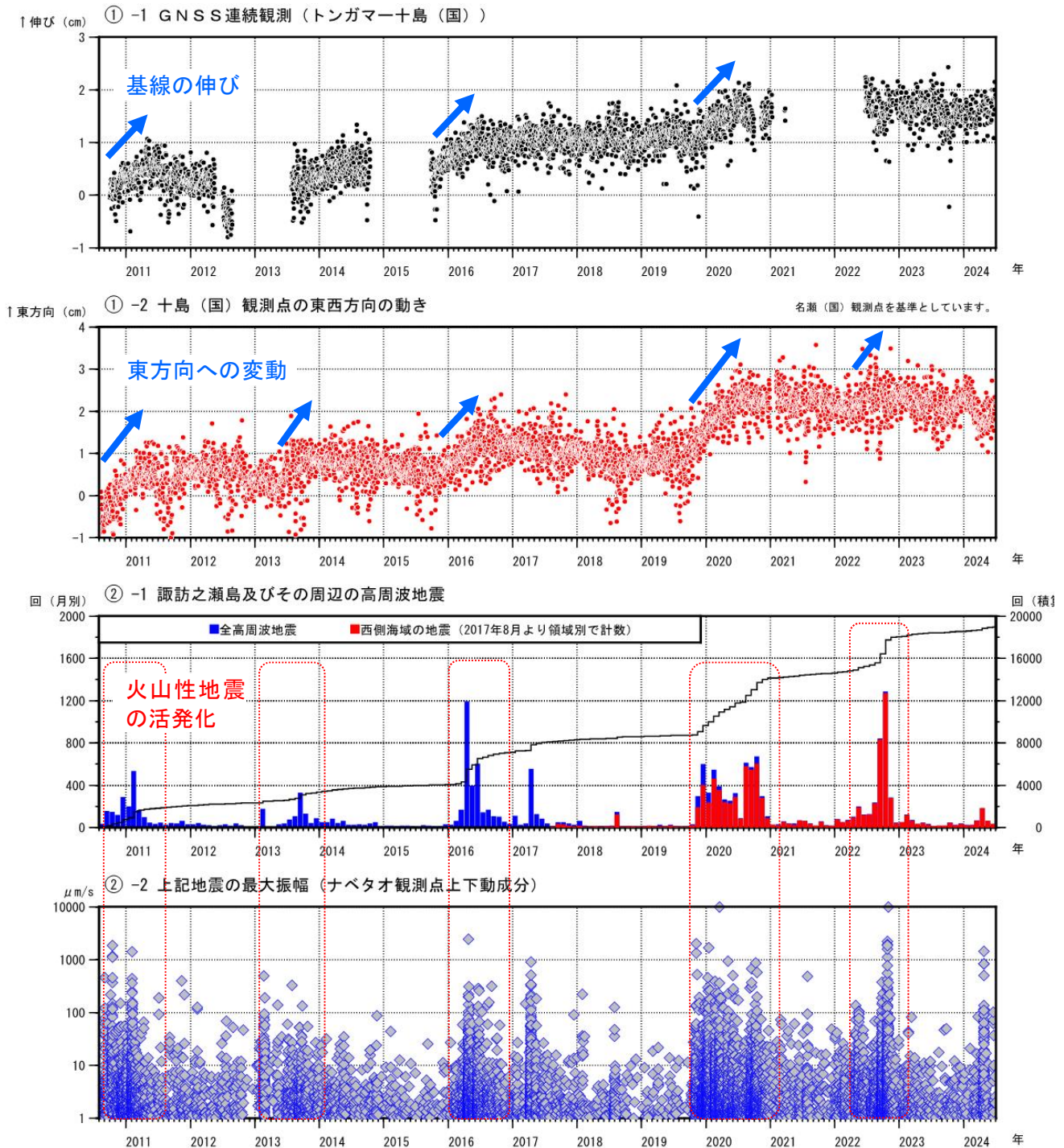
図6 諏訪之瀬島 GNSS連続観測と周辺の火山性地震（2010年8月～2024年6月）
