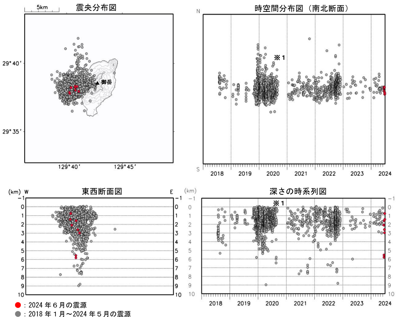
図4 諏訪之瀬島 震源分布図（2018年1月～2024年6月）
