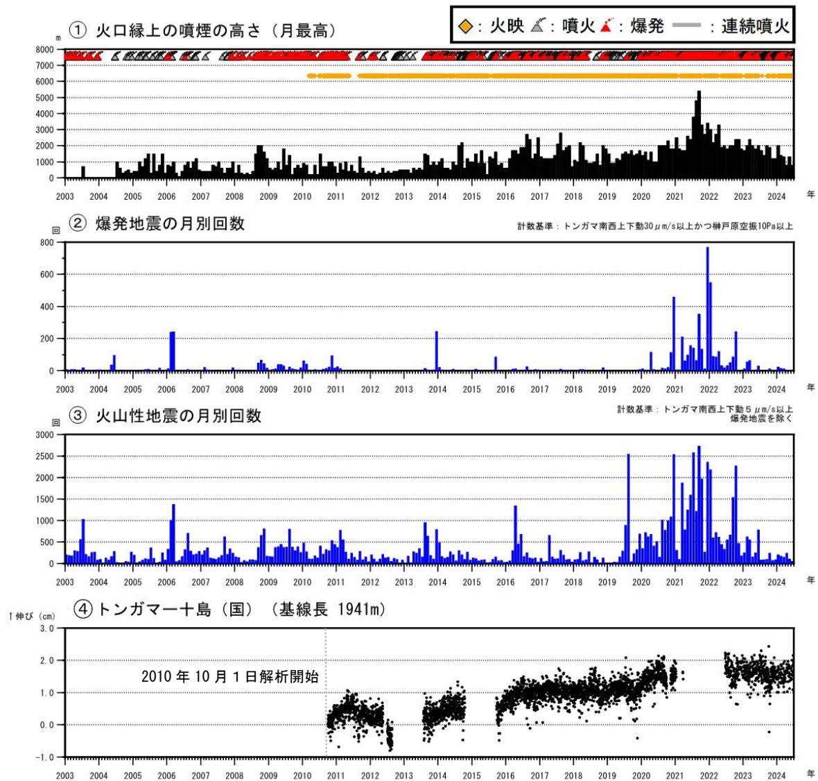
図2 諏訪之瀬島 長期の火山活動経過図（2003年1月～2024年6月）
