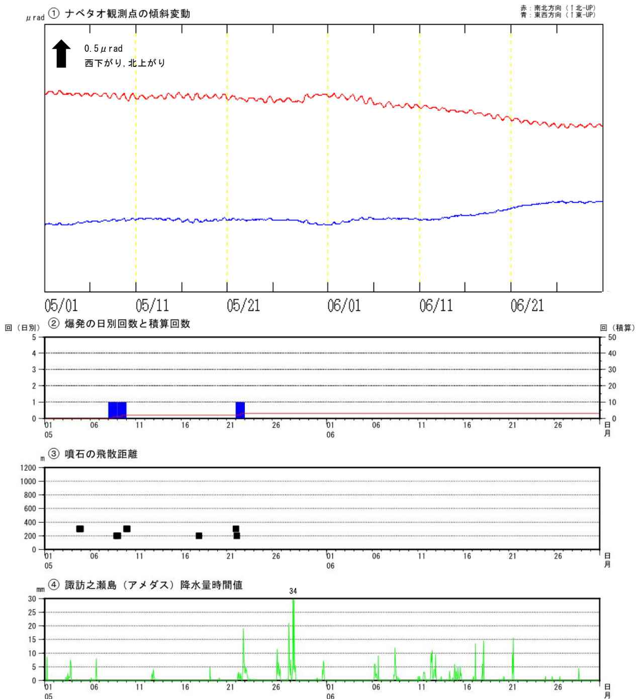
図5 諏訪之瀬島 ナベタオ観測点の傾斜変動と噴火活動（2024年5月～2024年6月）
