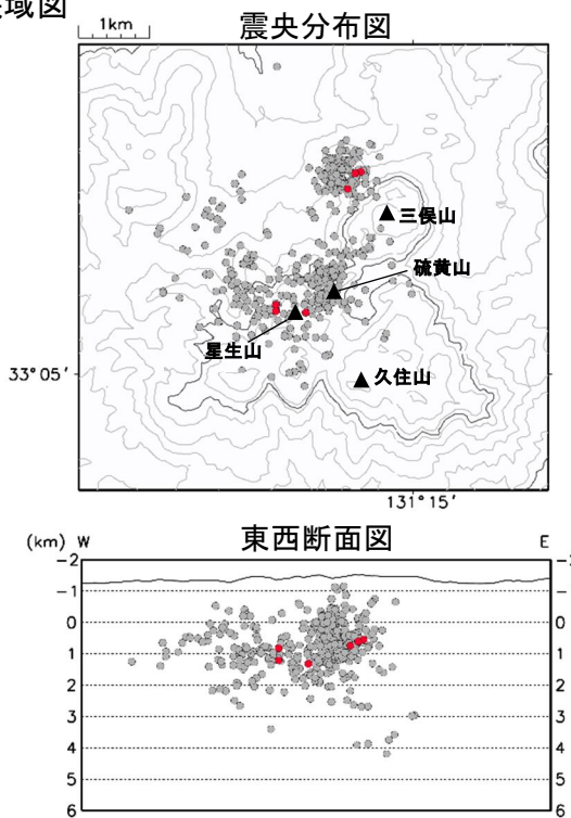
図3 九重山 震源分布図 ①広域図 ②狭域図（2010 年 1 月～2024 年 8 月）
