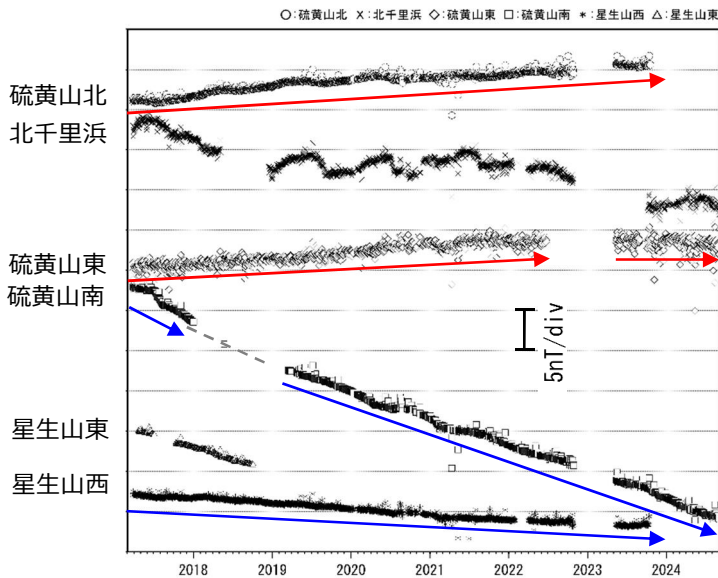
図 4-1 九重山 連続観測による全磁力の変化 (2017年3月～2024年8月)
