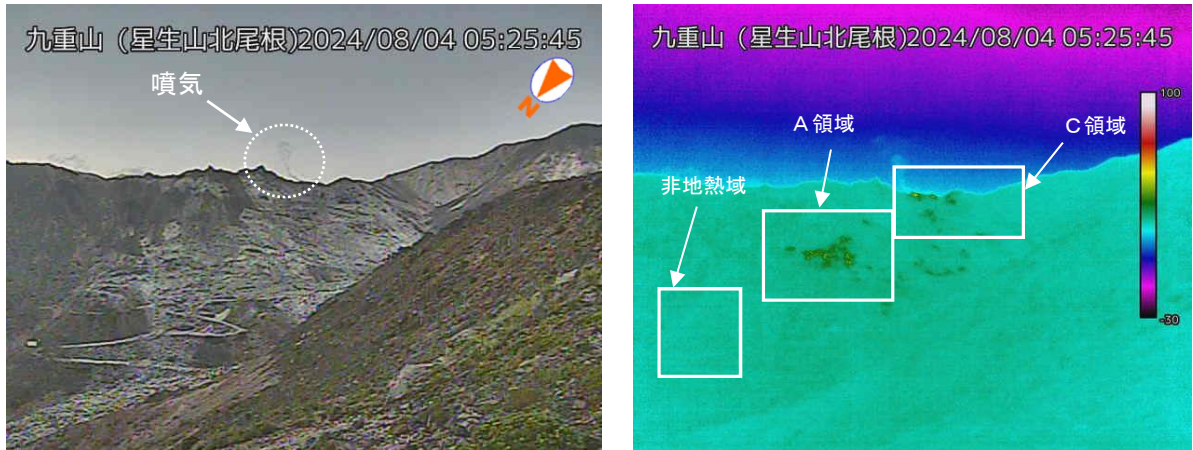
図 1-1 九重山 硫黄山の噴気及び地熱域の状況（8月4日 星生山北尾根監視カメラ）
