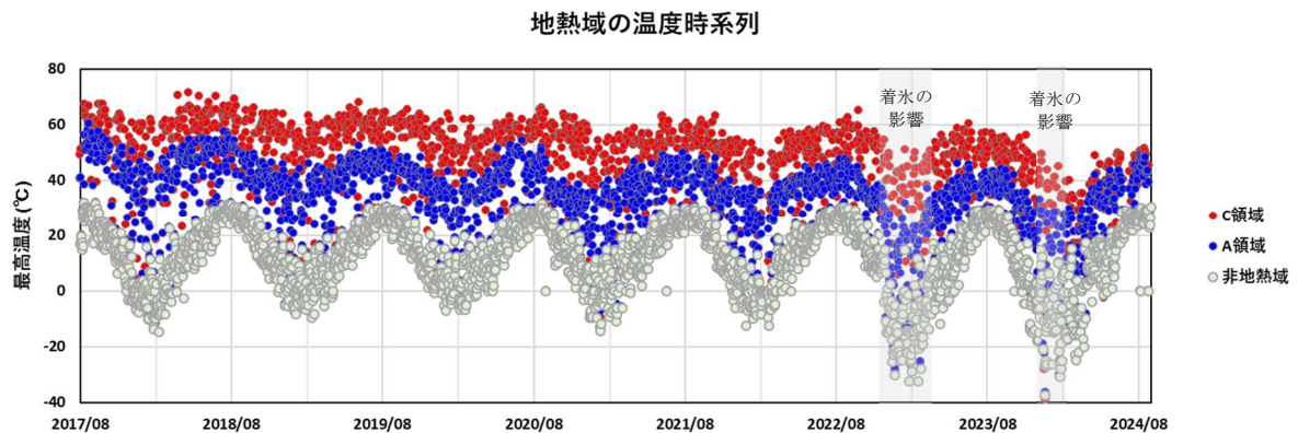
図 1-2 九重山 星生山北尾根の赤外熱映像装置による日別最高温度（2017年8月～2024年8月）
