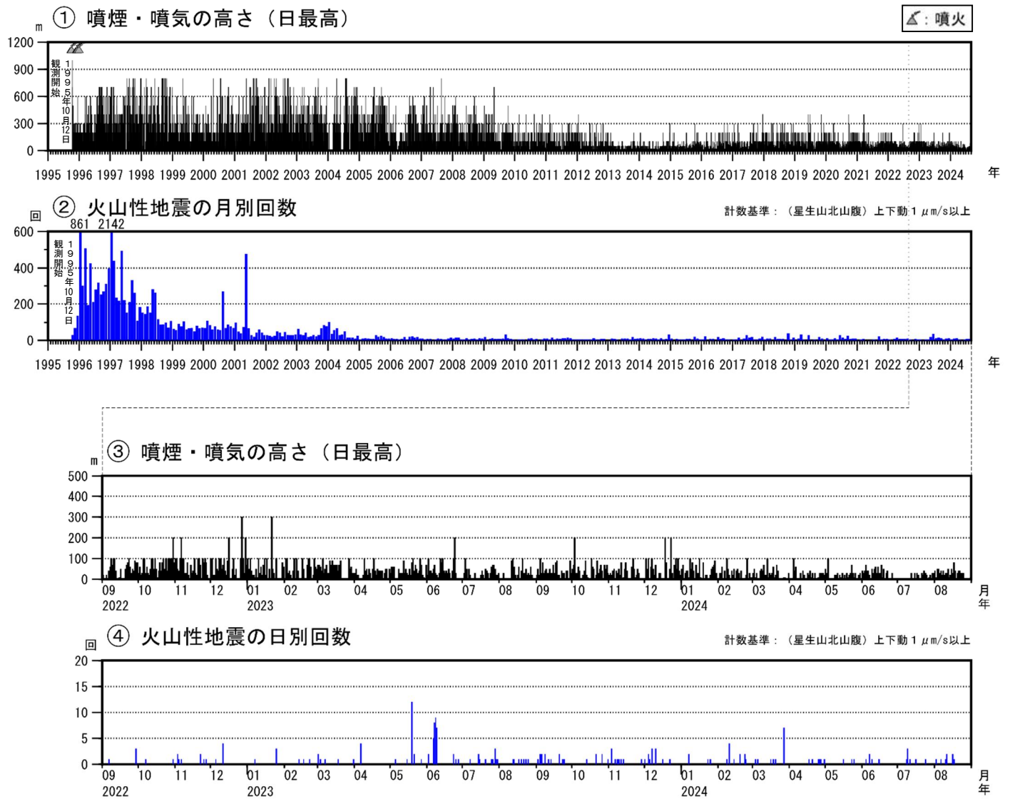
図2 九重山 火山活動経過図（1995年1月～2024年8月）
