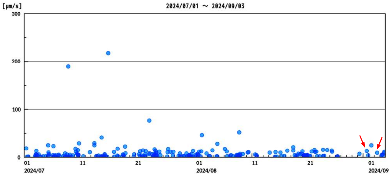
図2 薩摩硫黄島 火山性地震の最大振幅（2024年7月～9月3日、物草観測点 上下動成分）
