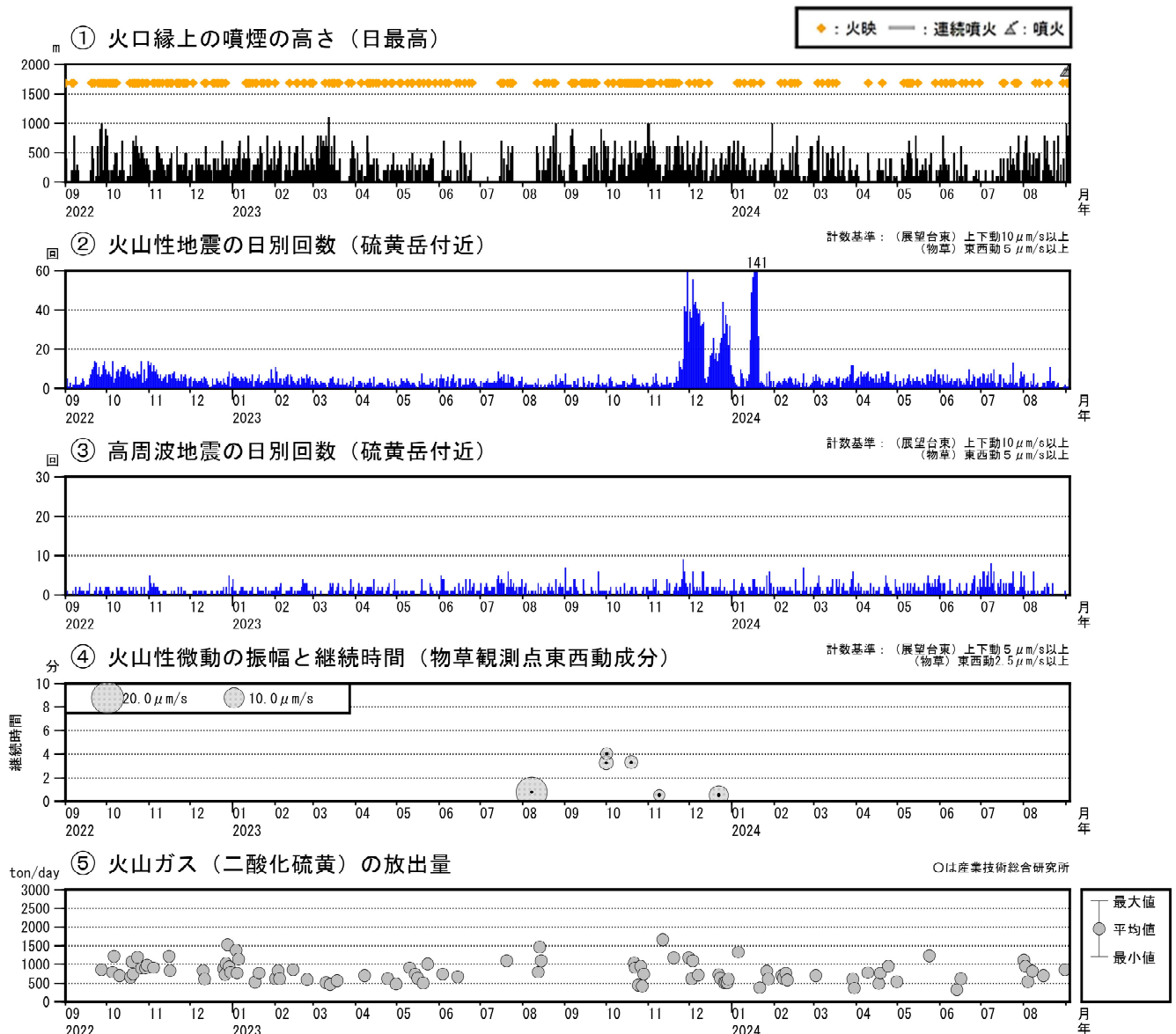
図5 薩摩硫黄島 火山活動経過図（2022年9月～2024年9月3日）
