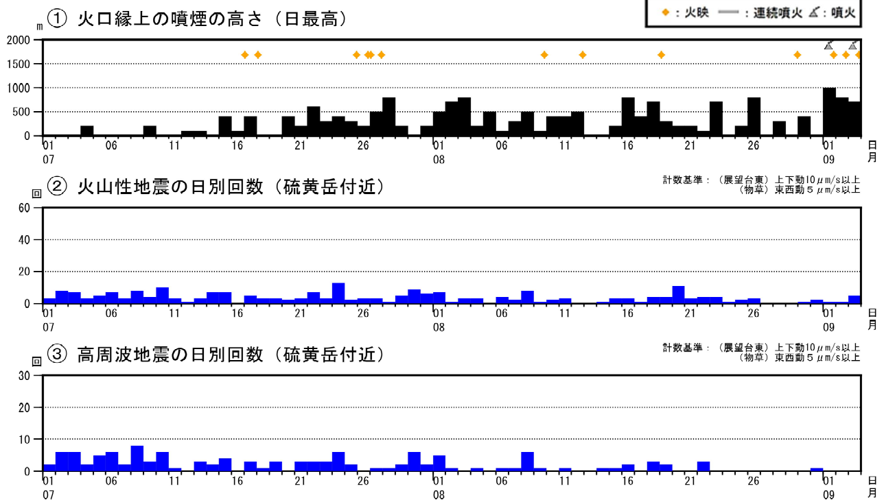
図3 薩摩硫黄島 火山活動経過図（2024年7月～9月3日）
