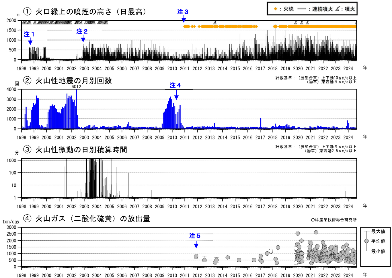
図4 薩摩硫黄島 火山活動経過図（1998年1月～2024年9月3日）
