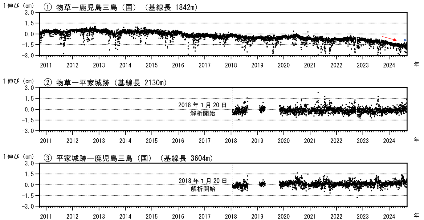
図6 薩摩硫黄島 GNSS連続観測による基線長変化（2010年10月～2024年9月3日）
