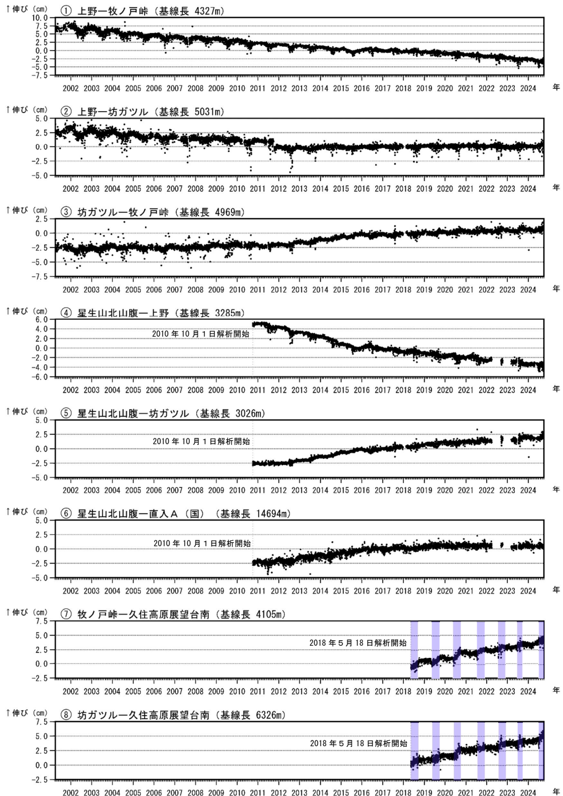
図5 九重山 GNSS 連続観測による基線長変化（2001年4月～2024年9月）
