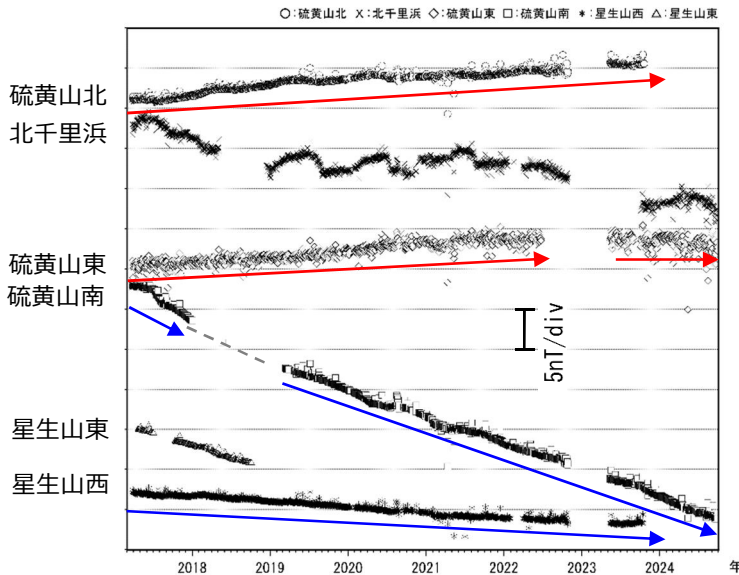
図 4-1 九重山 連続観測による全磁力の変化 (2017年3月～2024年9月)
