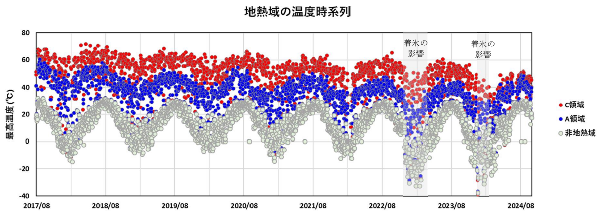
図 1-2 九重山 星生山北尾根の赤外熱映像装置による日別最高温度（2017年8月～2024年9月）
