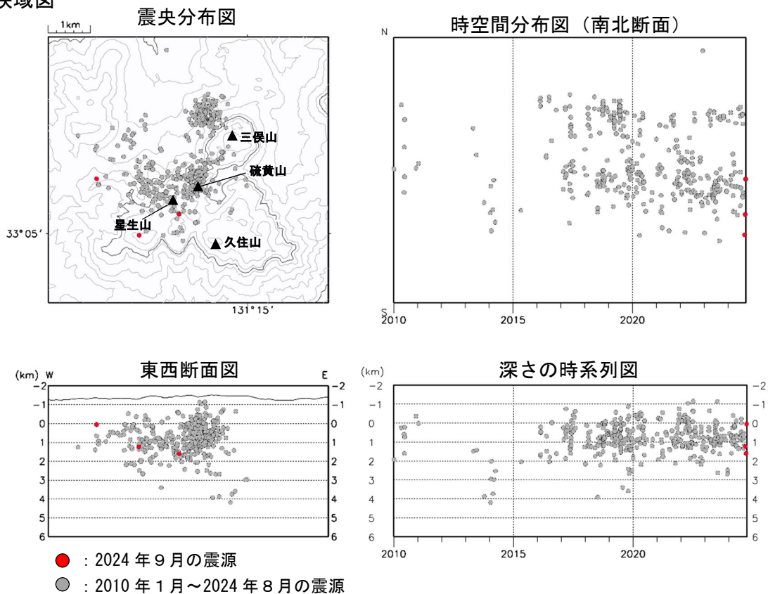
図3 九重山 震源分布図 ①広域図 ②狭域図（2010年1月～2024年9月）
