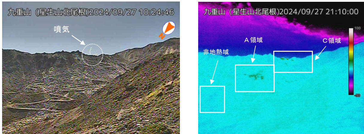
図 1-1 九重山 硫黄山の噴気及び地熱域の状況（9月27日 星生山北尾根監視カメラ）
