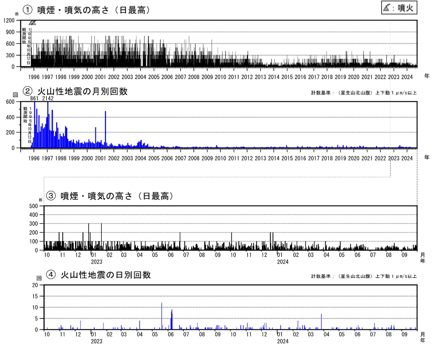
図2 九重山 火山活動経過図（1995年1月～2024年9月）
