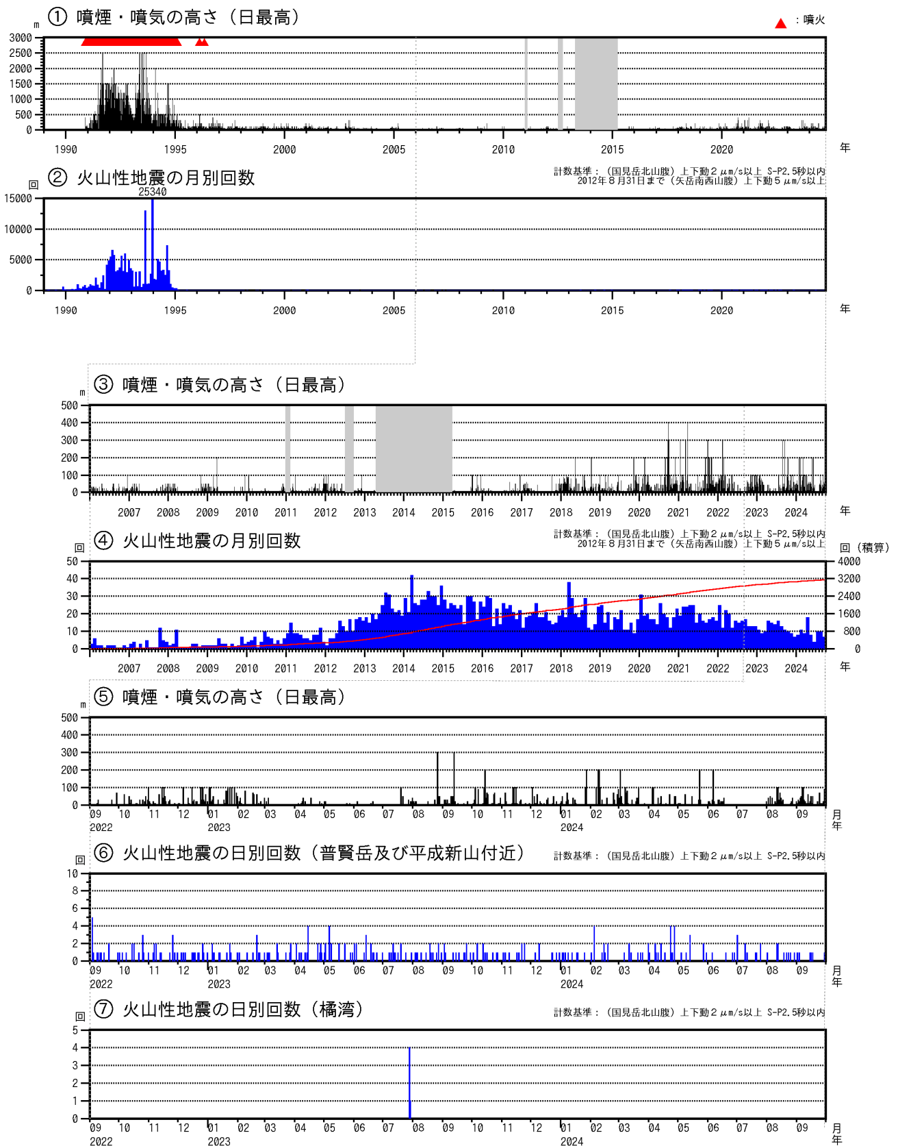
図2 雲仙岳 火山活動経過図（1989年1月～2024年9月）
