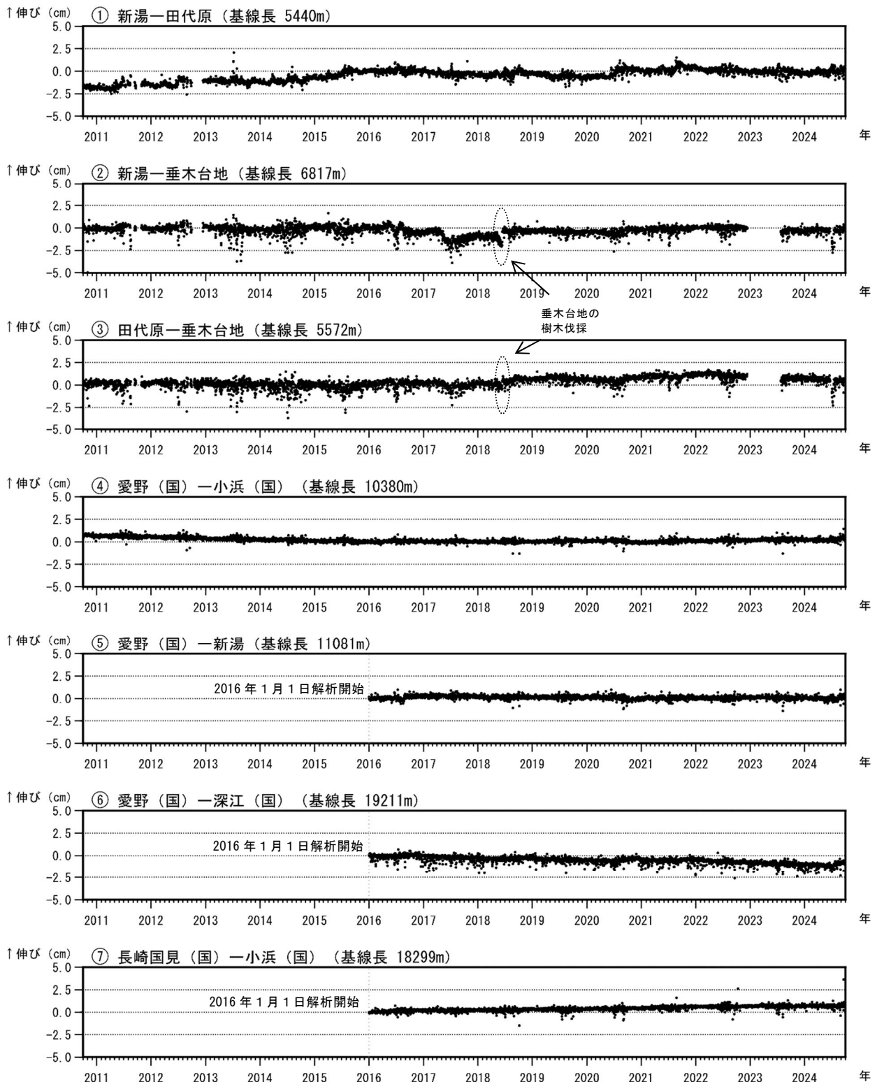
図4 雲仙岳 GNSS連続観測による基線長変化（2010年10月～2024年9月）
