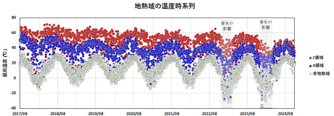
図 1-2 九重山 星生山北尾根の赤外熱映像装置による日別最高温度（2017年8月～2024年10月）
