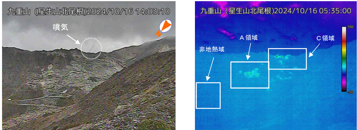
図 1-1 九重山 硫黄山の噴気及び地熱域の状況（10月16日 星生山北尾根監視カメラ）
