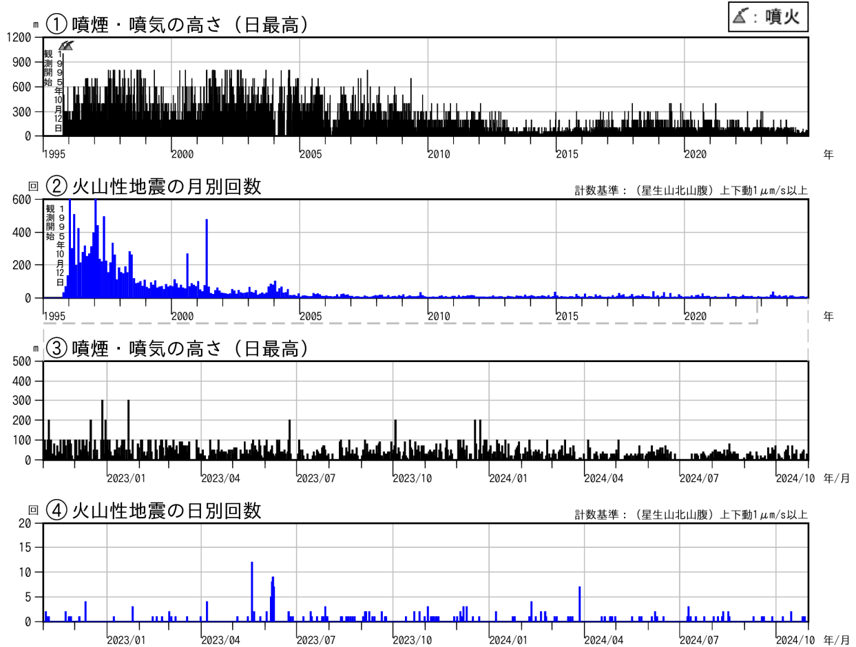
図2 九重山 火山活動経過図（1995年1月～2024年10月）
