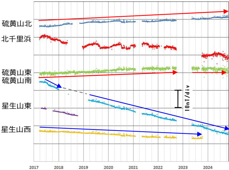
図 4-1 九重山 連続観測による全磁力の変化 (2017年3月～2024年10月)
