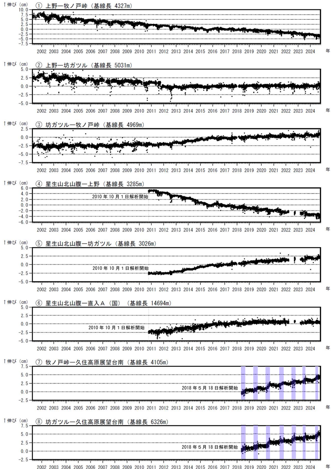
図5 九重山 GNSS 連続観測による基線長変化（2001年4月～2024年10月）
