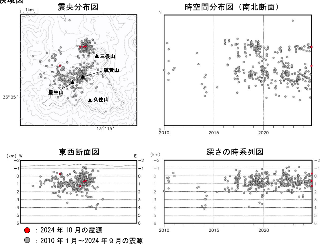
図3 九重山 震源分布図 ①広域図 ②狭域図（2010年1月～2024年10月）
