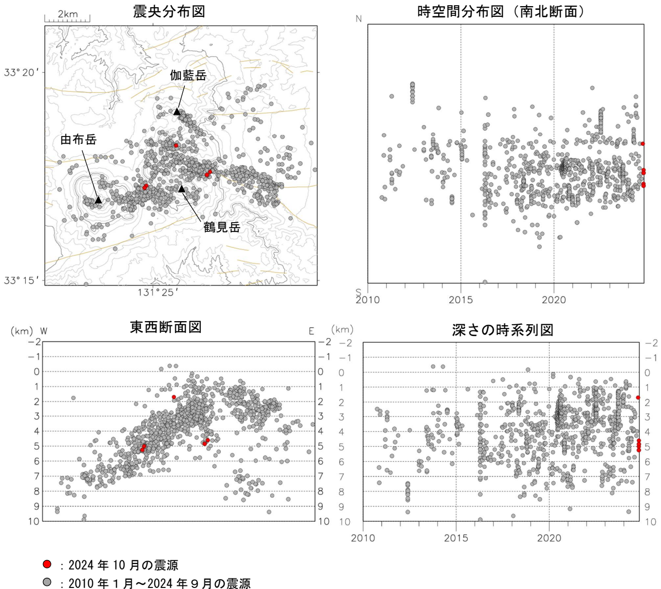
図3 鶴見岳・伽藍岳 震源分布図（2010年1月～2024年10月）
