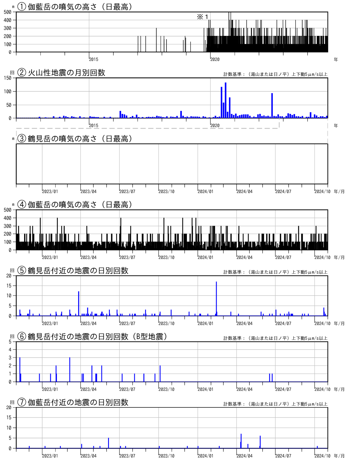
図2 鶴見岳・伽藍岳 火山活動経過図（2012年1月～2024年10月）
