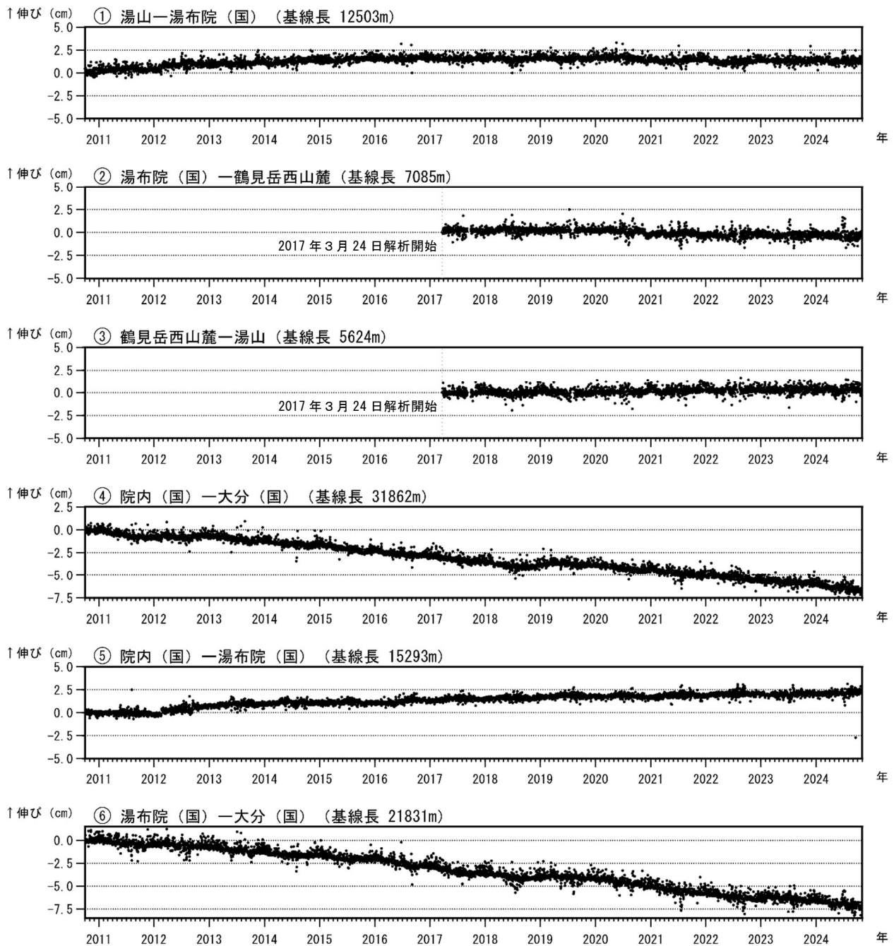
図4 鶴見岳・伽藍岳 GNSS連続観測による基線長変化（2010年10月～2024年10月）
