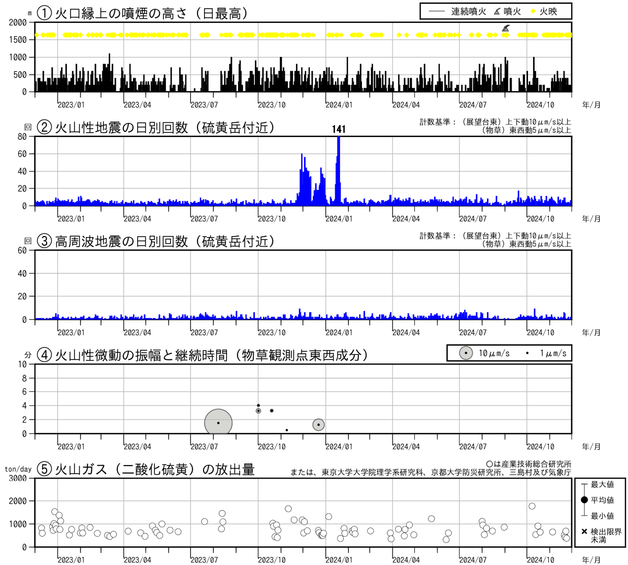
図3 薩摩硫黄島 火山活動経過図（2022年12月～2024年11月）
