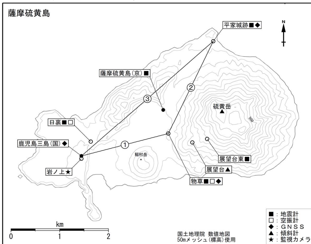
図5 薩摩硫黄島 観測点配置図とGNSS連続観測の基線番号
