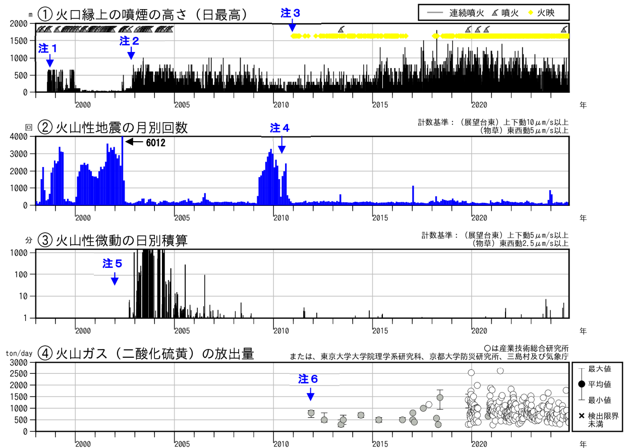
図2 薩摩硫黄島 火山活動経過図（1998年1月～2024年11月）
