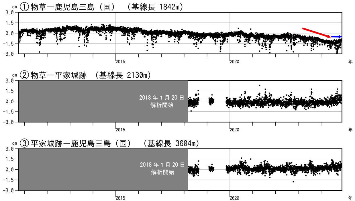
図4 薩摩硫黄島 GNSS連続観測による基線長変化（2010年10月～2024年11月）
