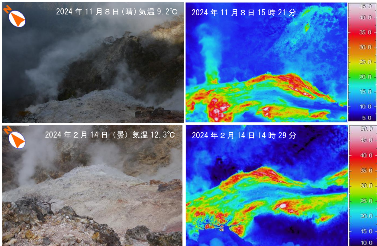
図 2-1 鶴見岳・伽藍岳 鶴見岳地獄谷赤池噴気孔の状況と地表面温度分布（鶴見岳地獄谷赤池噴気孔にて撮影）
