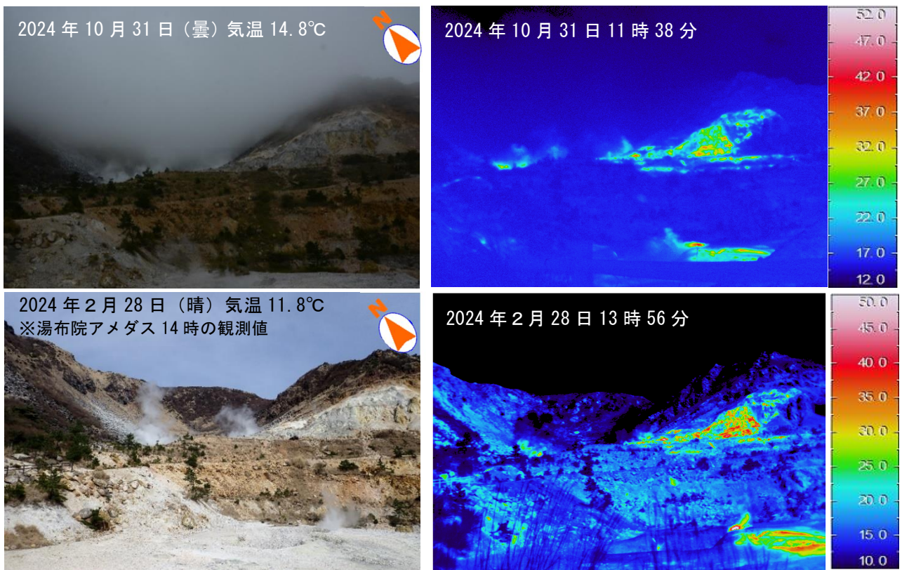
図 2-2 鶴見岳・伽藍岳 伽藍岳A群噴気地帯の状況と地表面温度分布（泥火山西観測点より撮影）
