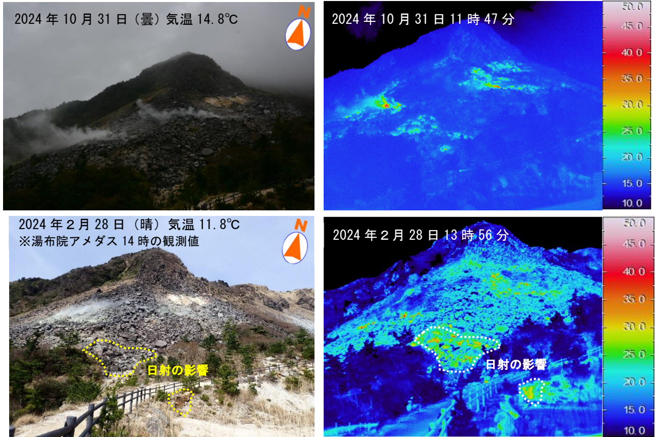
図 2-3 鶴見岳・伽藍岳 伽藍岳B群噴気地帯の状況と地表面温度分布（泥火山西観測点より撮影） 2024 年 2 月 28 日に実施した観測と比較して、噴気の状況及び、地熱域の分布や温度に特段の 変化は認められませんでした。
