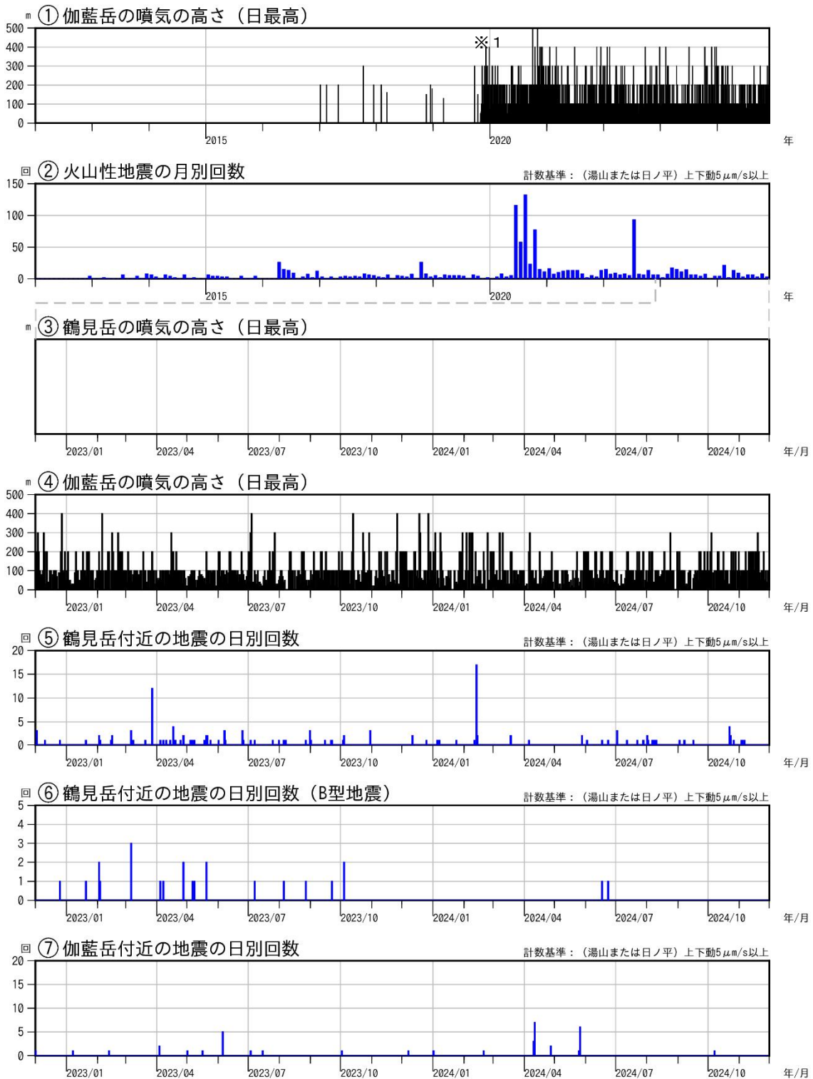
図3 鶴見岳・伽藍岳 火山活動経過図（2012年1月～2024年11月）
