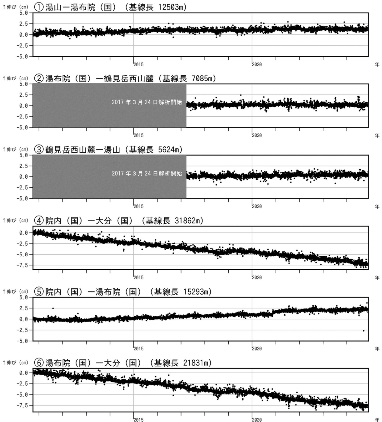
図5 鶴見岳・伽藍岳 GNSS連続観測による基線長変化（2010年10月～2024年11月）
