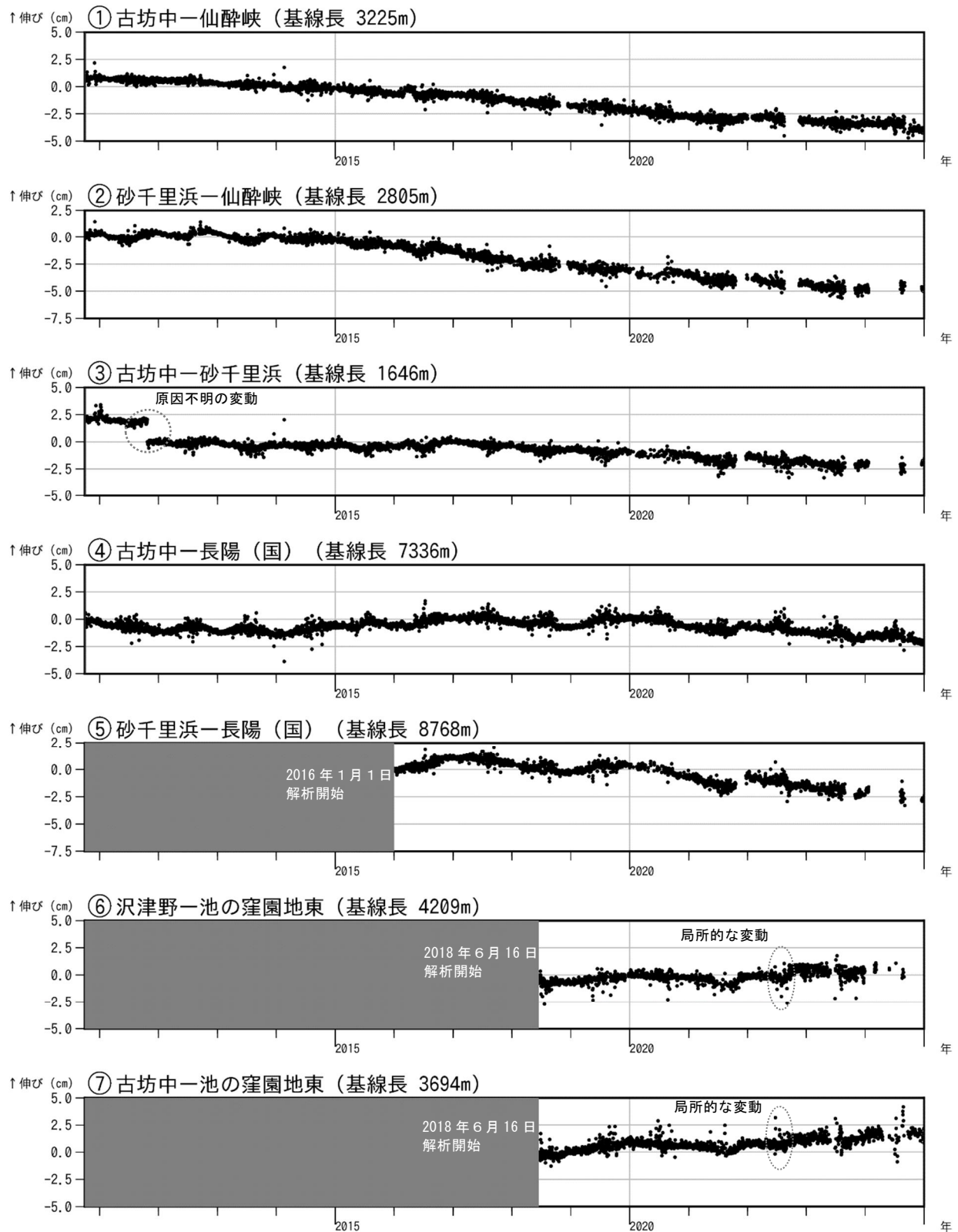
図5 阿蘇山 GNSS 連続観測による基線長変化（2010年11月～2024年12月）
